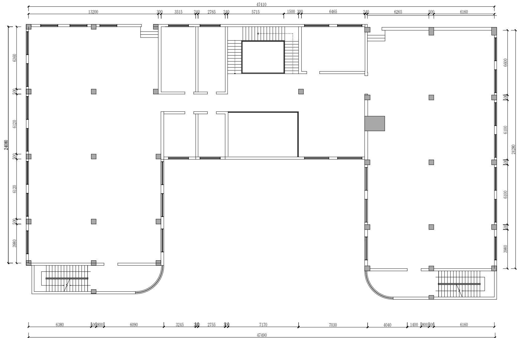
原始结构图
