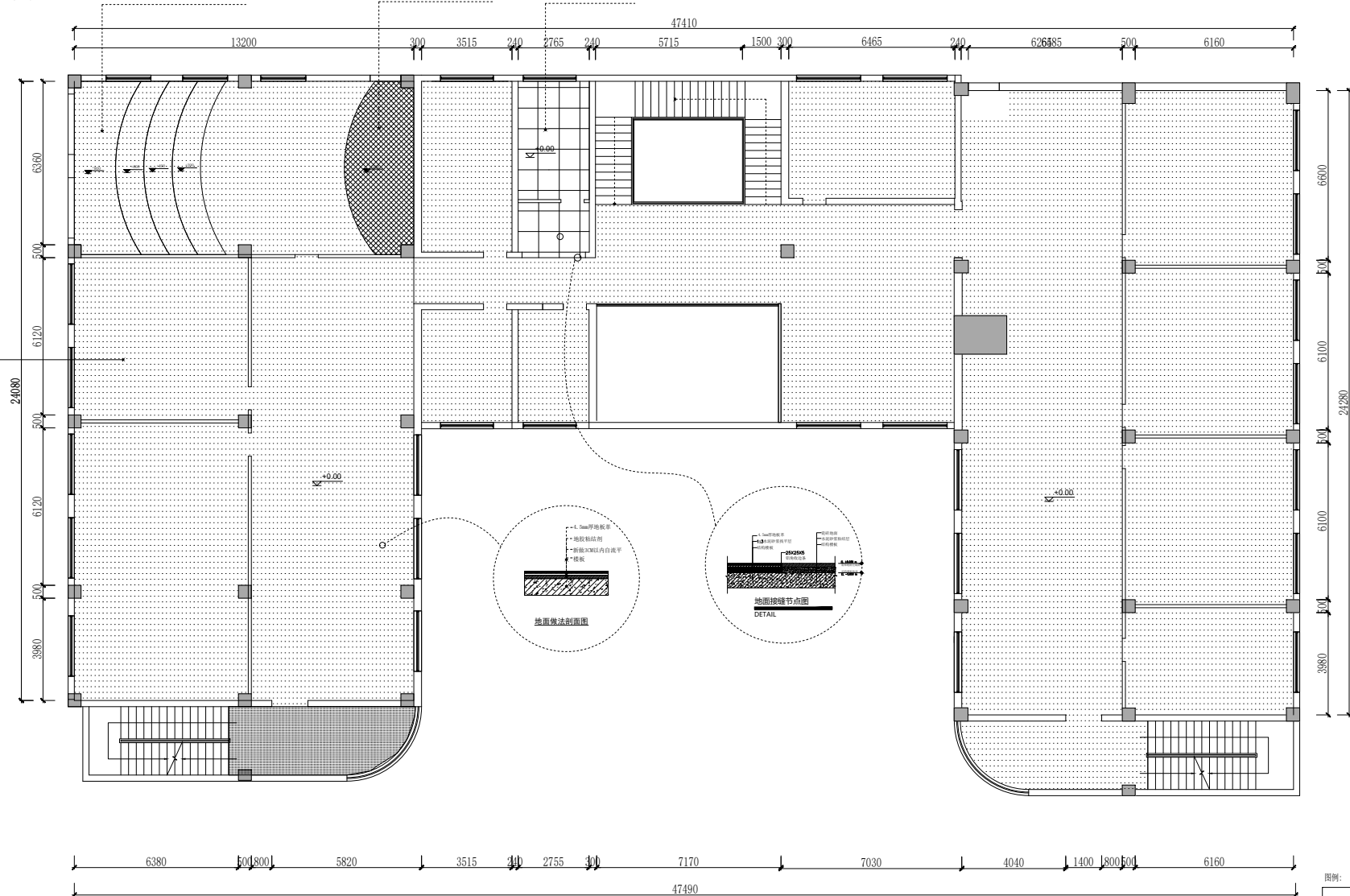
地面铺装图
