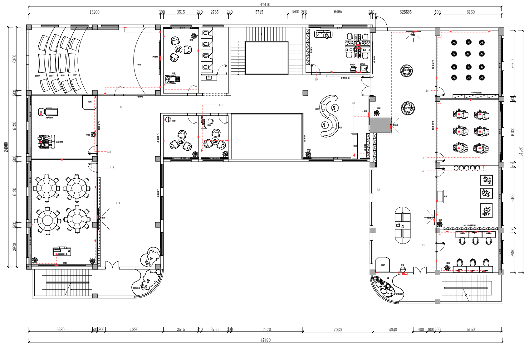
强电连线图
