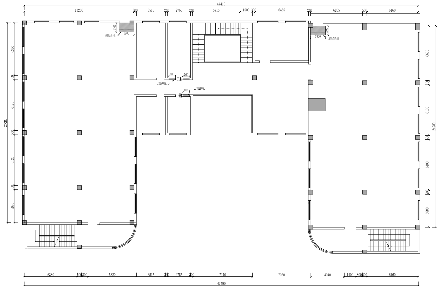
拆墙图
