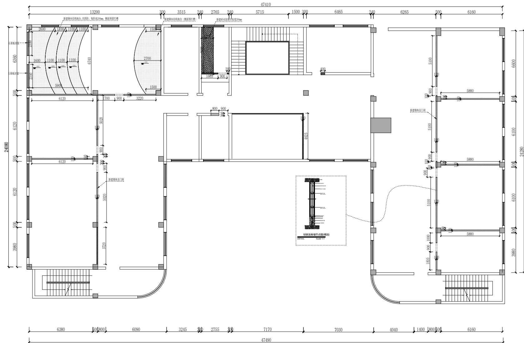
砌墙图
