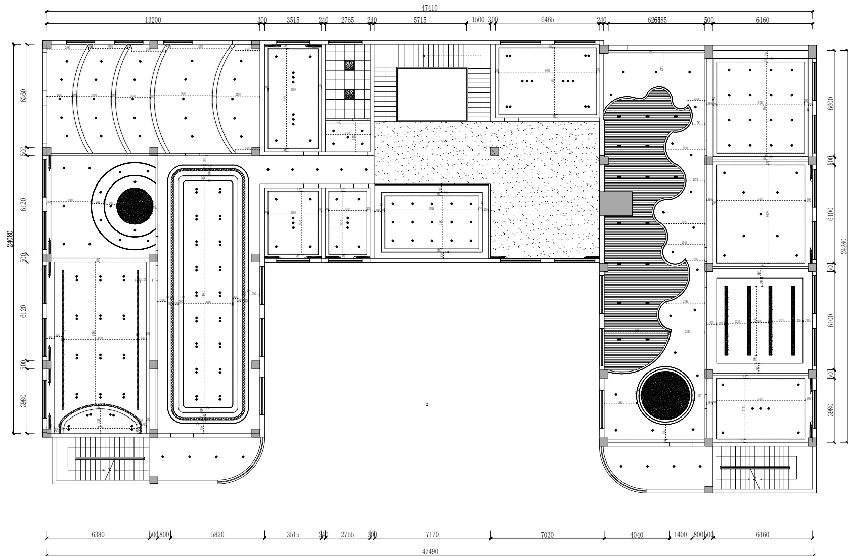
天花尺寸图
