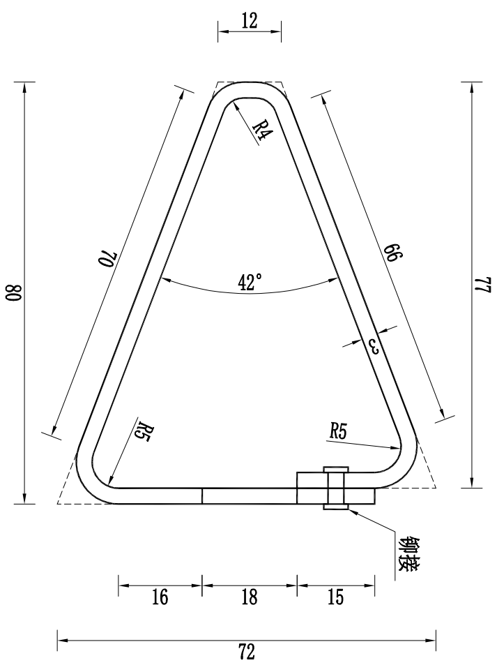
轮廓标俯视图 1:1
