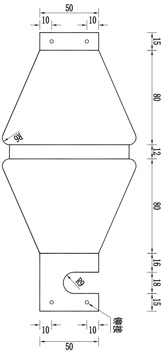
轮廓展开图 1:2
