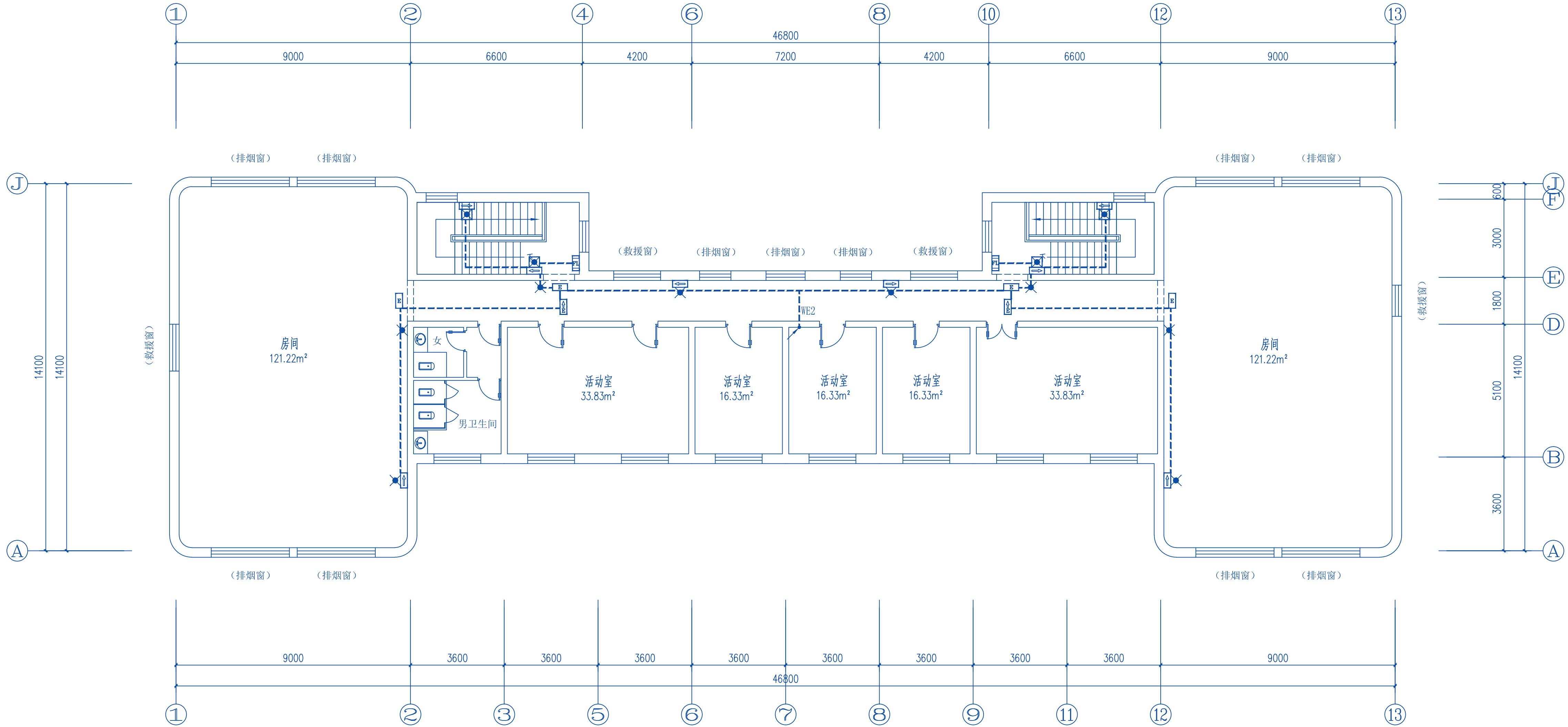
二层改造应急照明平面图 1:100
