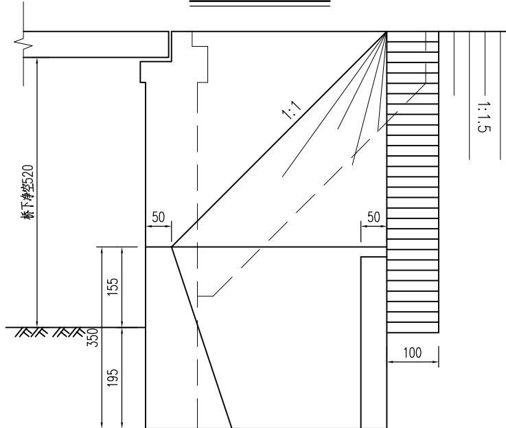
锥坡立面布置图
