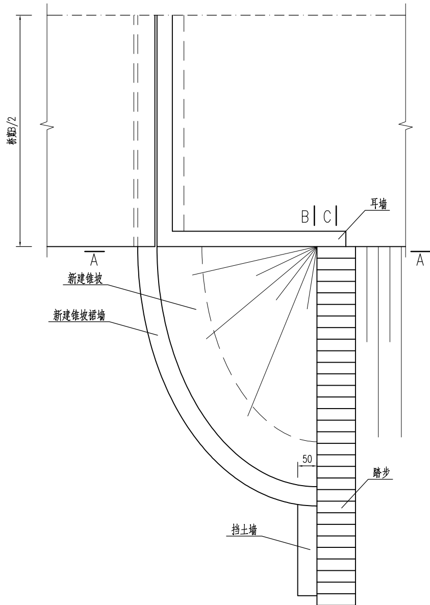
锥坡立面布置图
