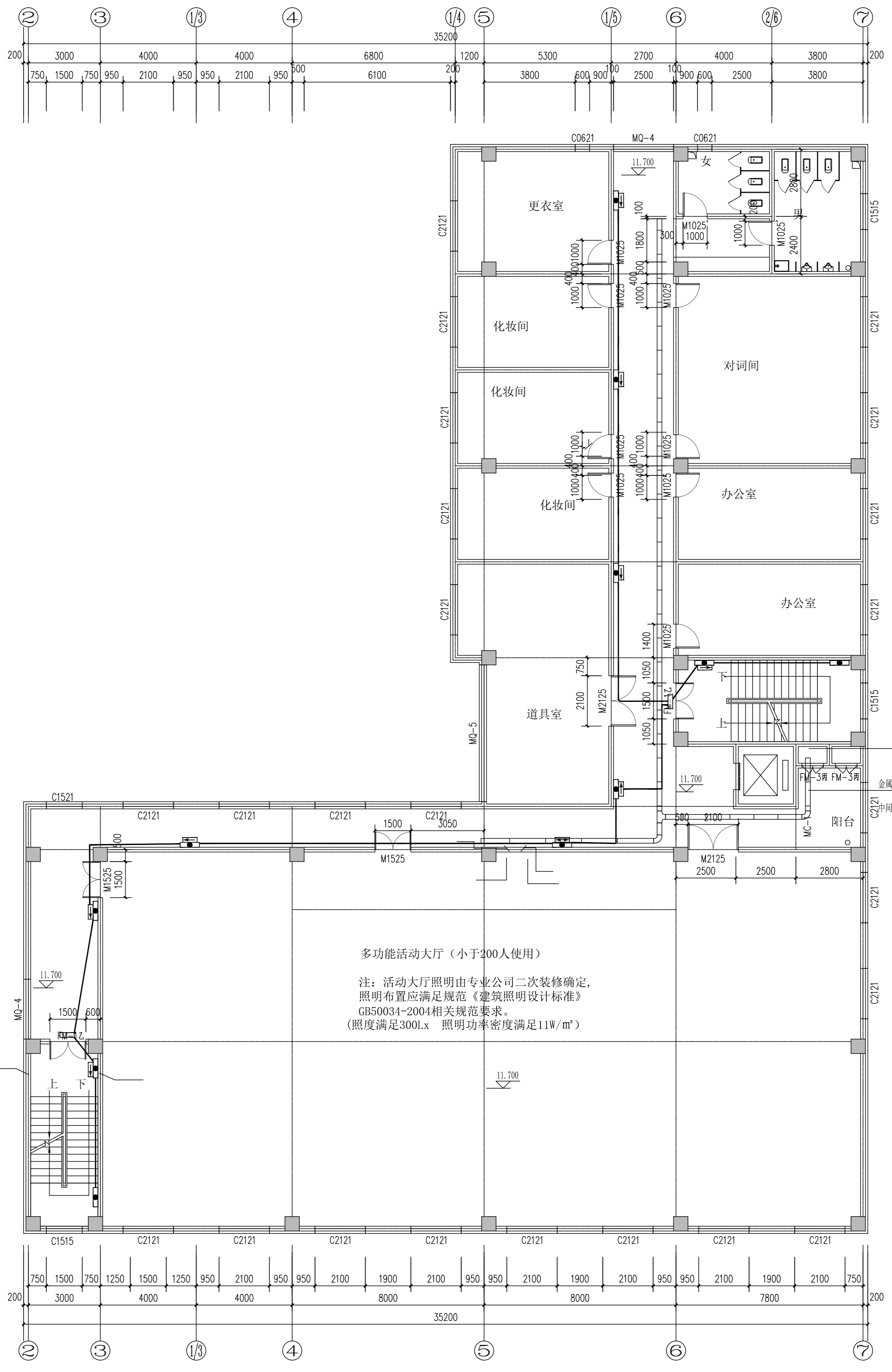
四层照明平面图 1:100
