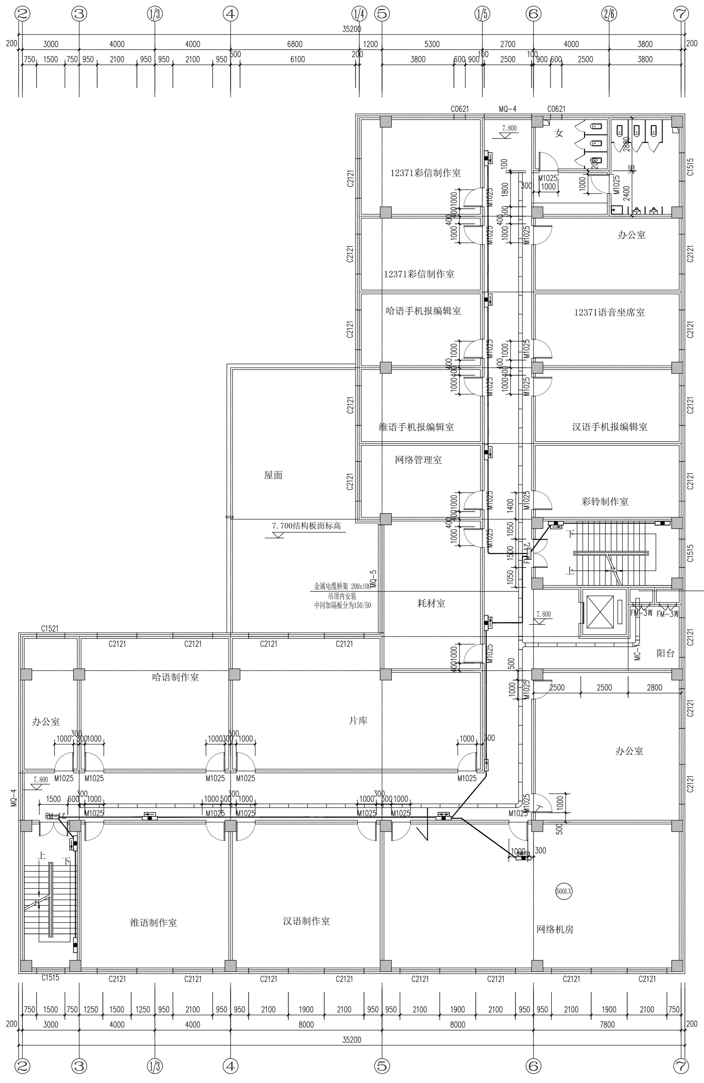
三层照明平面图 1:100
