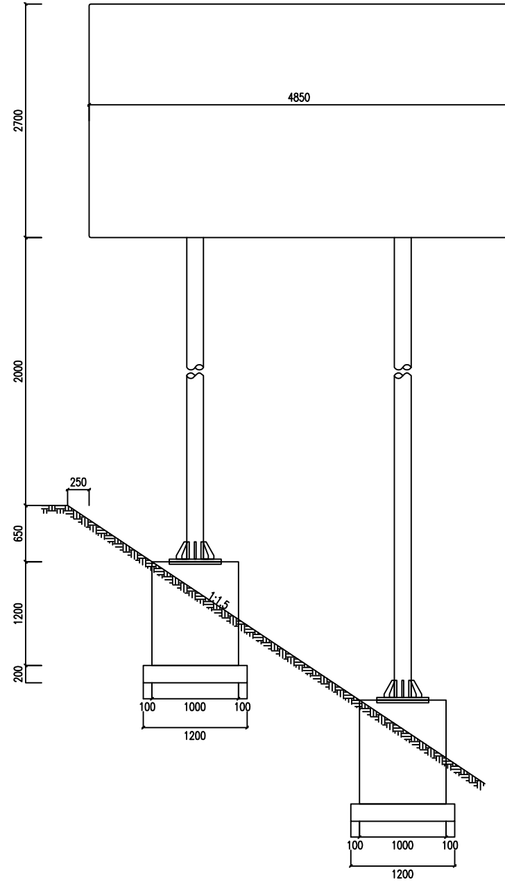
立面图 1:60
