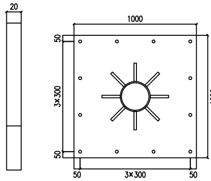
加劲法兰盘
