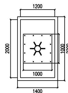
基础平面图
