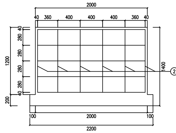
侧面
