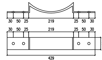
抱箍底衬大样图
