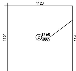
基础箍筋大样图
