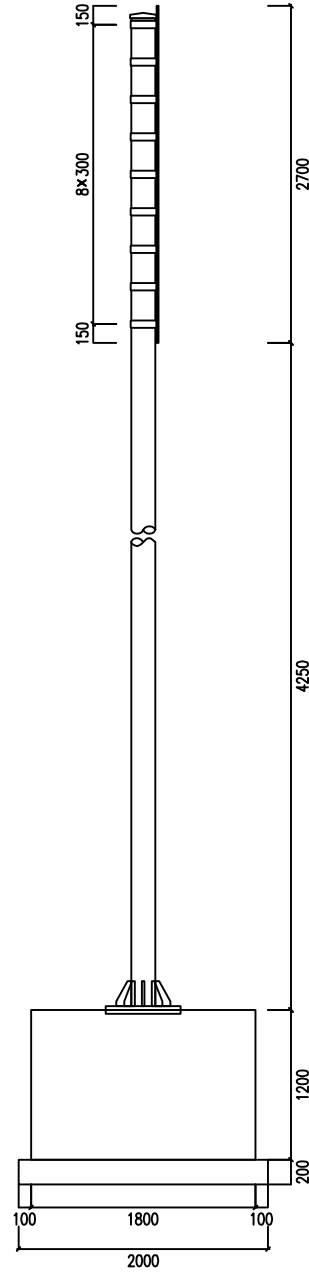
侧面图 1:60
