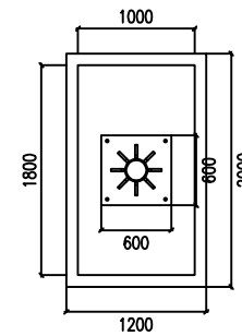
基础平面图 1:70
