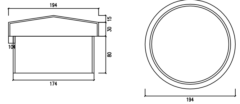
柱帽大样图
