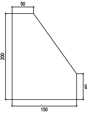
加劲肋构造图
