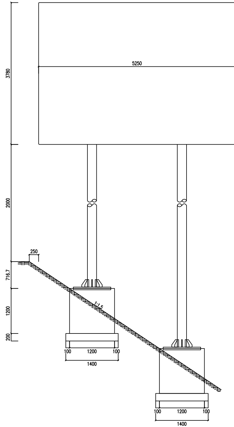
立面图
