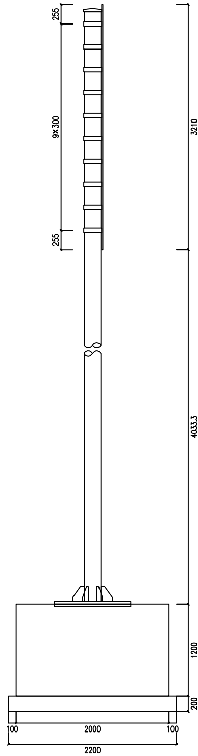
侧面图
