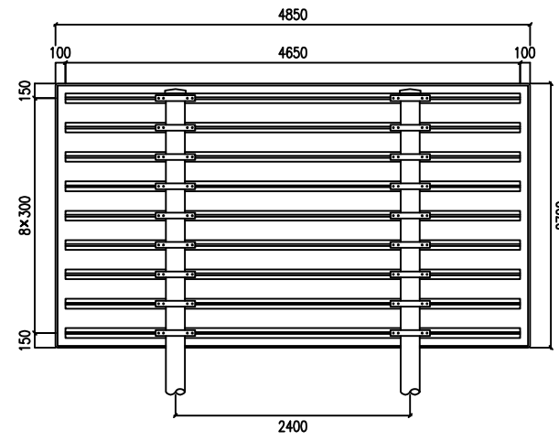
标志板与立柱联结示意图 1:70
