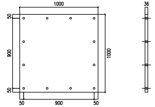
底座法兰盘
