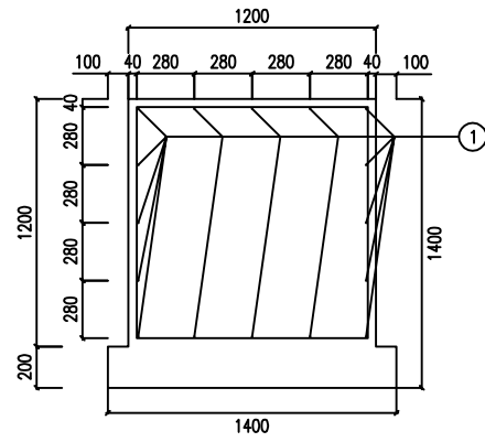
立面
