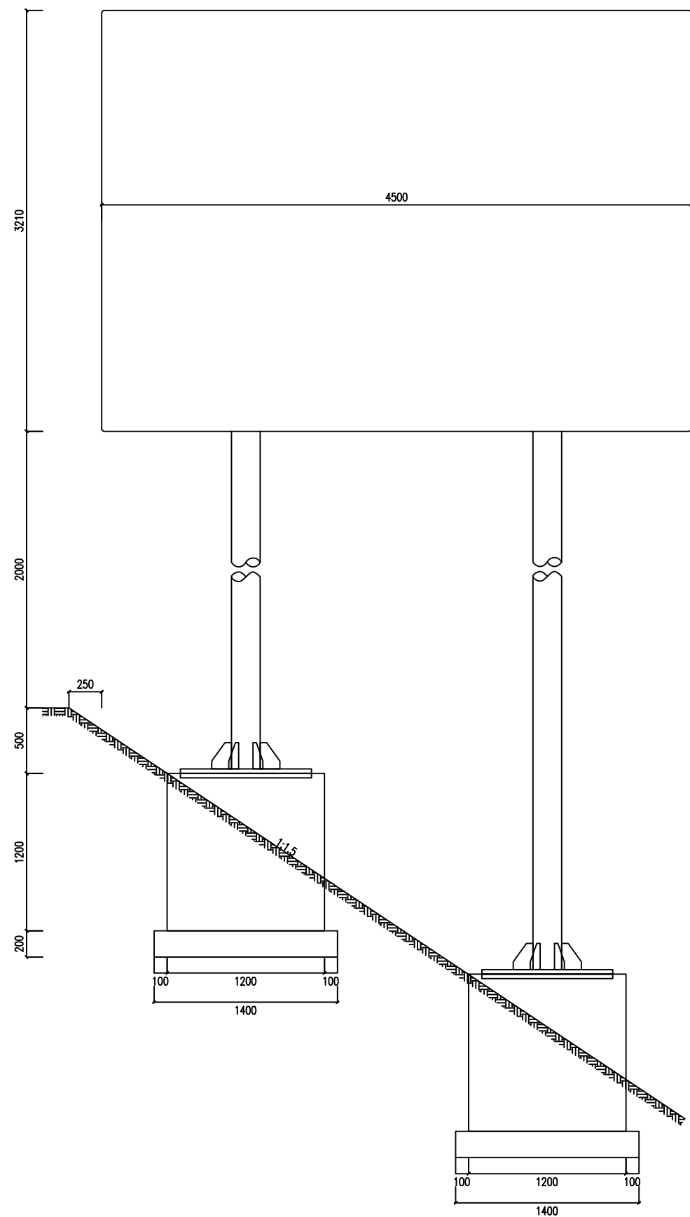
立面图
