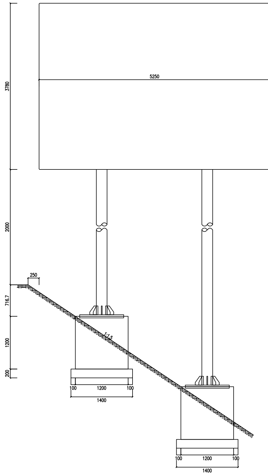
立面图
