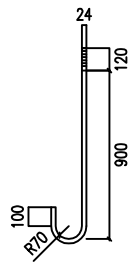
地脚螺栓大样图
