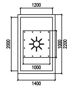
基础平面图
