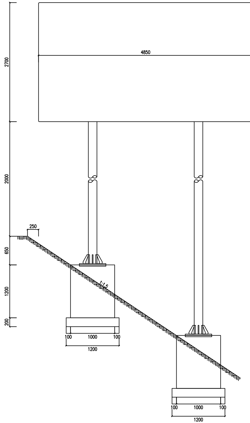
立面图 1:50
