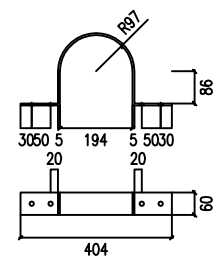
抱箍大样图 1:20
