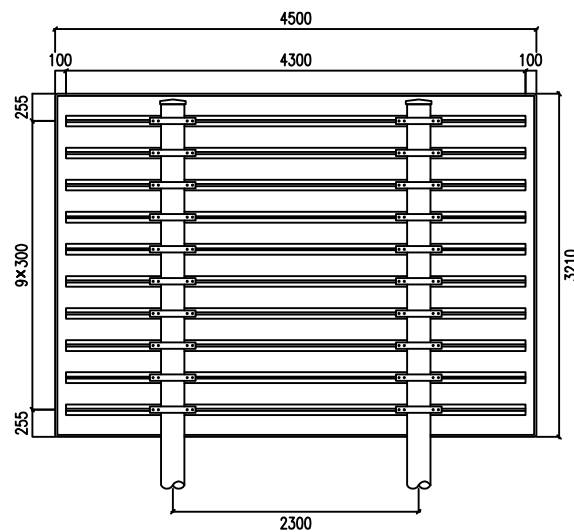
标志板与立柱联结示意图
