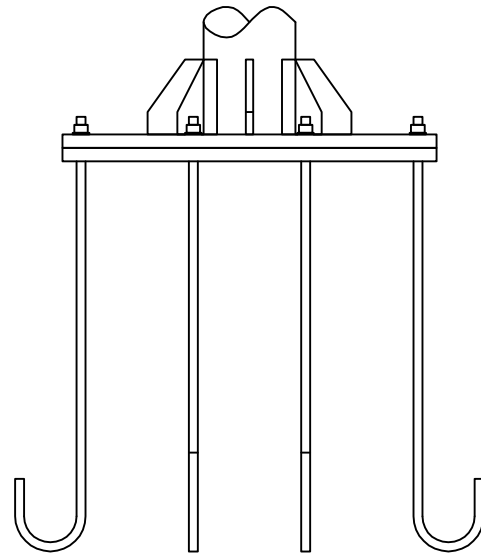
底座连接大样
