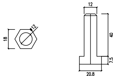
滑动螺栓大样
