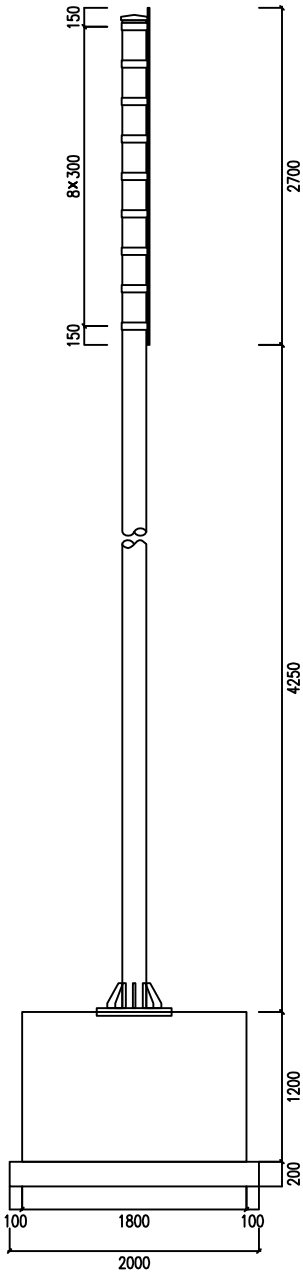
侧面图
