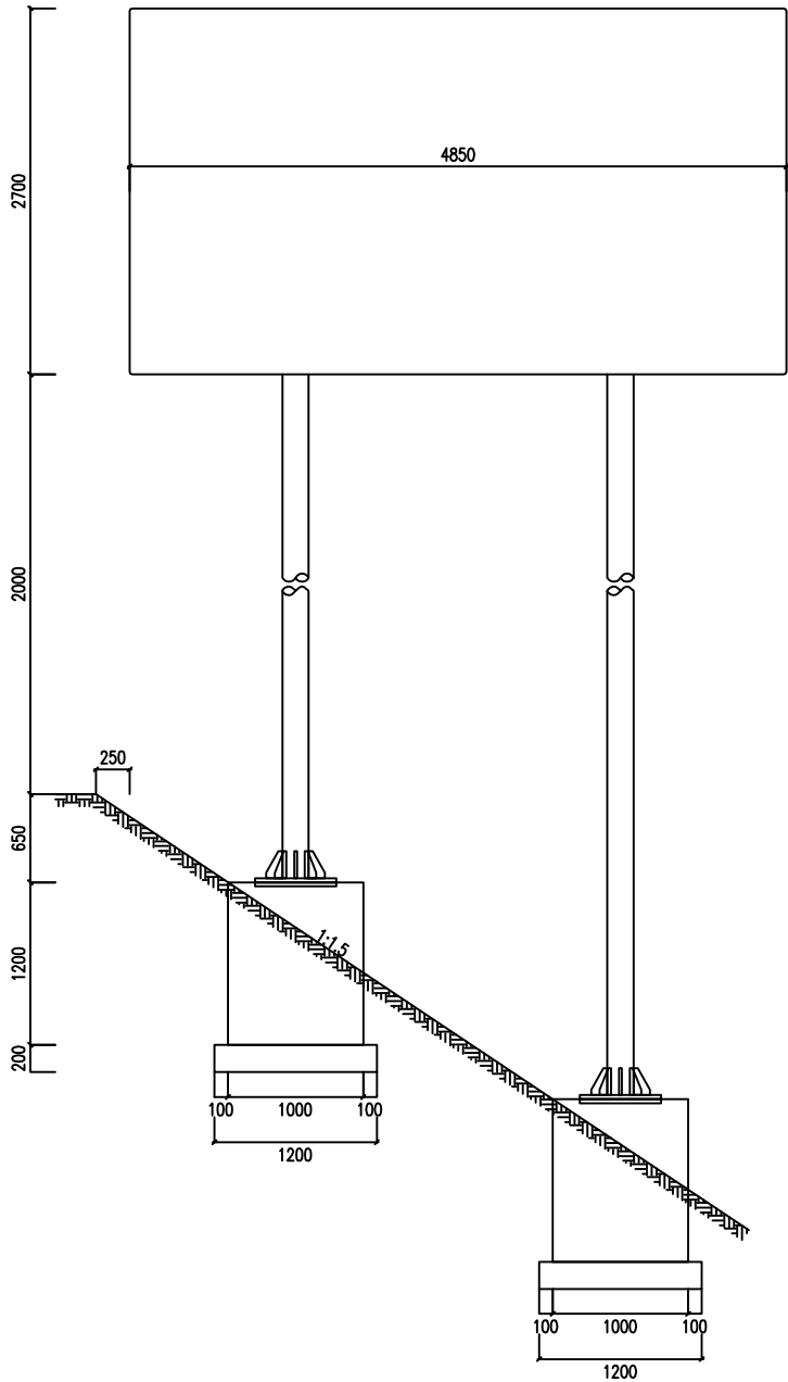
立面图
