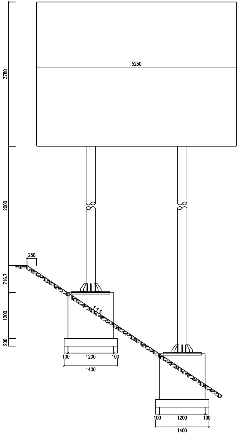
立面图
