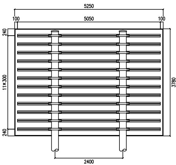
标志板与立柱联结示意图
