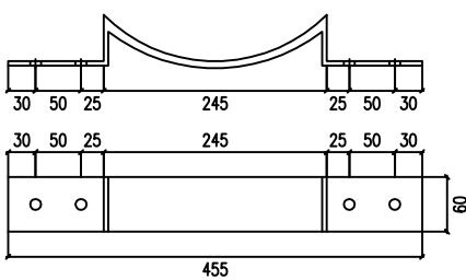
抱箍底衬大样图
