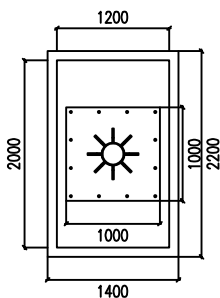
基础平面图
