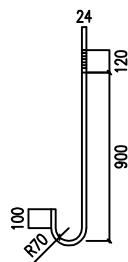
地脚螺栓大样图
