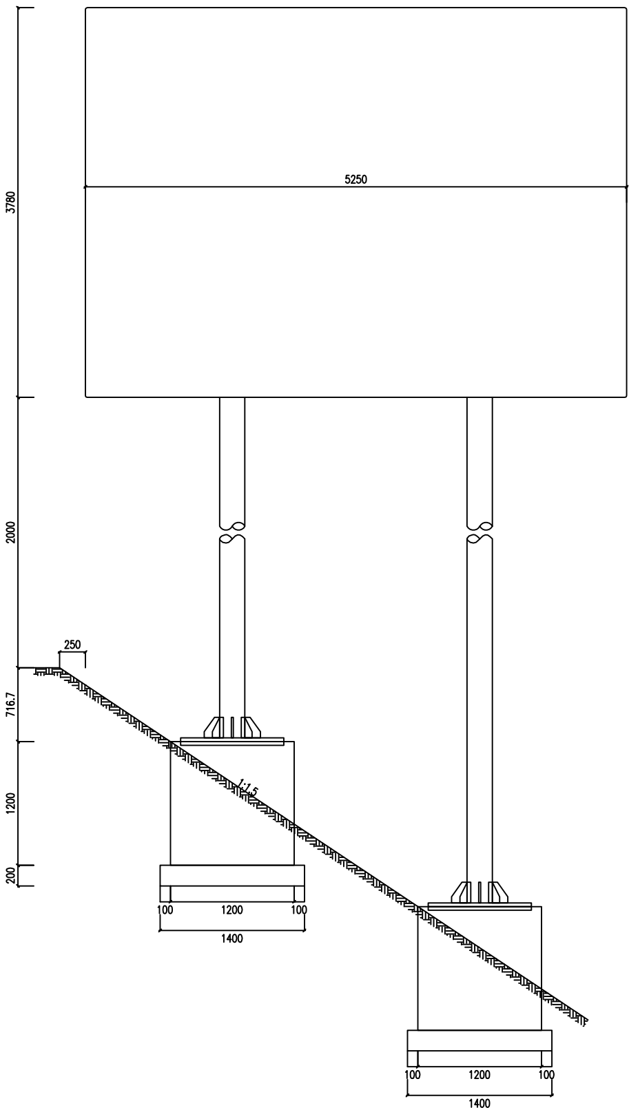
立面图
