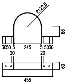
抱箍大样图
