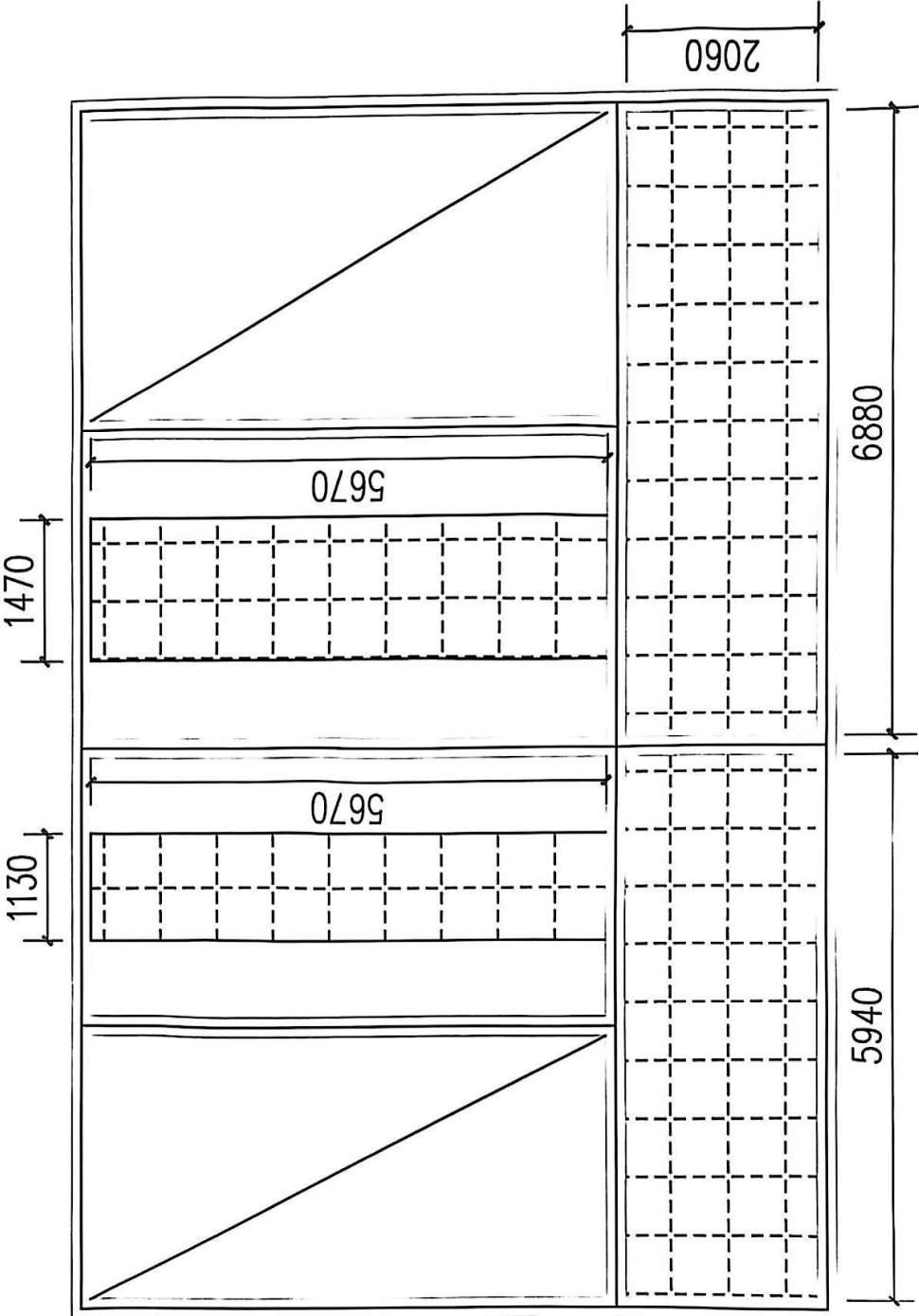
铜新小学卫生间贴砖平面图
