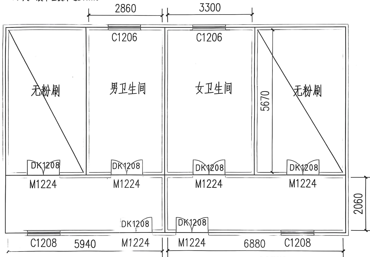
铜新小学卫生间墙面粉刷平面图
