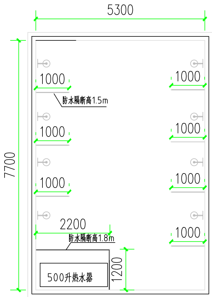
杜热中学女生洗衣间改洗澡堂平面图
