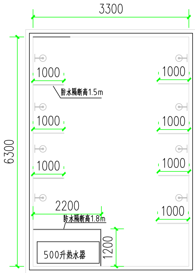
杜热中男生卫生间改洗澡堂平面图
