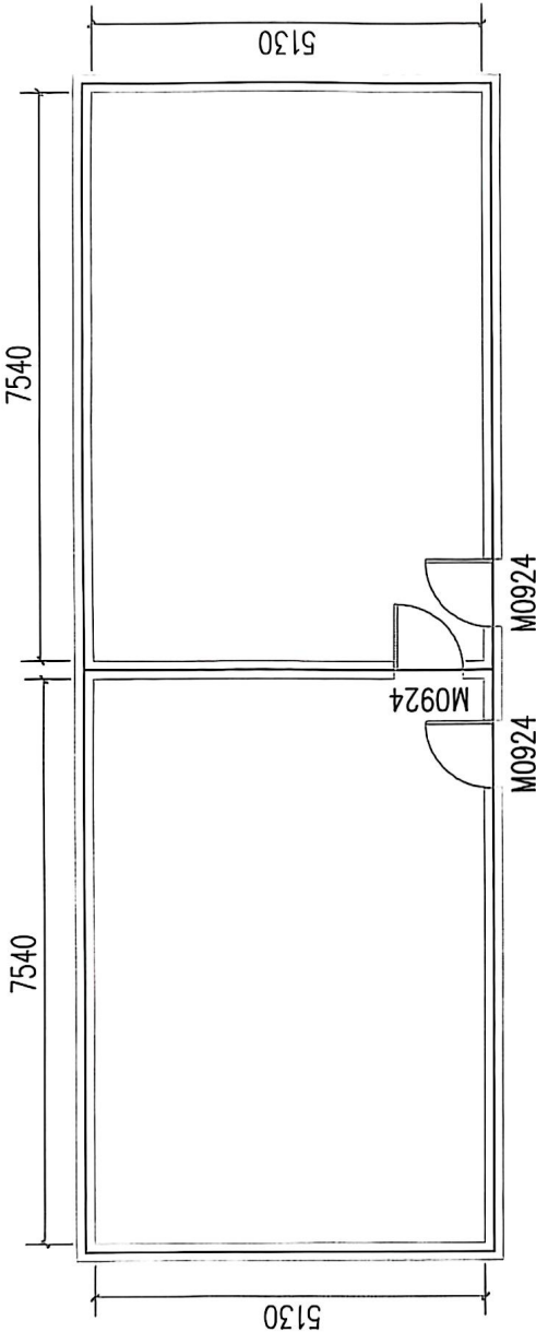
幼儿园大班、寝室木地板平面图
