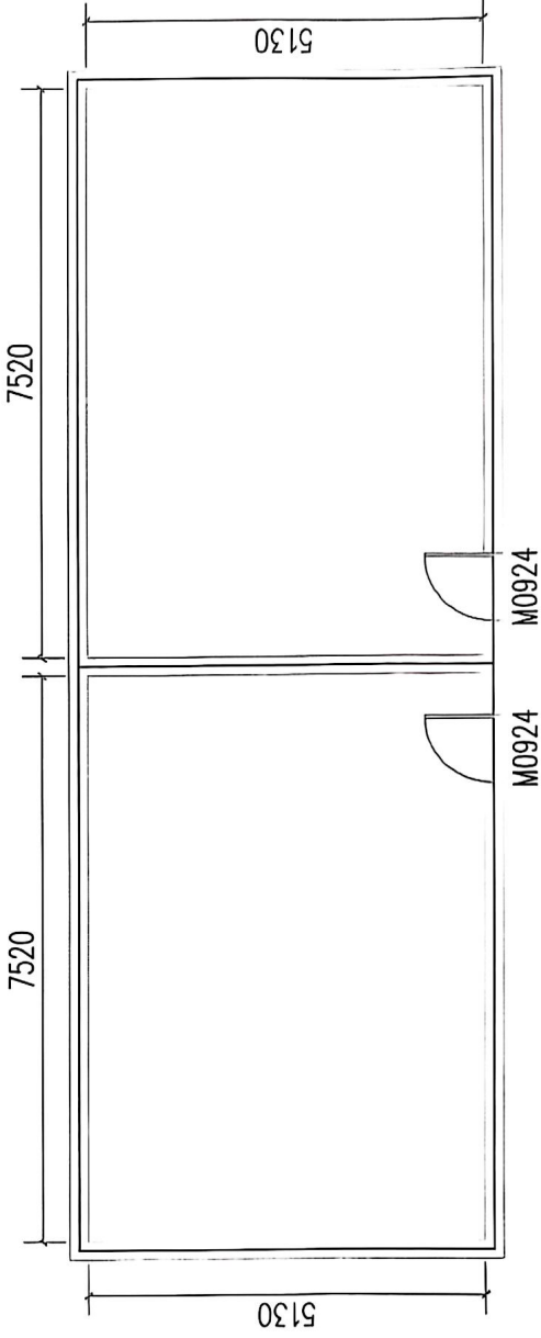
幼儿园中班、小班木地板平面图
