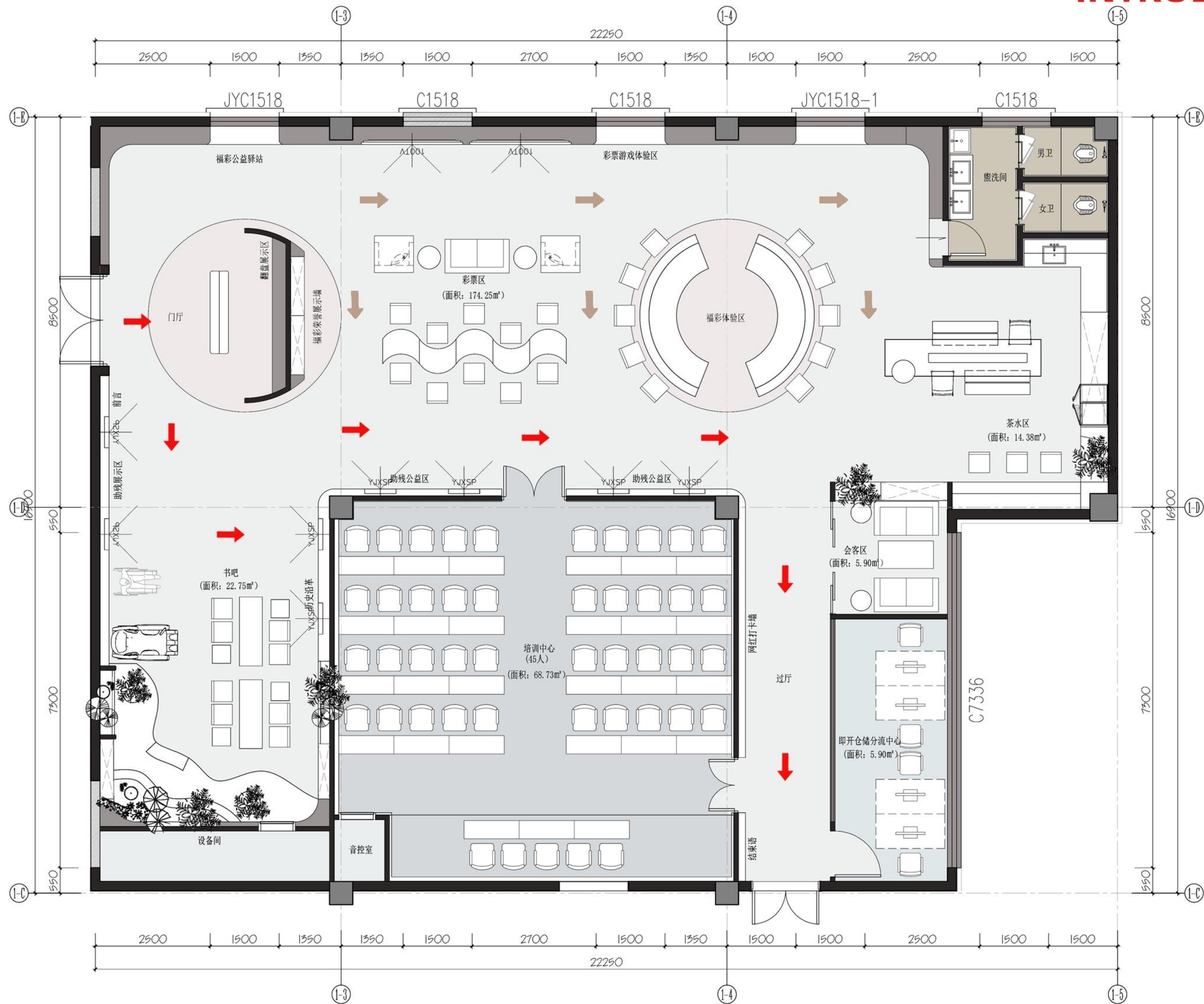
平面布置图 PLAN
