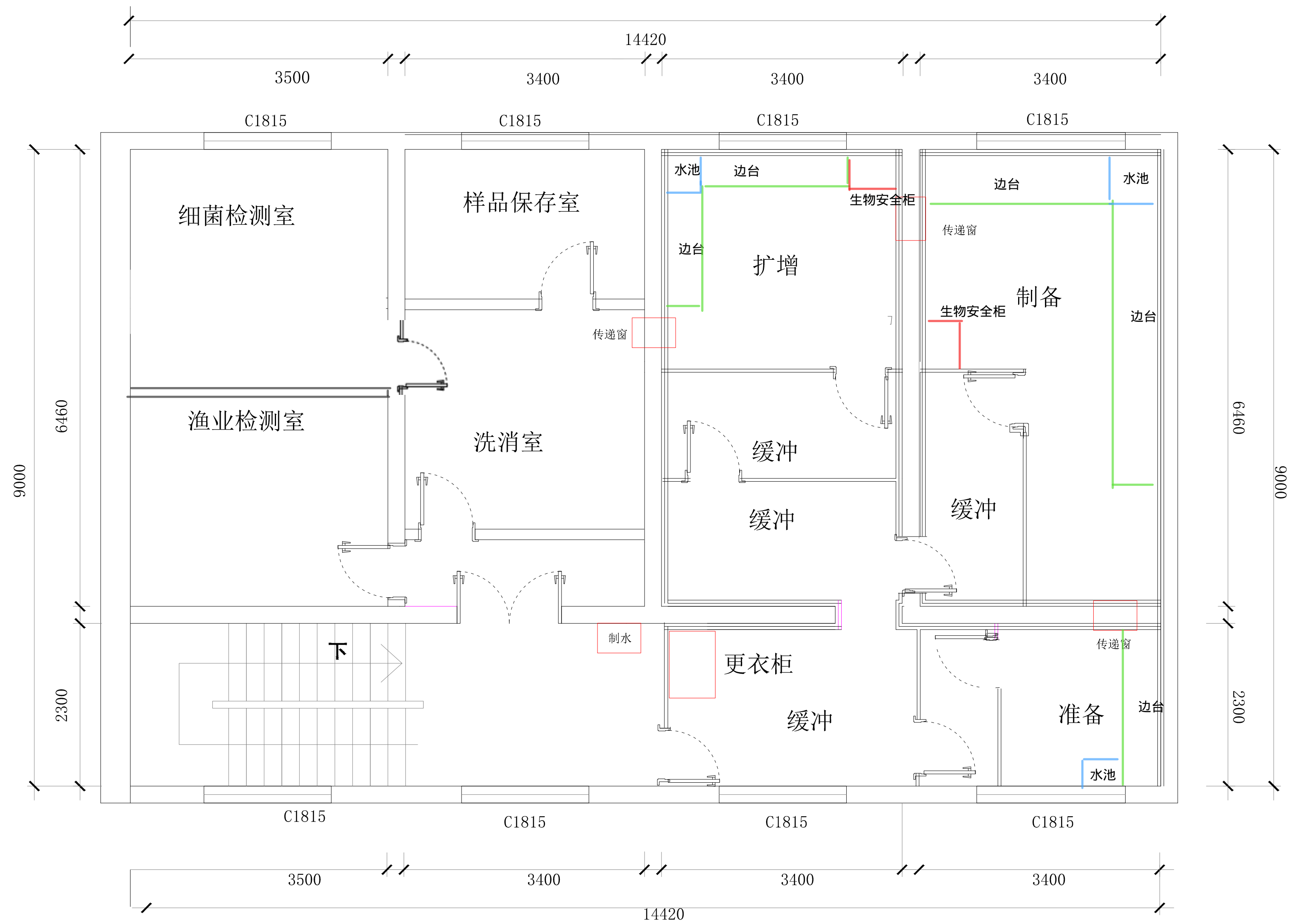
二层平面框架
