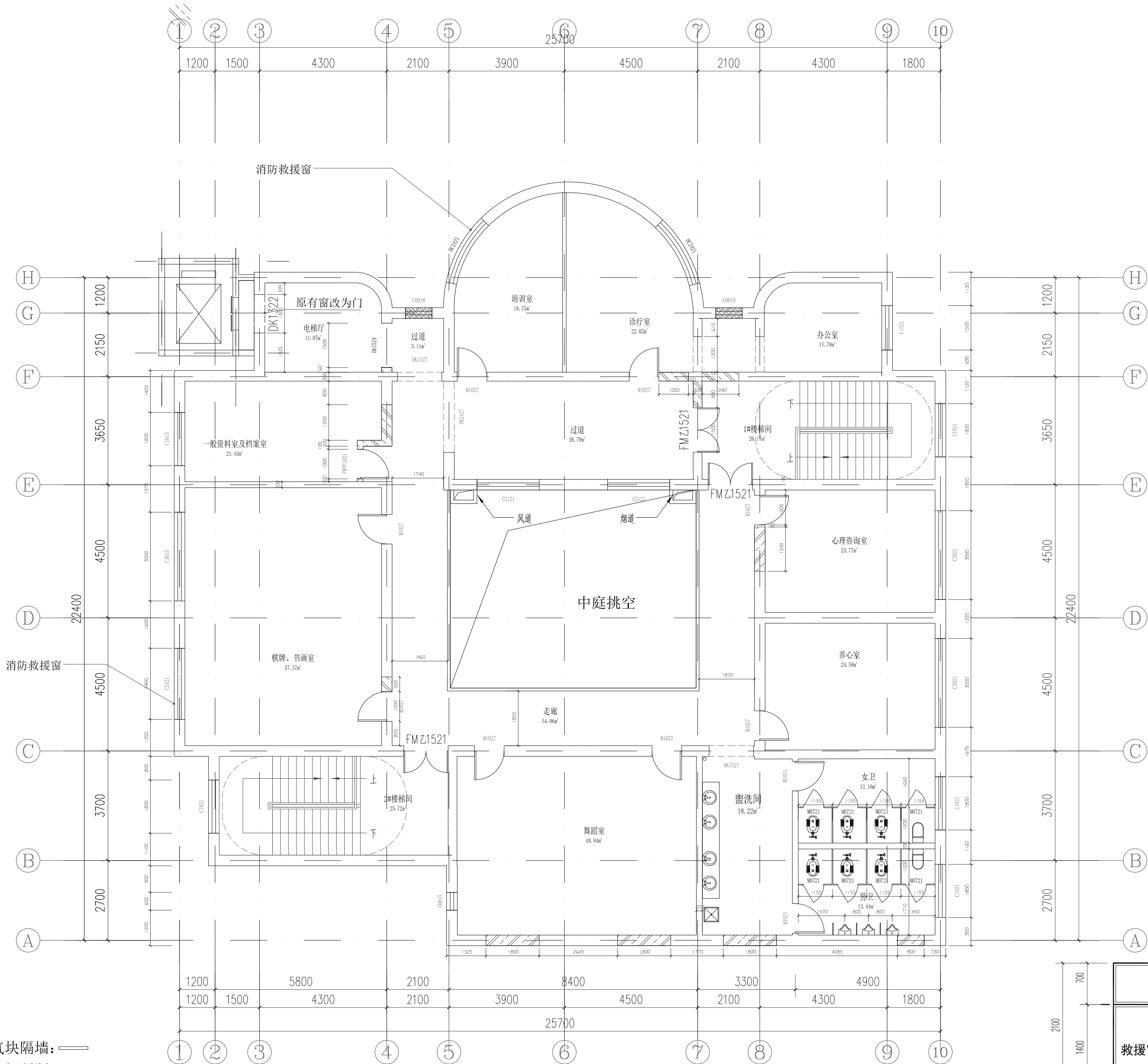
二层平面布置及新增隔墙图 1:100
