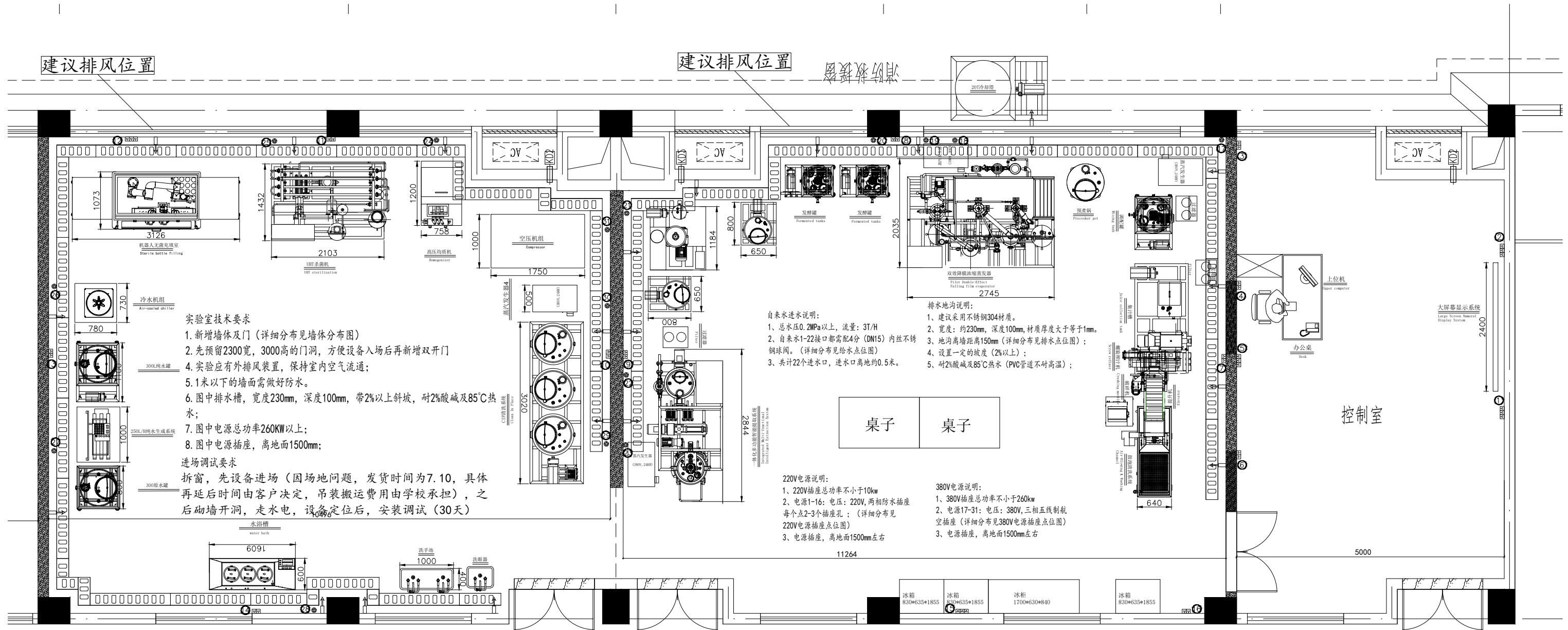
1-设备布局图及要求
