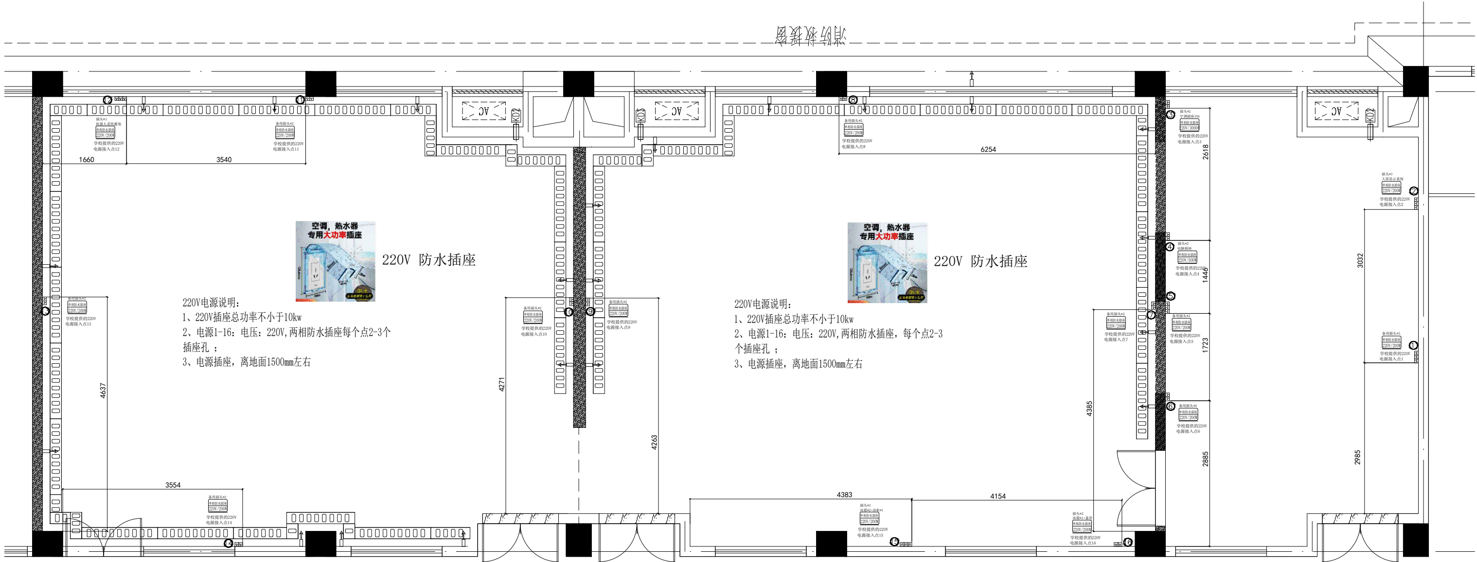
5-220V防水插座点位
