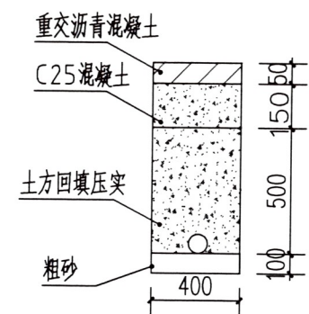
沥青路面开挖、回填断面图
