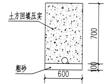
土方开挖、回填断面图
