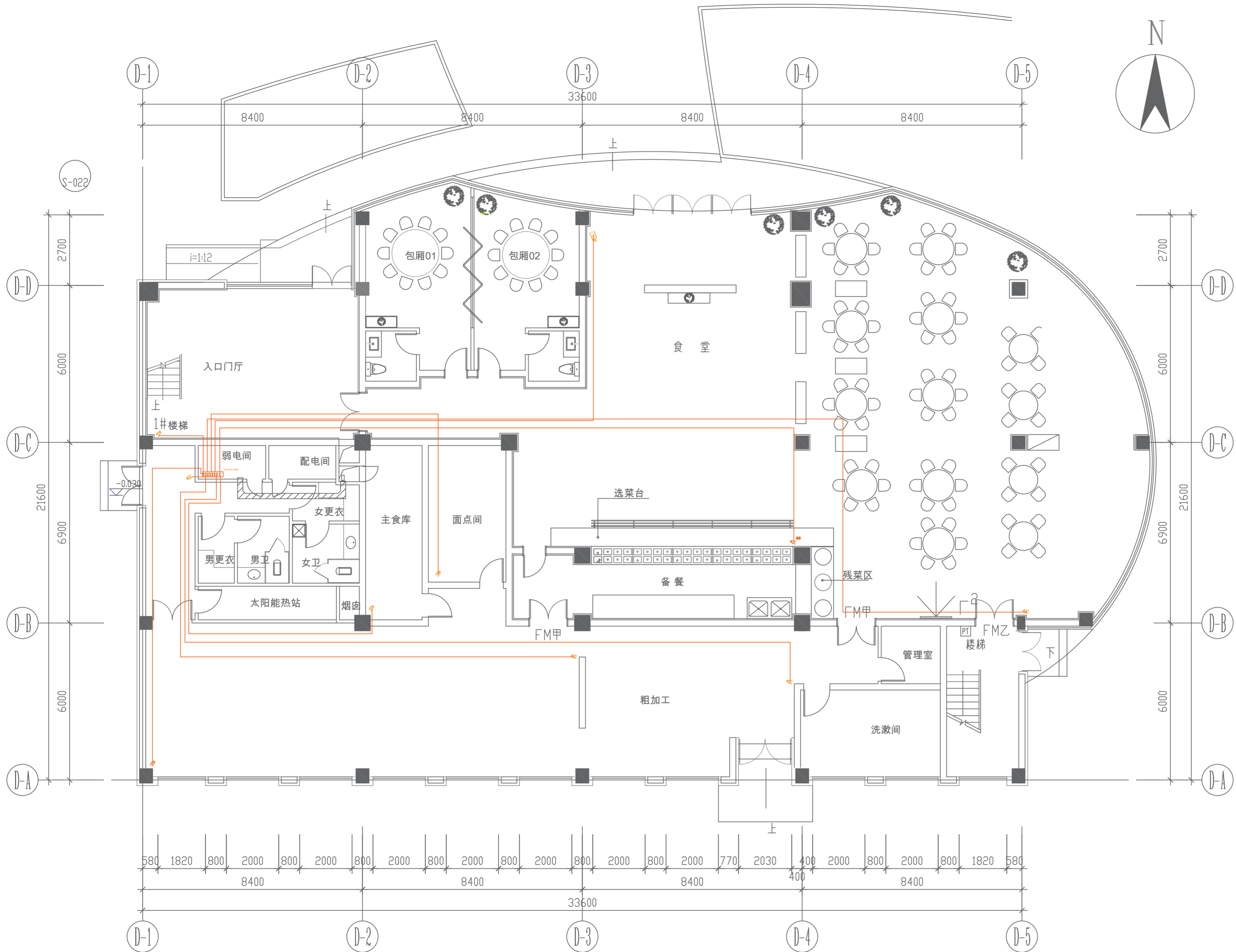
D楼一层平面图 1:100
