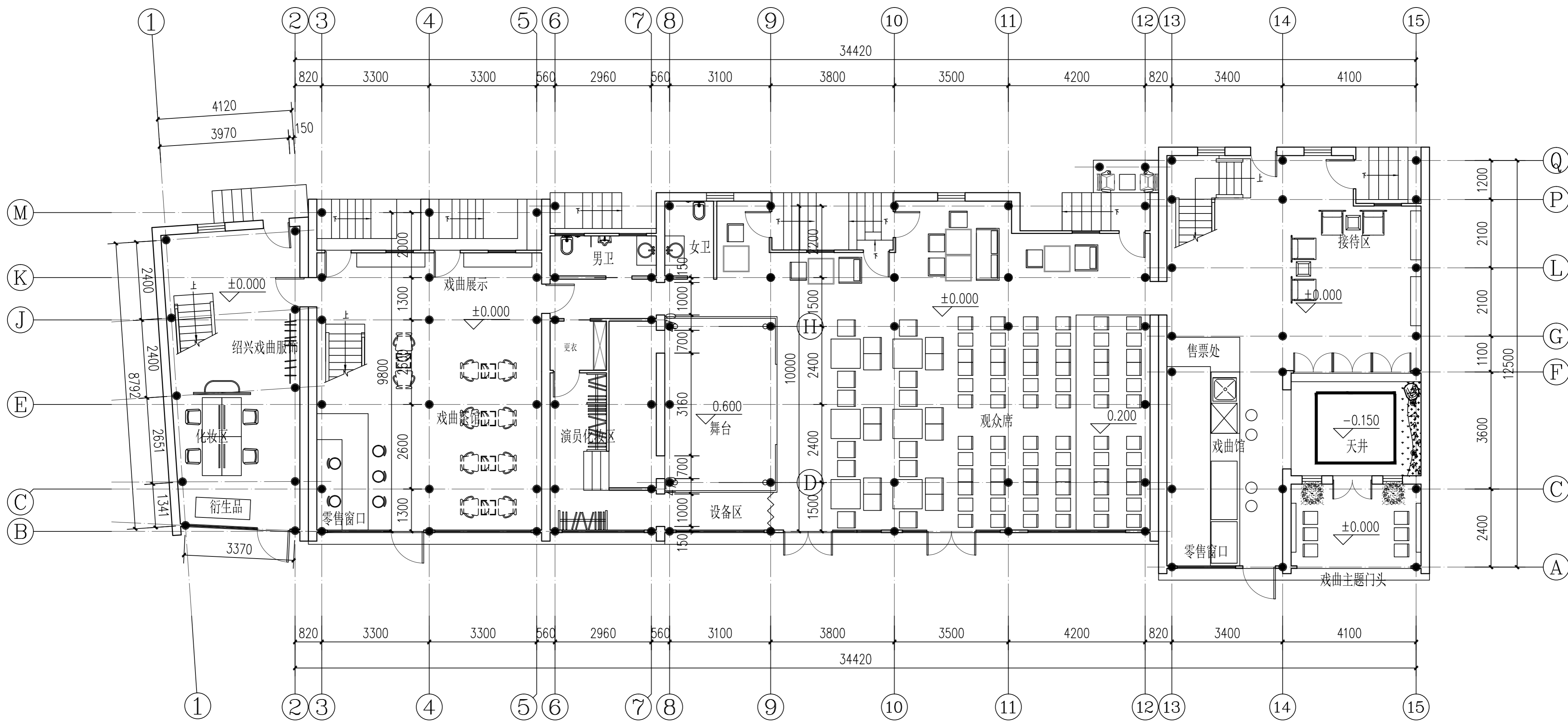
一层平面图 1:100
