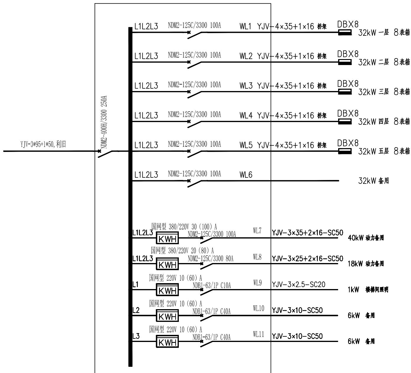
宿舍单元底层总开关箱DZKX52系统图
