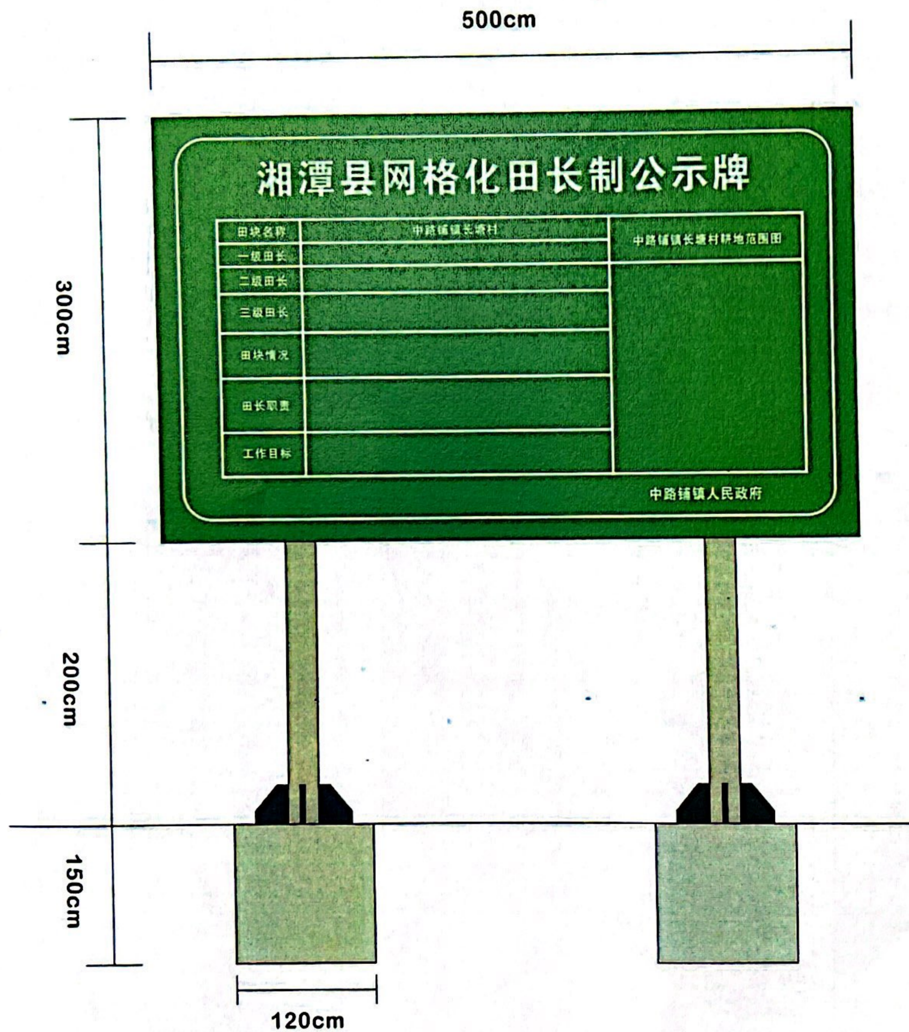
正面效果图-①
