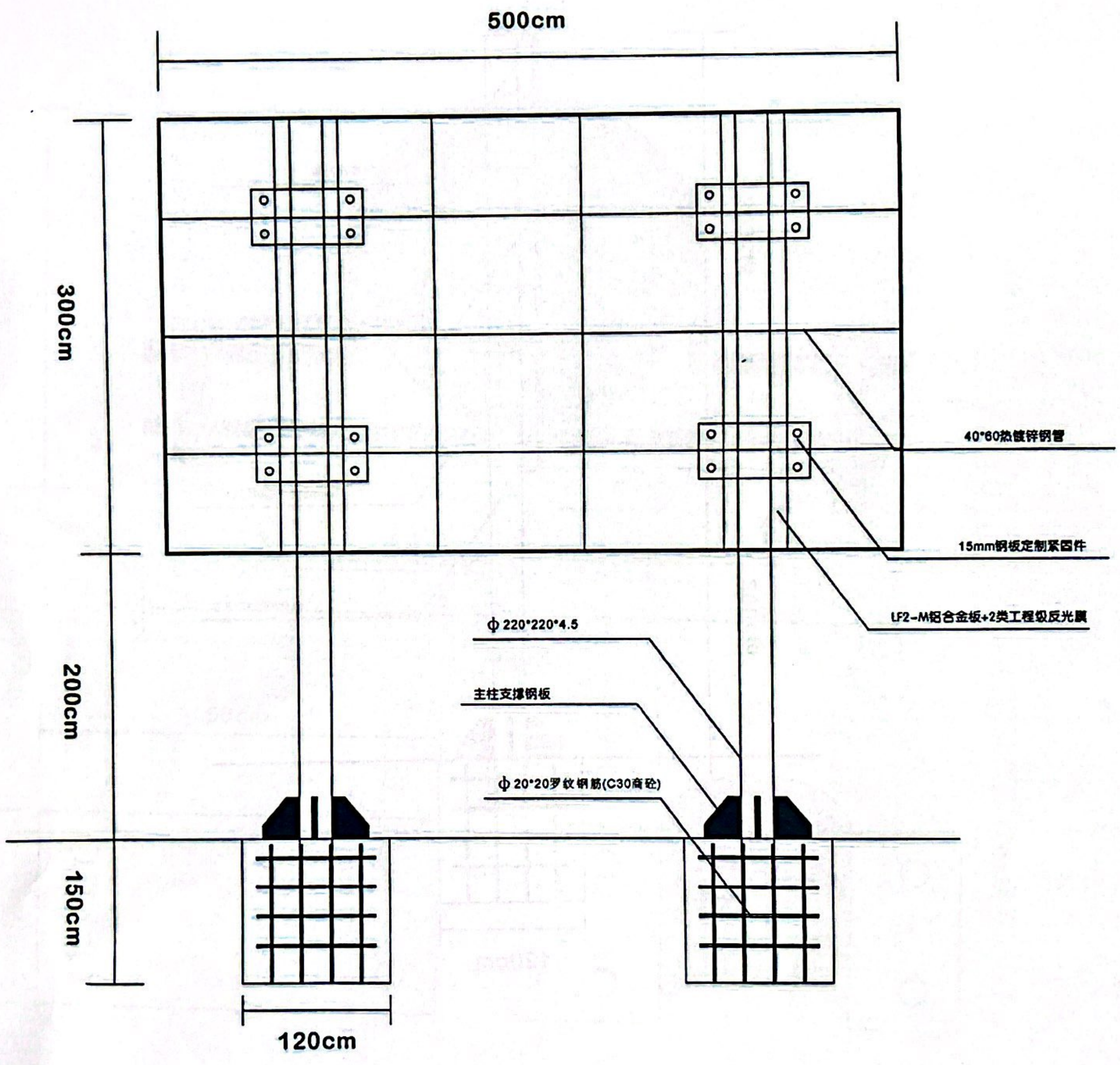
正面结构图-②
