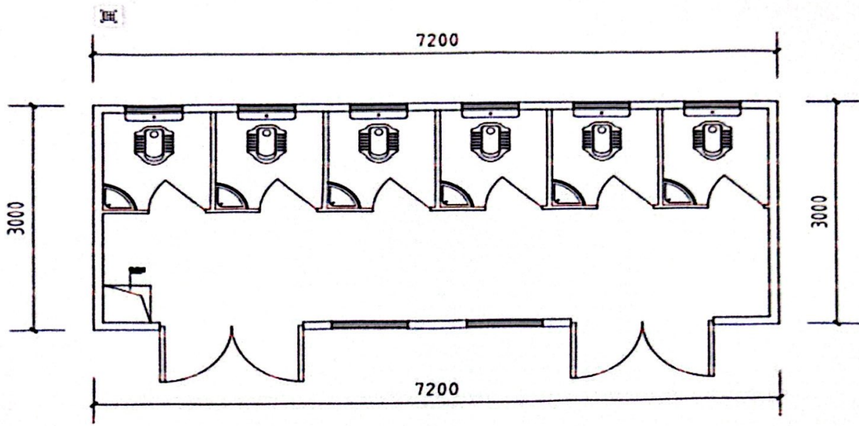
6蹲位泡沫封堵式厕所平面图
