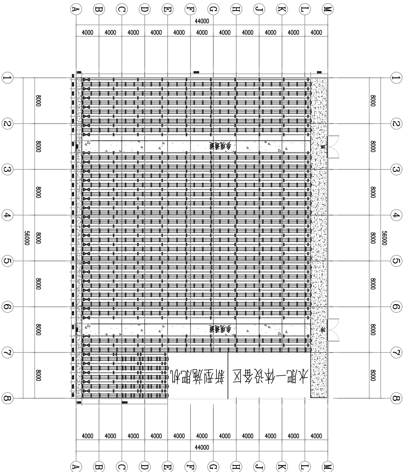
文架番茄栽培布置图 1:100
