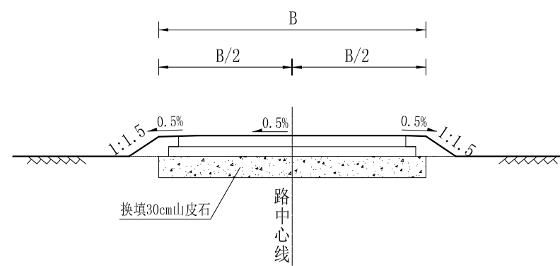
特殊路基设计图(旧路翻浆段)
