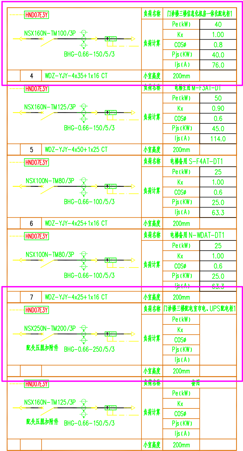
2AN7低压馈电柜
