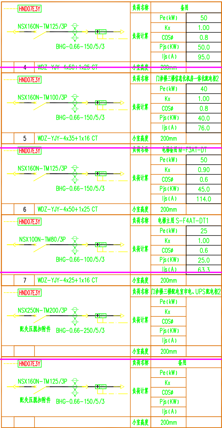
1AN7低压馈电柜
