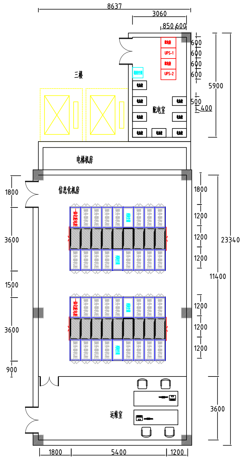
机房平面布置图
