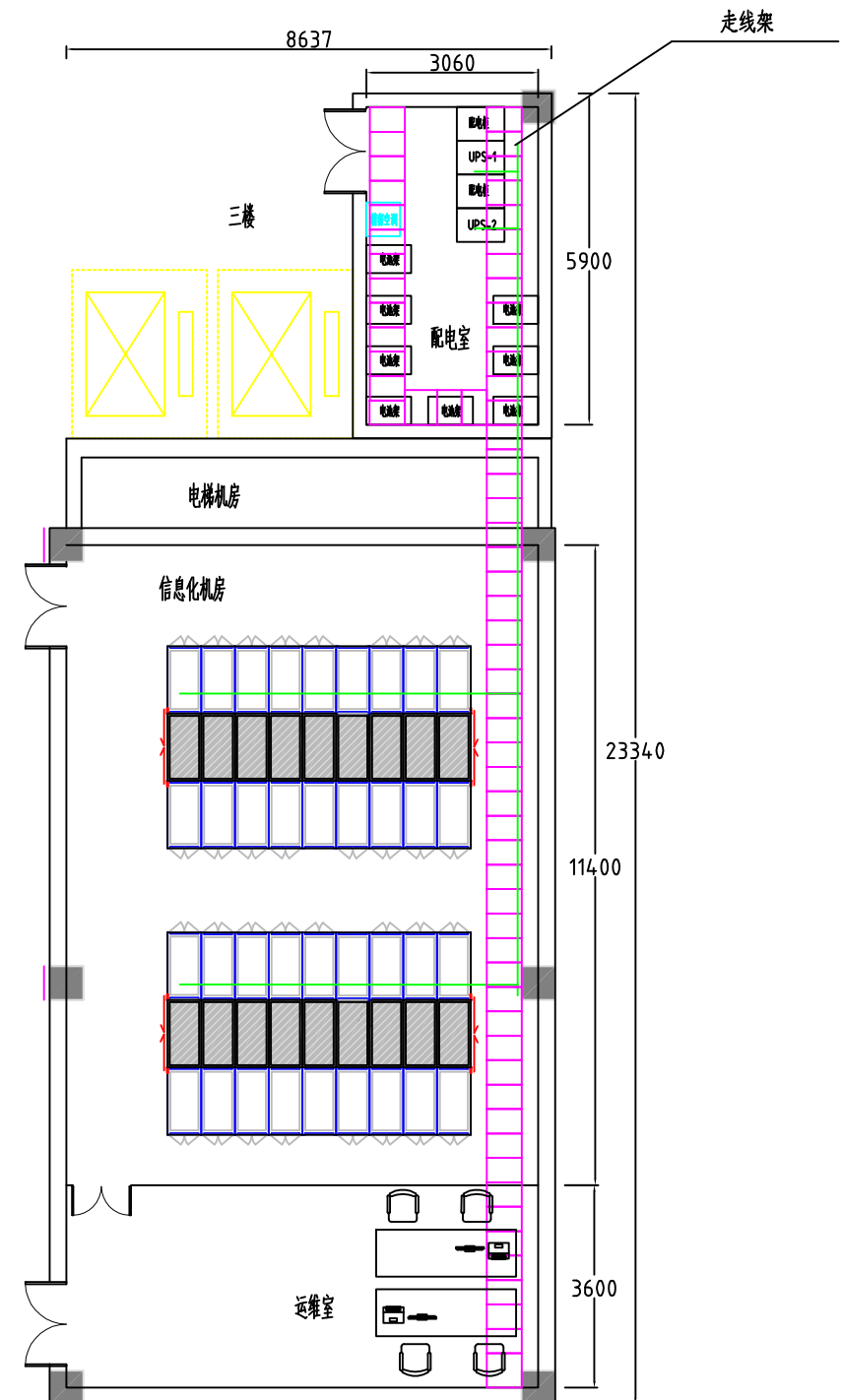
机房走线及路由图
