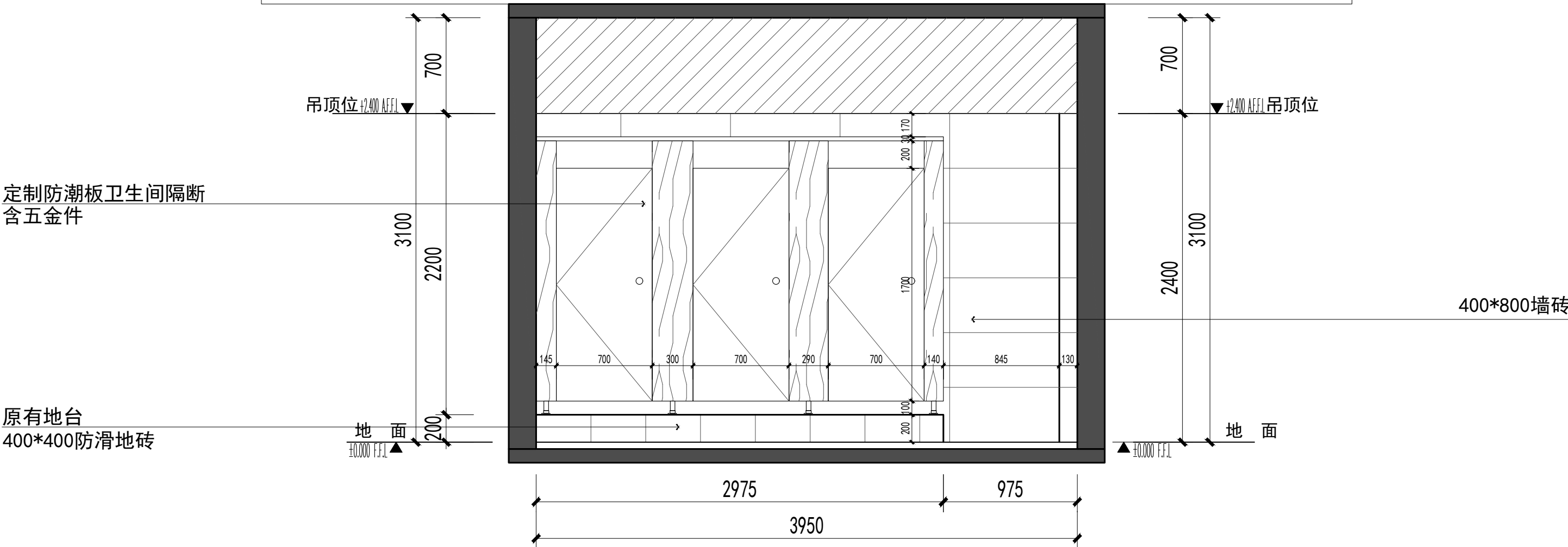
3F-9F男卫生间1F-06-D立面图 1:30
