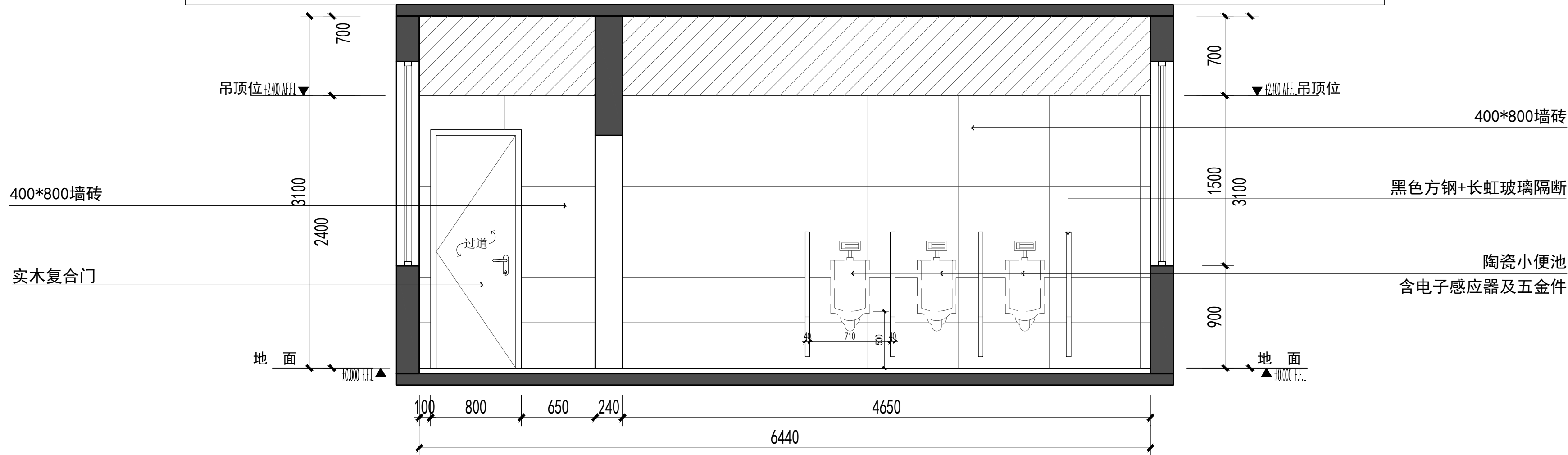
10F、11F男卫生间1F-07-C立面图 1:30
