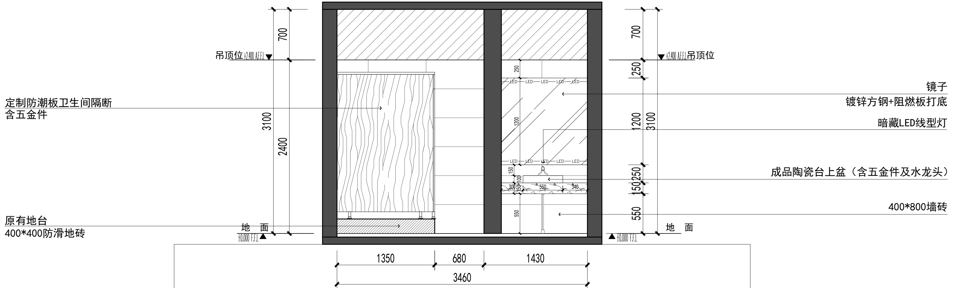
10F、11F男卫生间1F-08-A立面图 1:30
