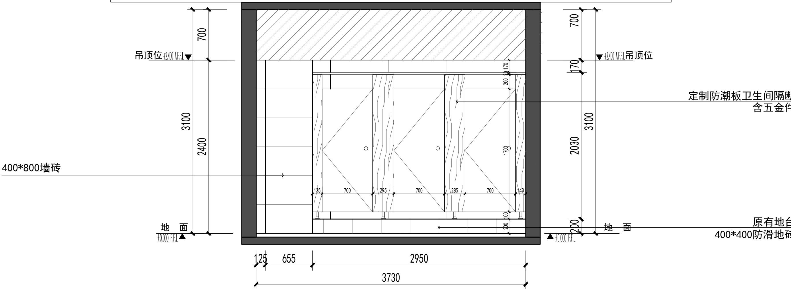
1F、2F女卫生间1F-01-A立面图 1:30
