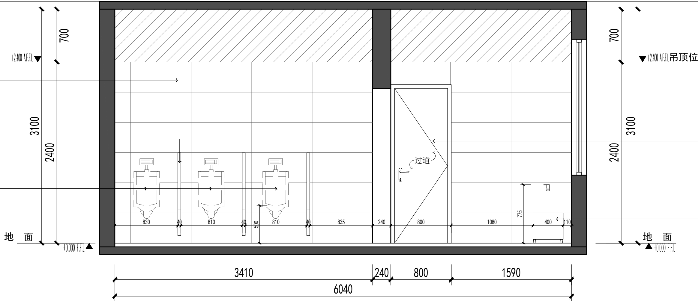
3F-9F男卫生间1F-04-C立面图 1:30
