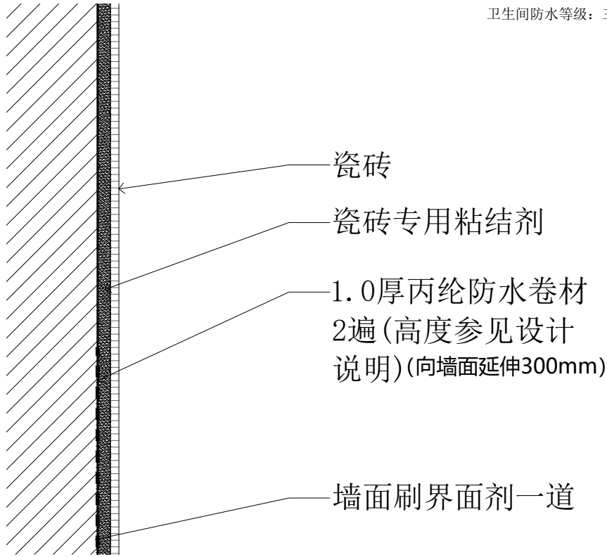
卫生间墙面瓷砖大样图 1:5
