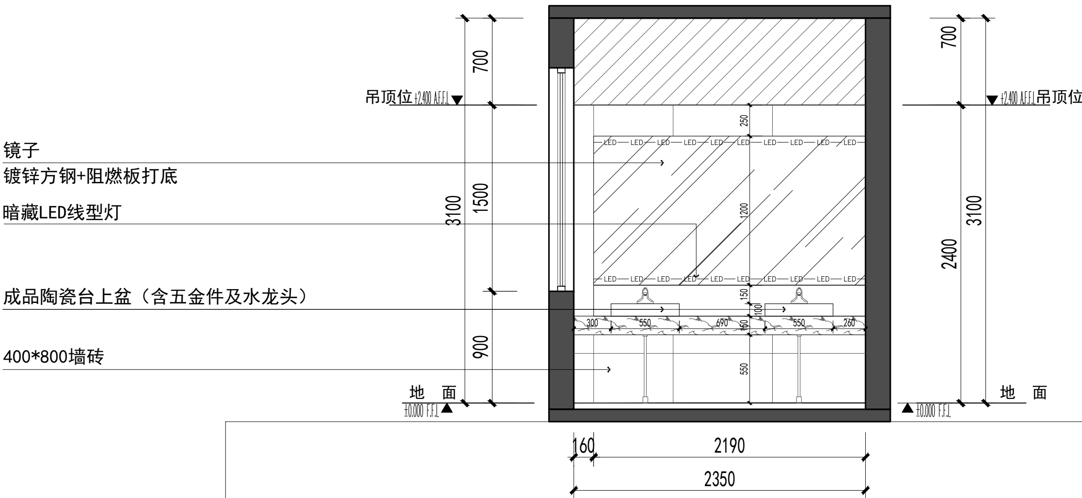
3F-9F男卫生间1F-05-D立面图 1:30
