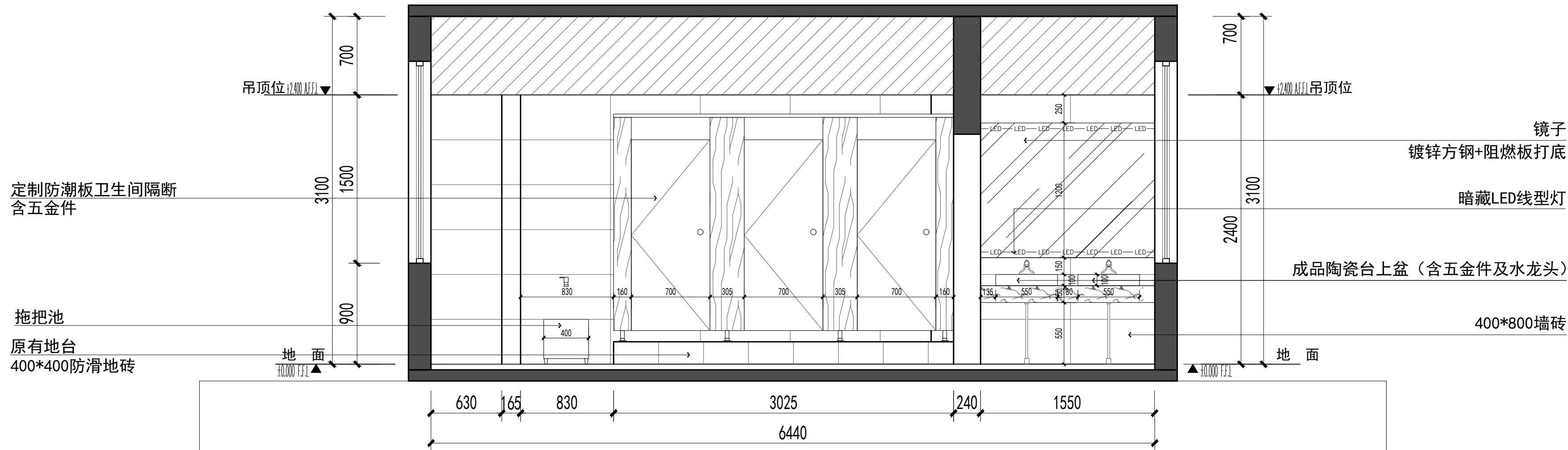
10F、11F男卫生间1F-07-A立面图 1:30
