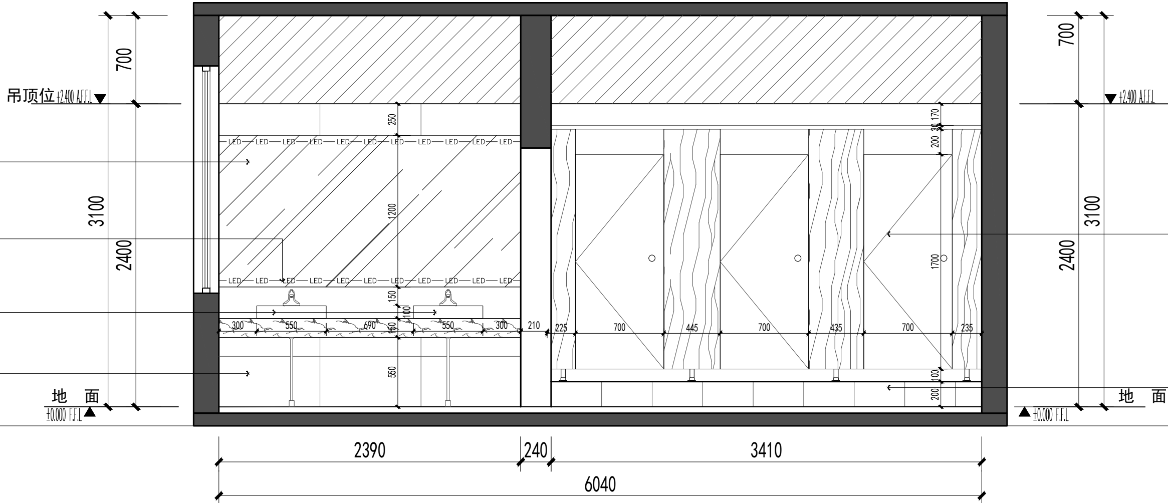
3F-9F男卫生间1F-04-A立面图 1:30
