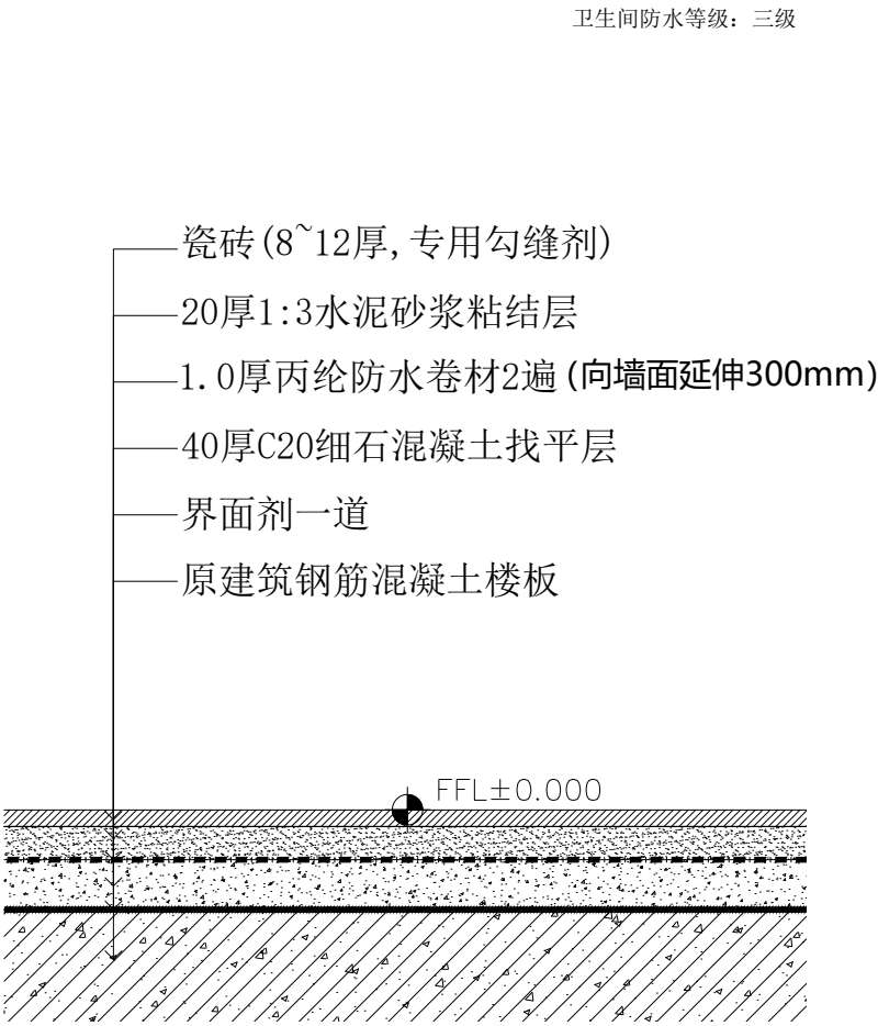
卫生间地面瓷砖大样图 1:5
