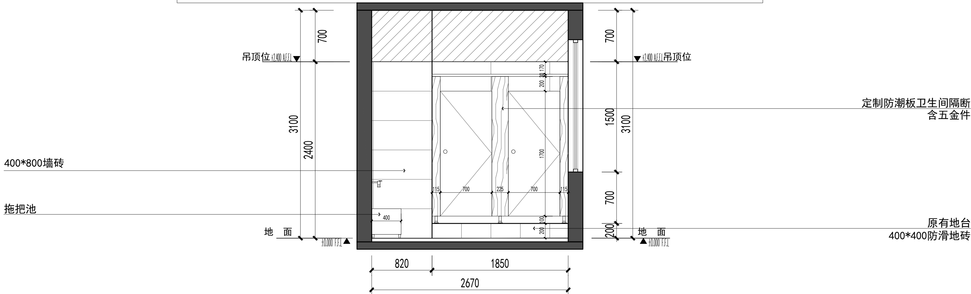
10F、11F男卫生间1F-08-D立面图 1:30
