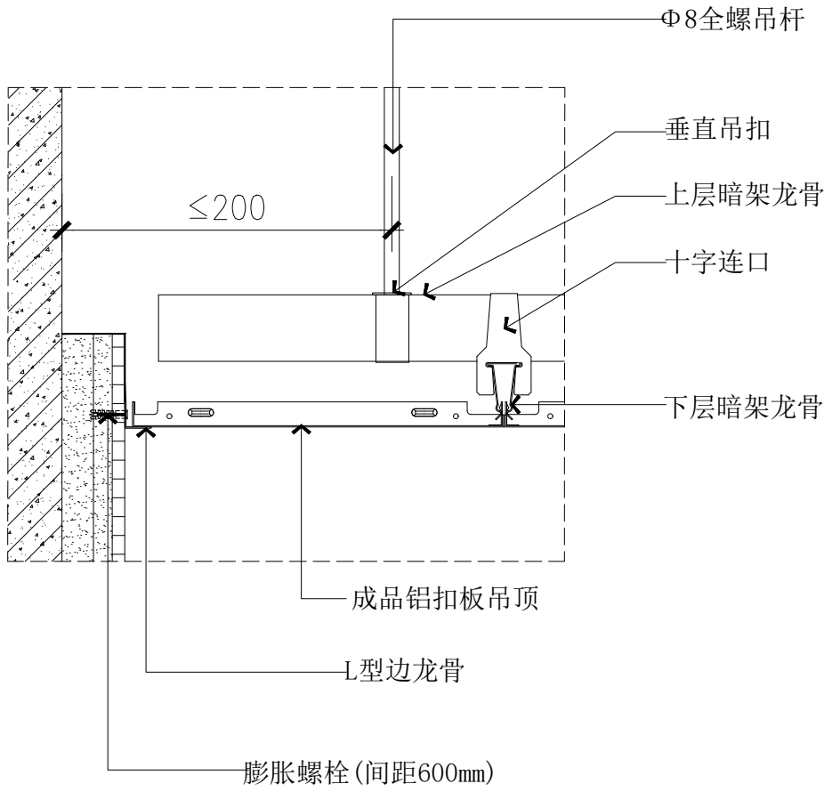
铝扣板吊顶A大样图 1:5
