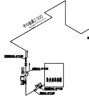
水表加药管路系统图
