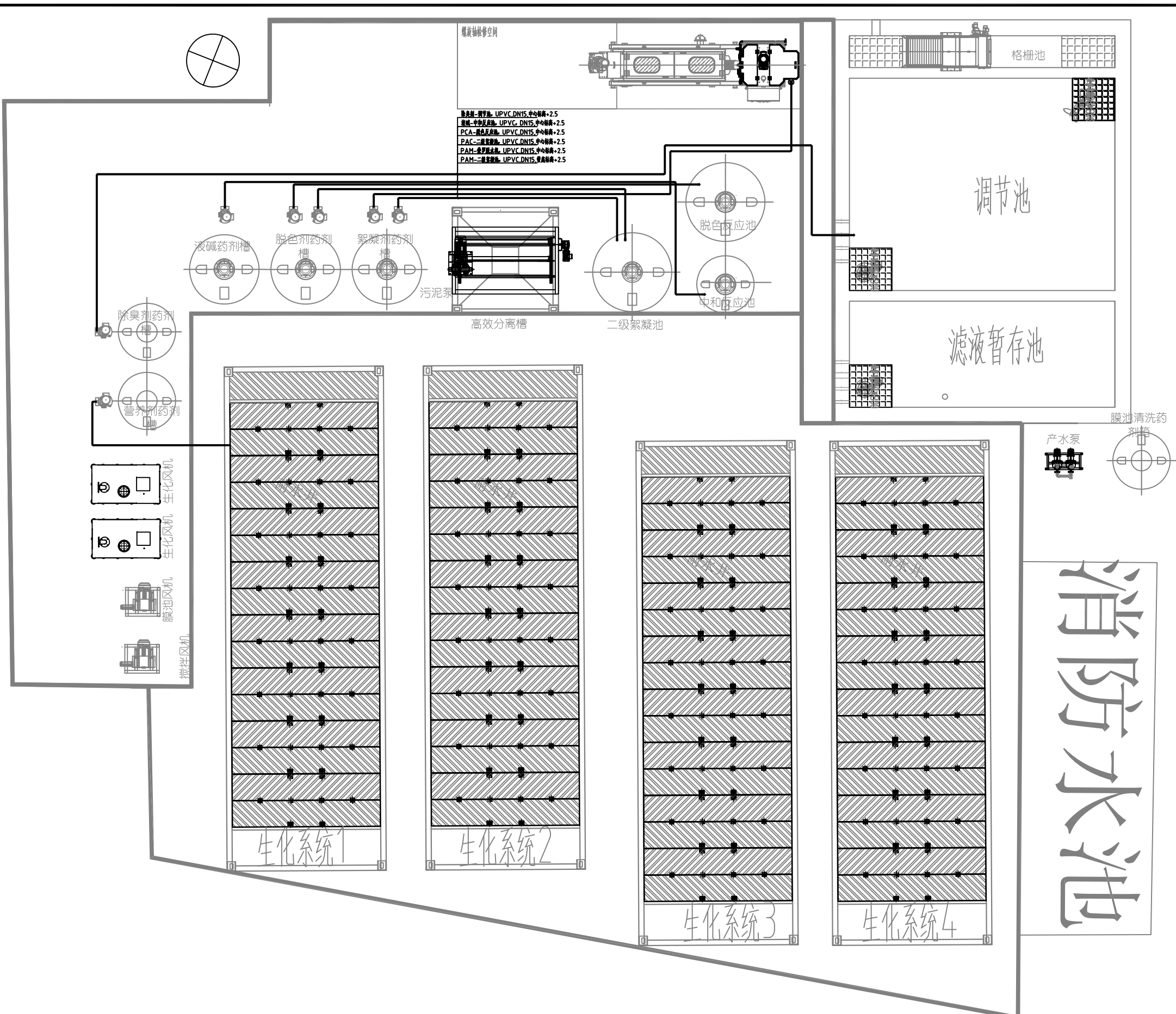
加药管路系统图
