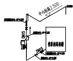
水表加药管路系统图
