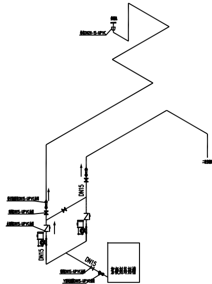
水表加药管路系统图
