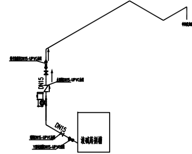
水表加药管路系统图
