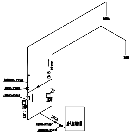
水表加药管路系统图
