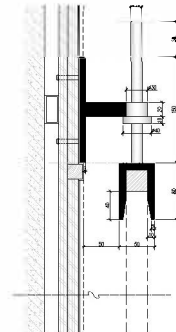
画框节点示意:
