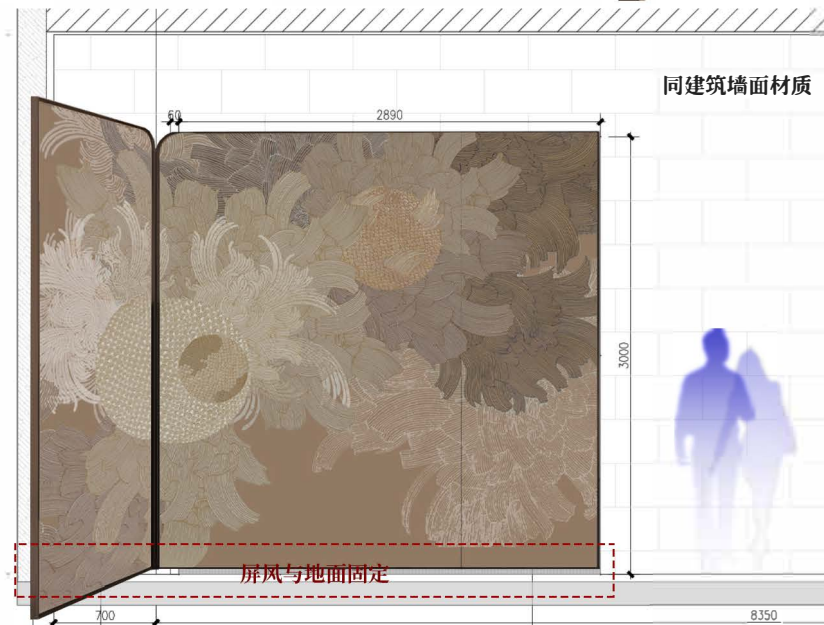
屏风底部做支撑结构与地面打螺栓固定:
