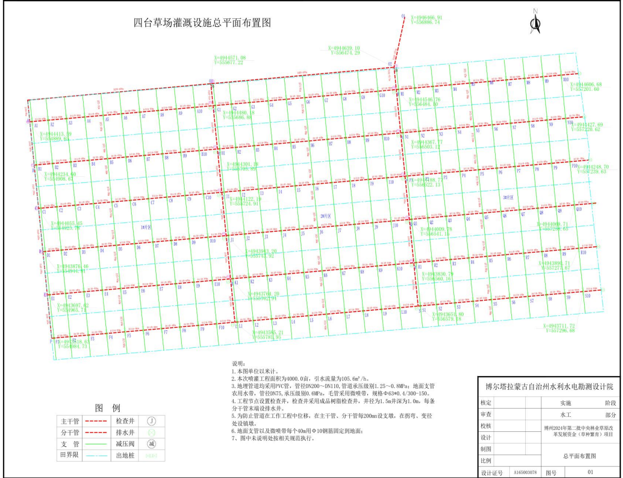
图 5-4 灌溉工程示意图
