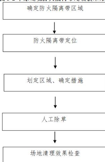
图 5-2 草原边境防火隔离带建设技术路线
