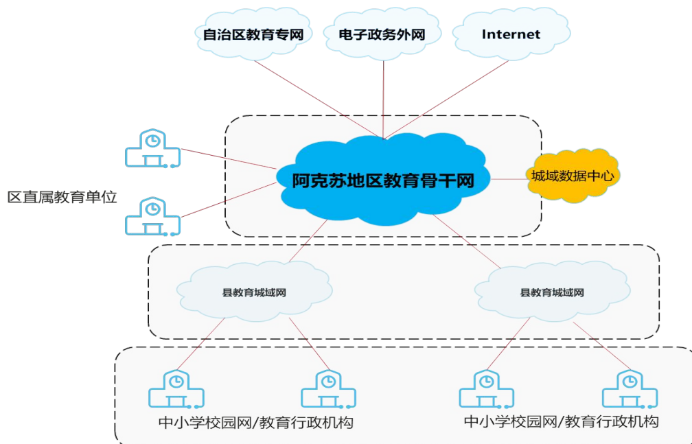
阿克苏地区教育专网目标网物理架构示意图
