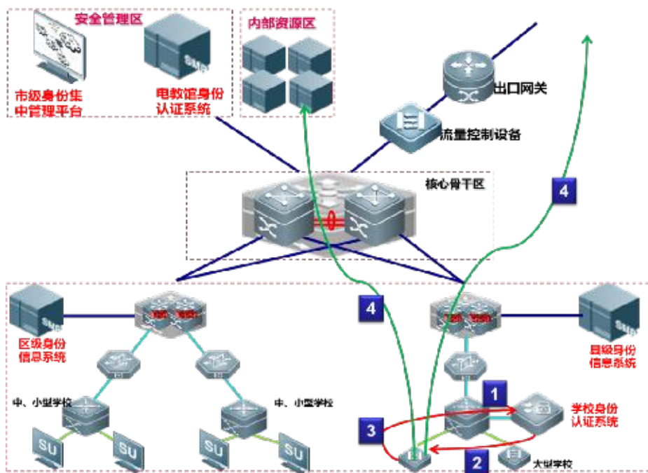
图：中小型学校到地县（市）教育局进行集中的身份认证
