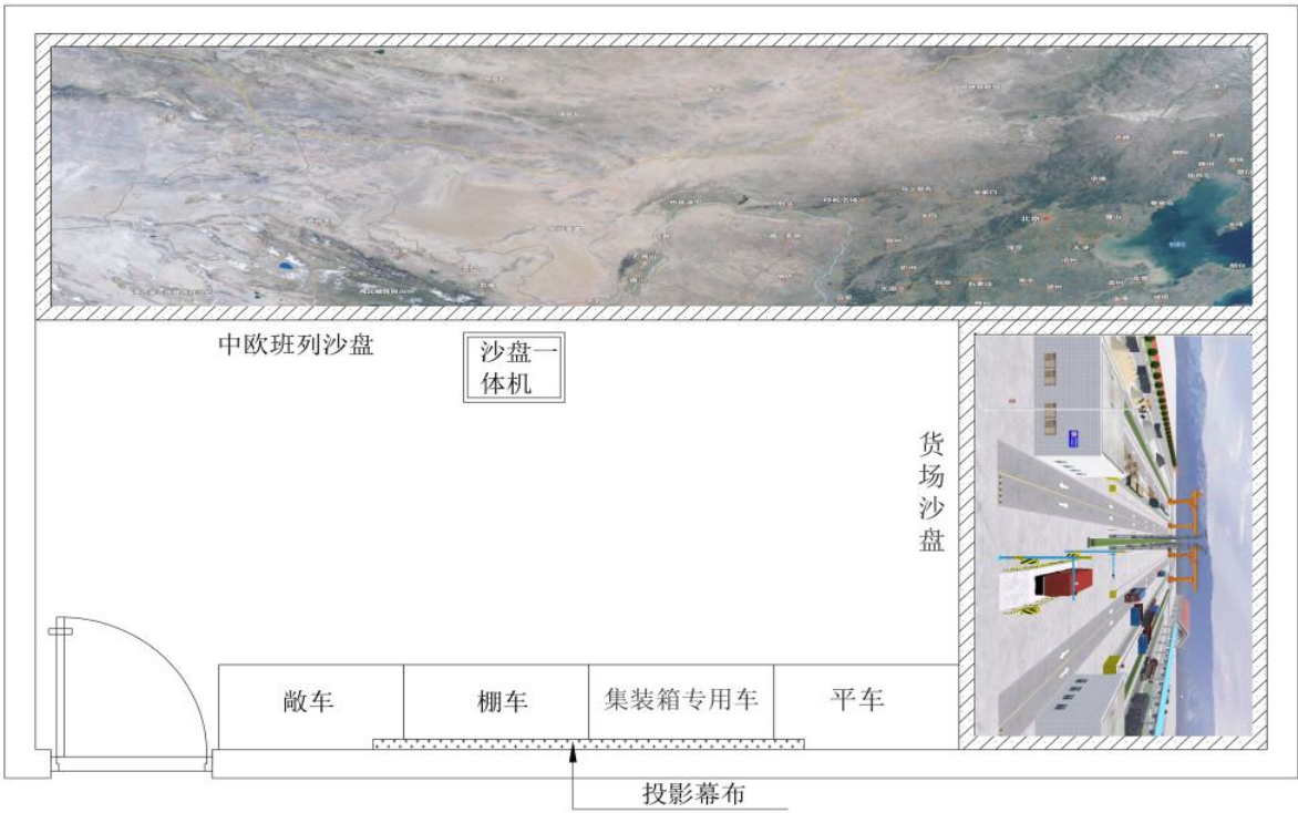
实训室布局图
