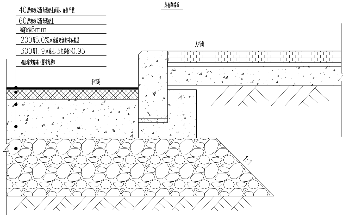
车行道路面结构图 1:20
