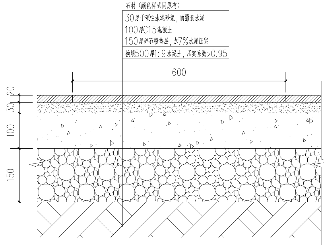
人行道铺装结构图 1:20
