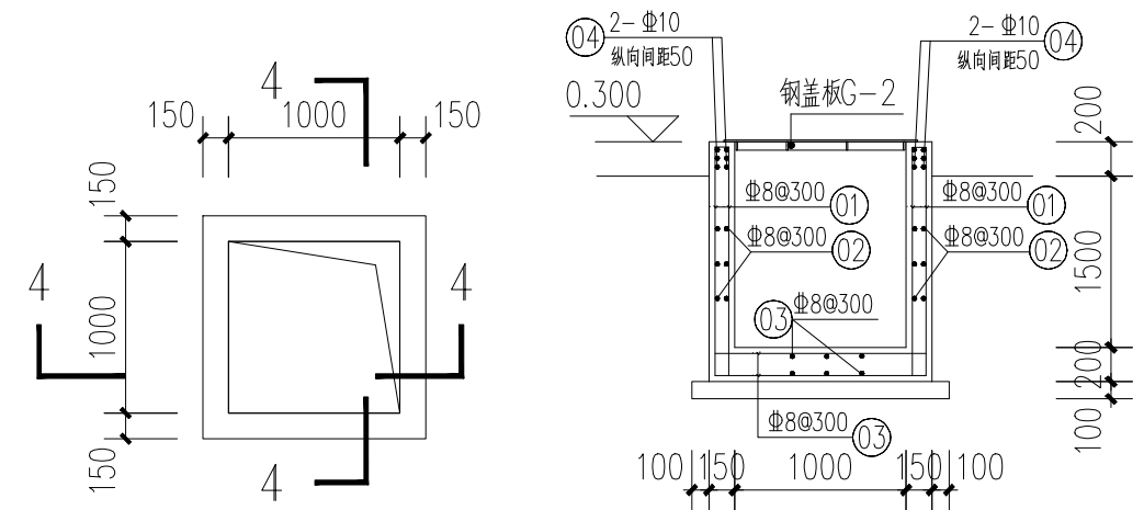
4-4 剖面及配筋图 一次性浇筑P6防渗混凝土
