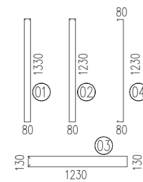
钢筋简图
