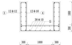
闸室配筋图 1: 50
