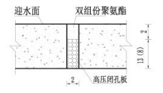
封顶板伸缩缝大样
