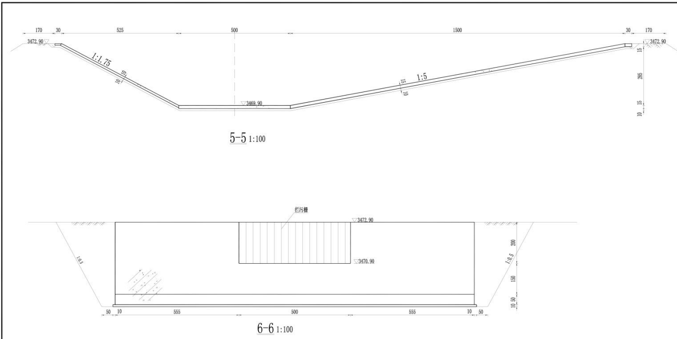
边坡与压顶结构缝大样
