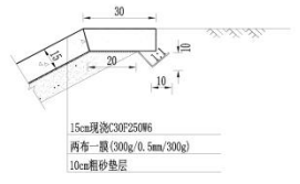
清淤通道出口大样 1:20
