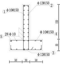
隔墙3-3断面墙配筋图 1:50
