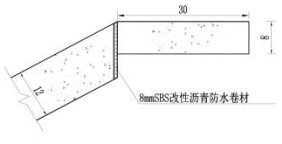
边坡与压顶结构缝大样
