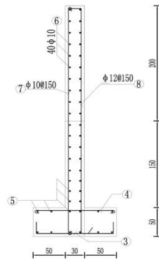
隔墙4-4断面墙配筋图 1:50
