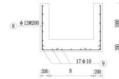
分水闸后矩形渠配筋图 1: 50
