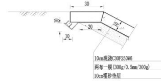
压顶大样 1:20
