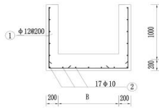
闸前矩形渠配筋图 1: 50
