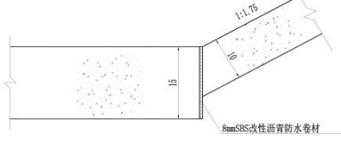
边坡、底板结构缝大样
