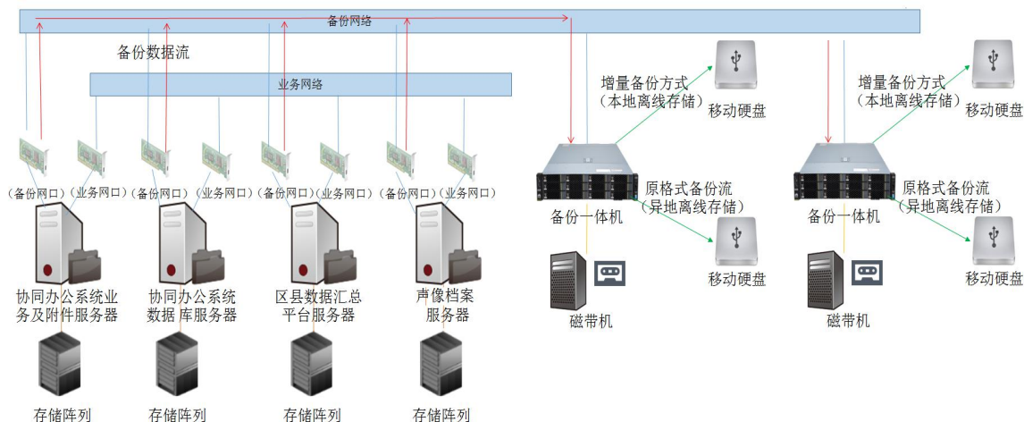
图备份系统逻辑架构图
