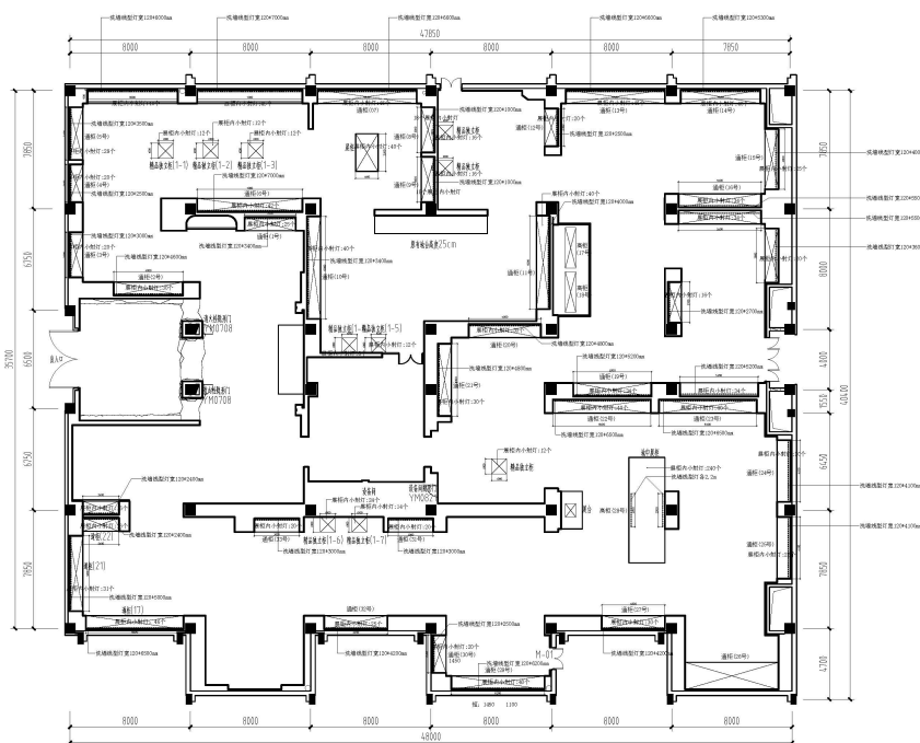
平面布置图
