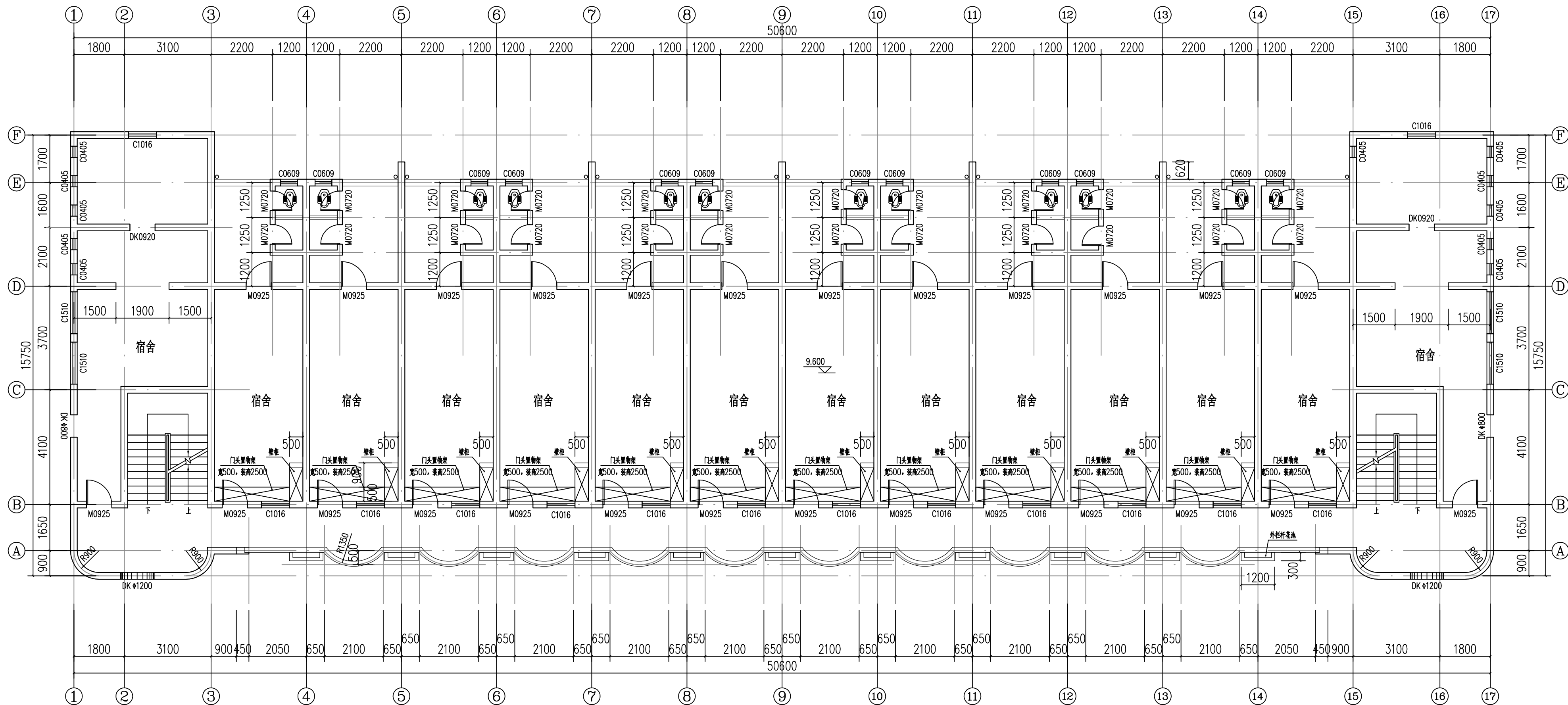
四层平面图 1:125
