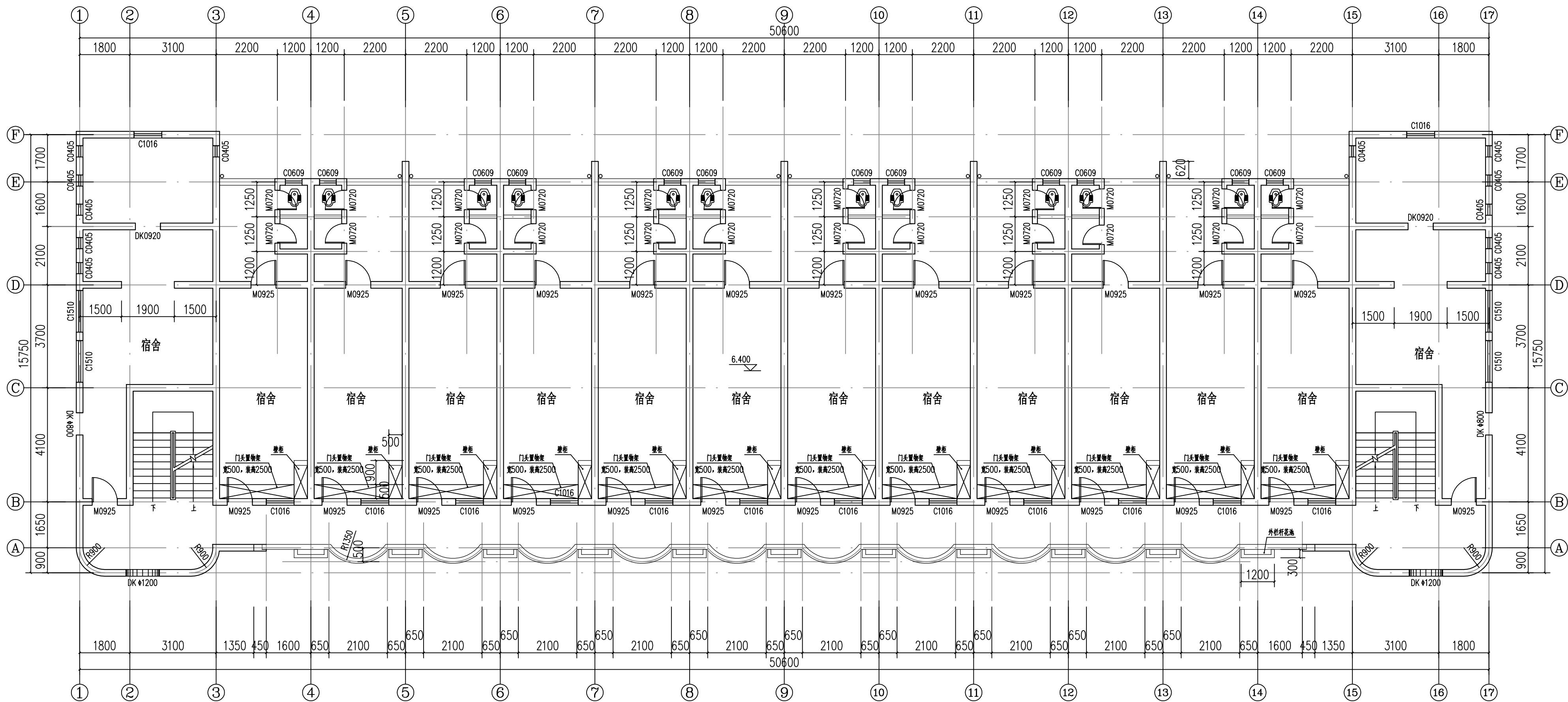
三层平面图 1:125
