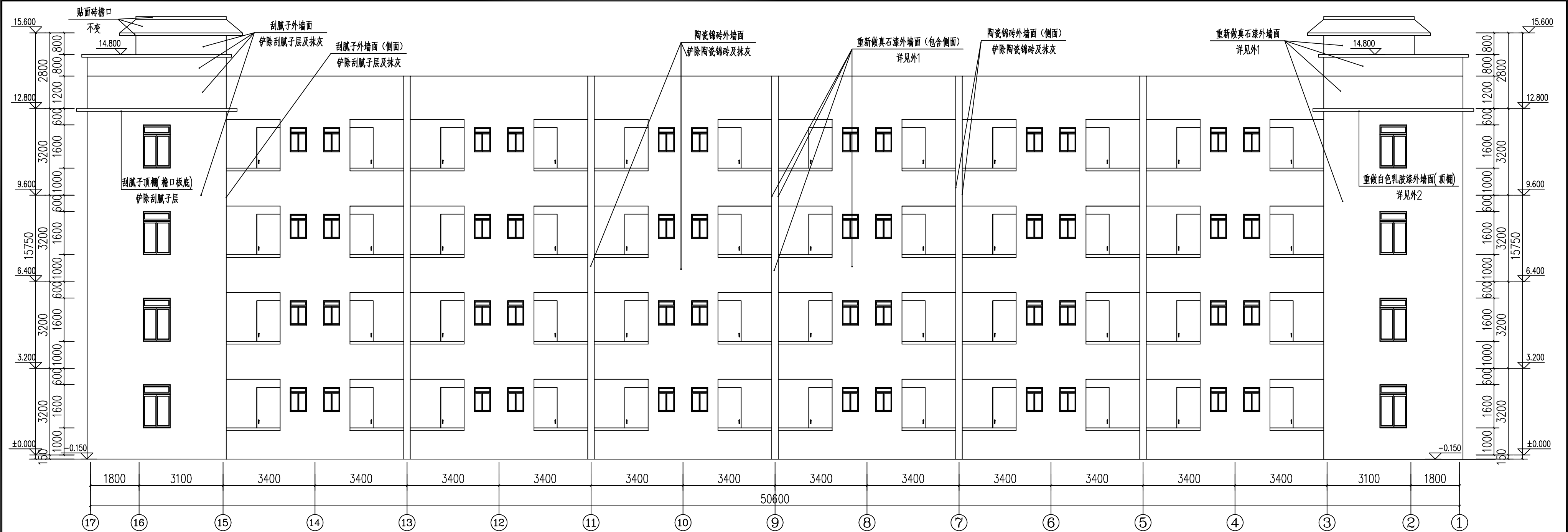
17~1轴背立面图 1:125
