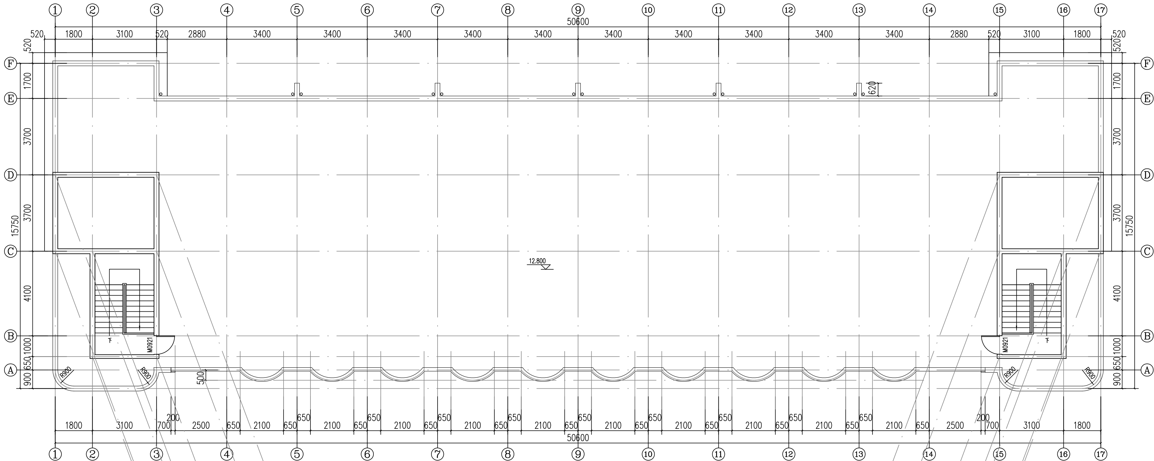
屋面层平面图 1:125
