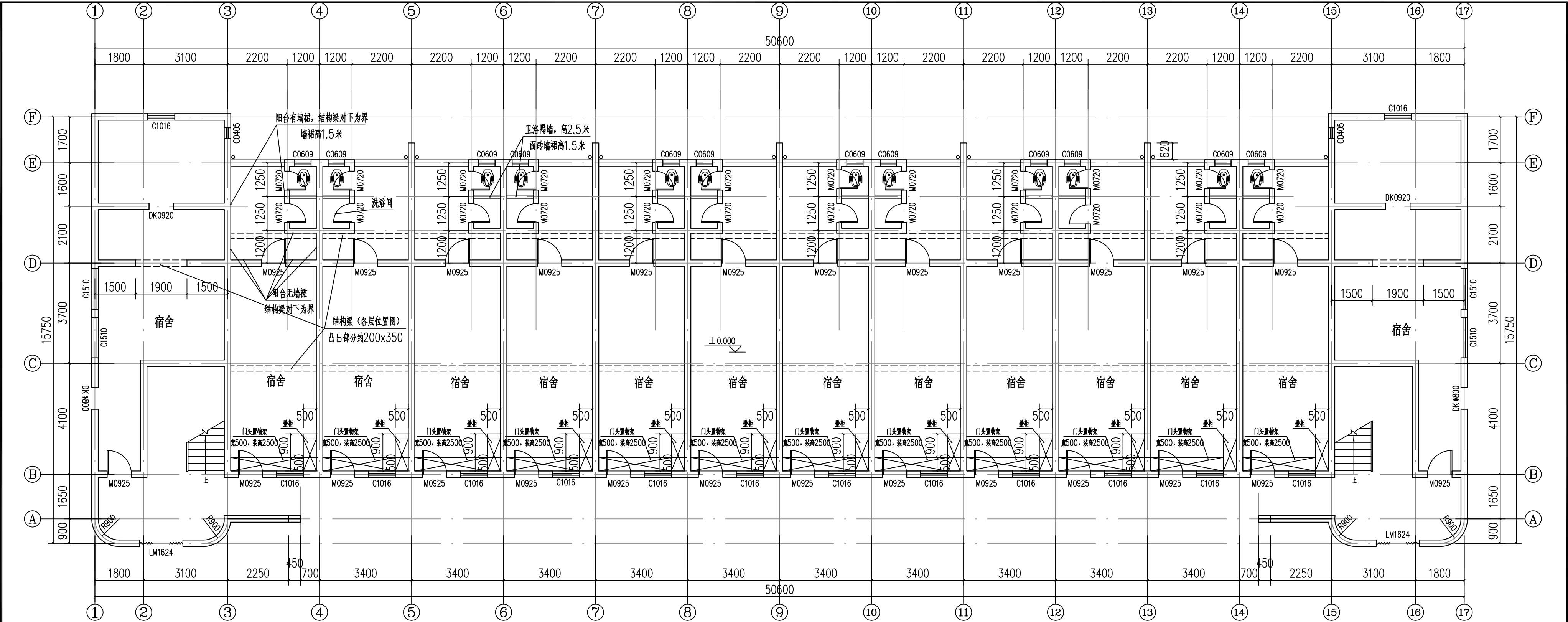
一层平面图 1:125
