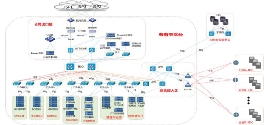
图 2 互联网商用云平台网络架构图
