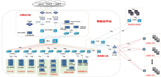
图 2 互联网商用云平台网络架构图
