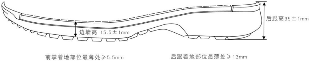
鞋底尺寸示意图
