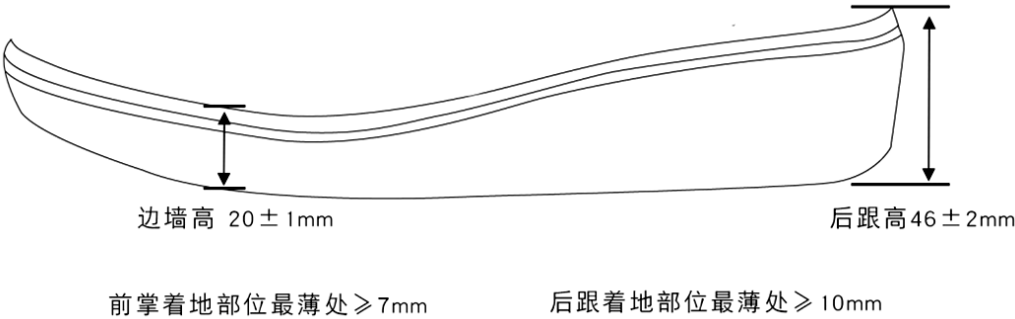
鞋底尺寸示意图
