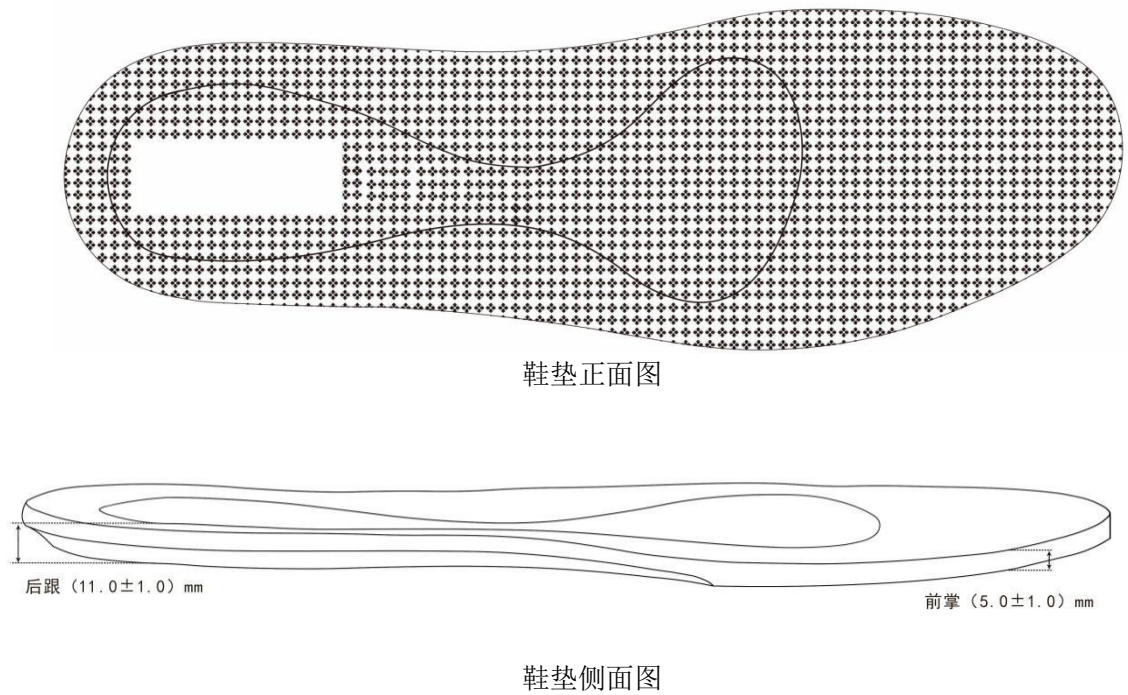
图 2.1 成型鞋垫样式
