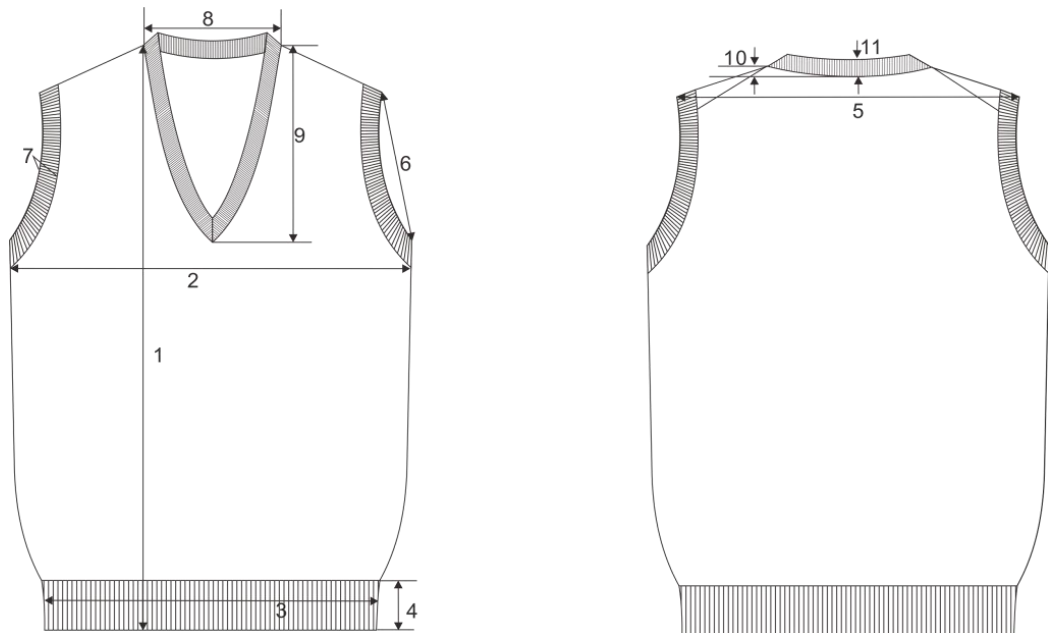
图3 男V领羊毛套头背心测量位置
