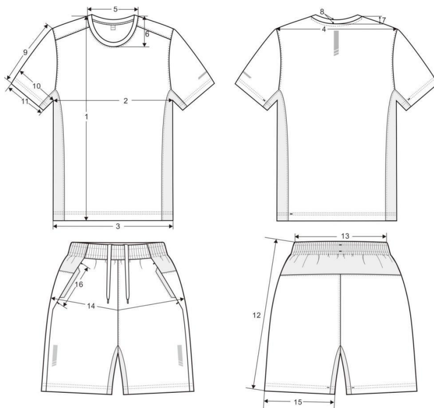
图 3 男夏体能训练服尺寸测量位置
