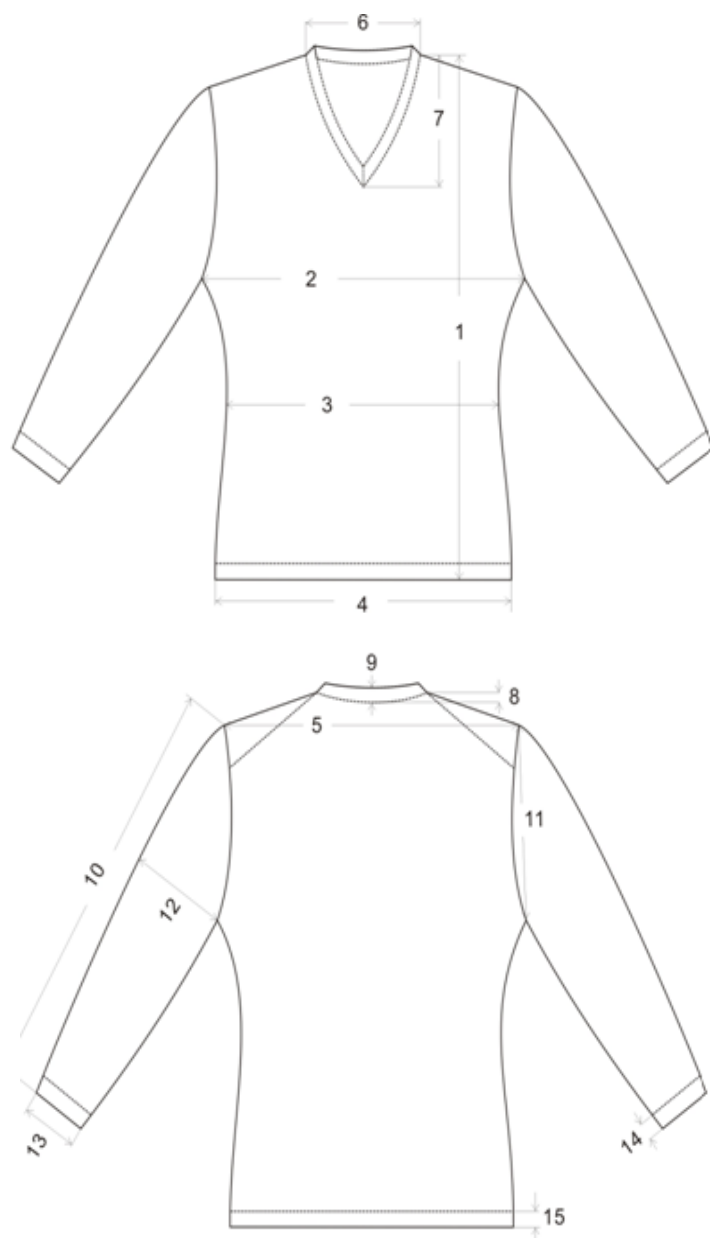
女 V 领保暖内衣测量图
