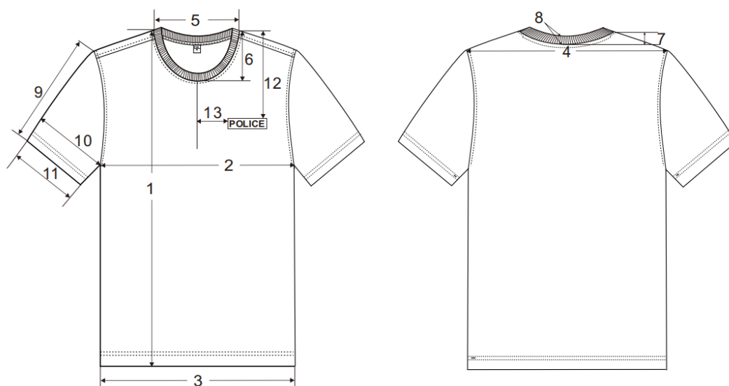
图 3 男圆领短袖棉 T 恤尺寸测量位置
