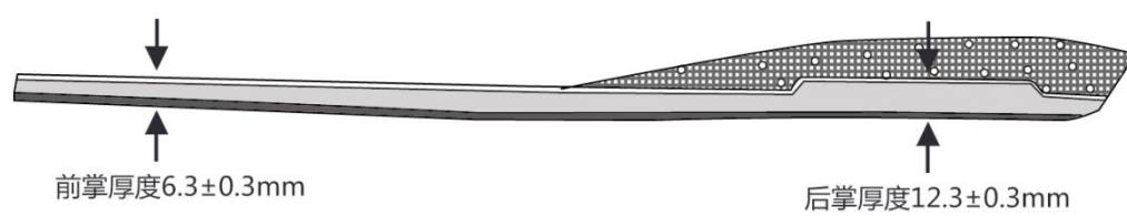
鞋垫尺寸示意图
