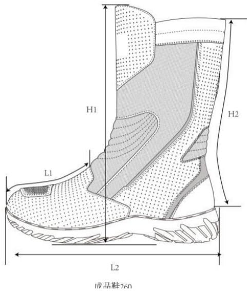
成品靴测量尺寸部位
