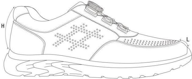
图 3 执勤凉鞋测量部位
