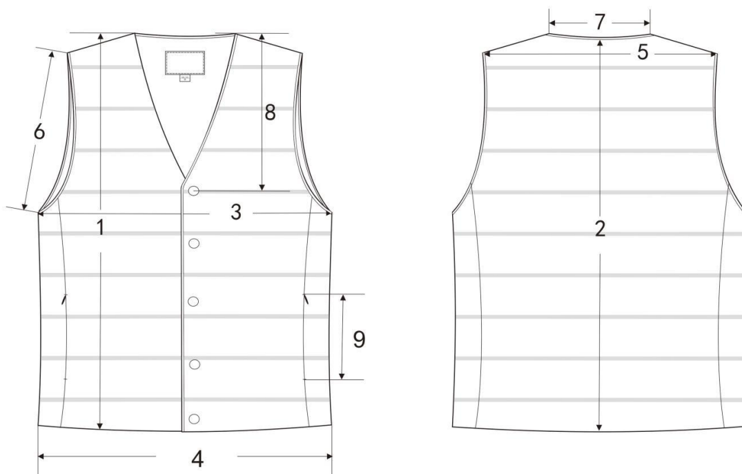
图3 男羽绒背心尺寸测量位置
