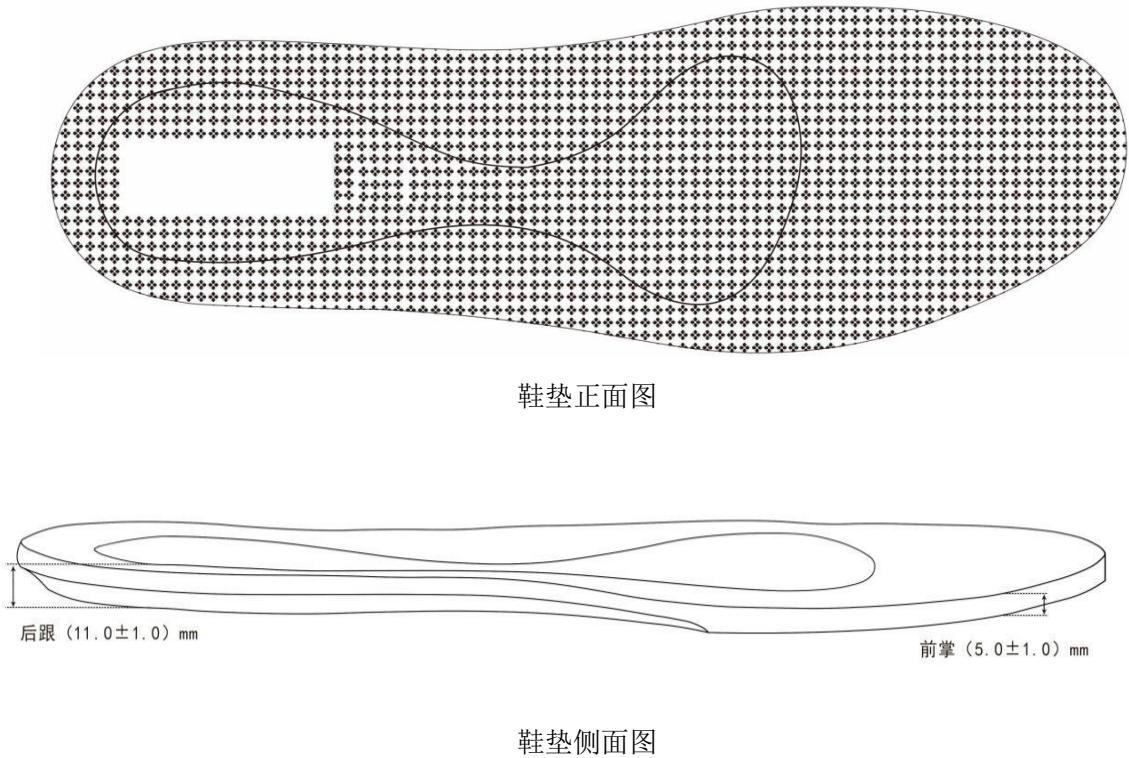
图 2.1 成型鞋垫样式
