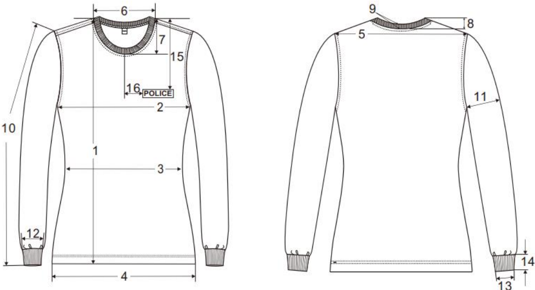
图 4 女圆领长袖棉 T 恤尺寸测量位置
