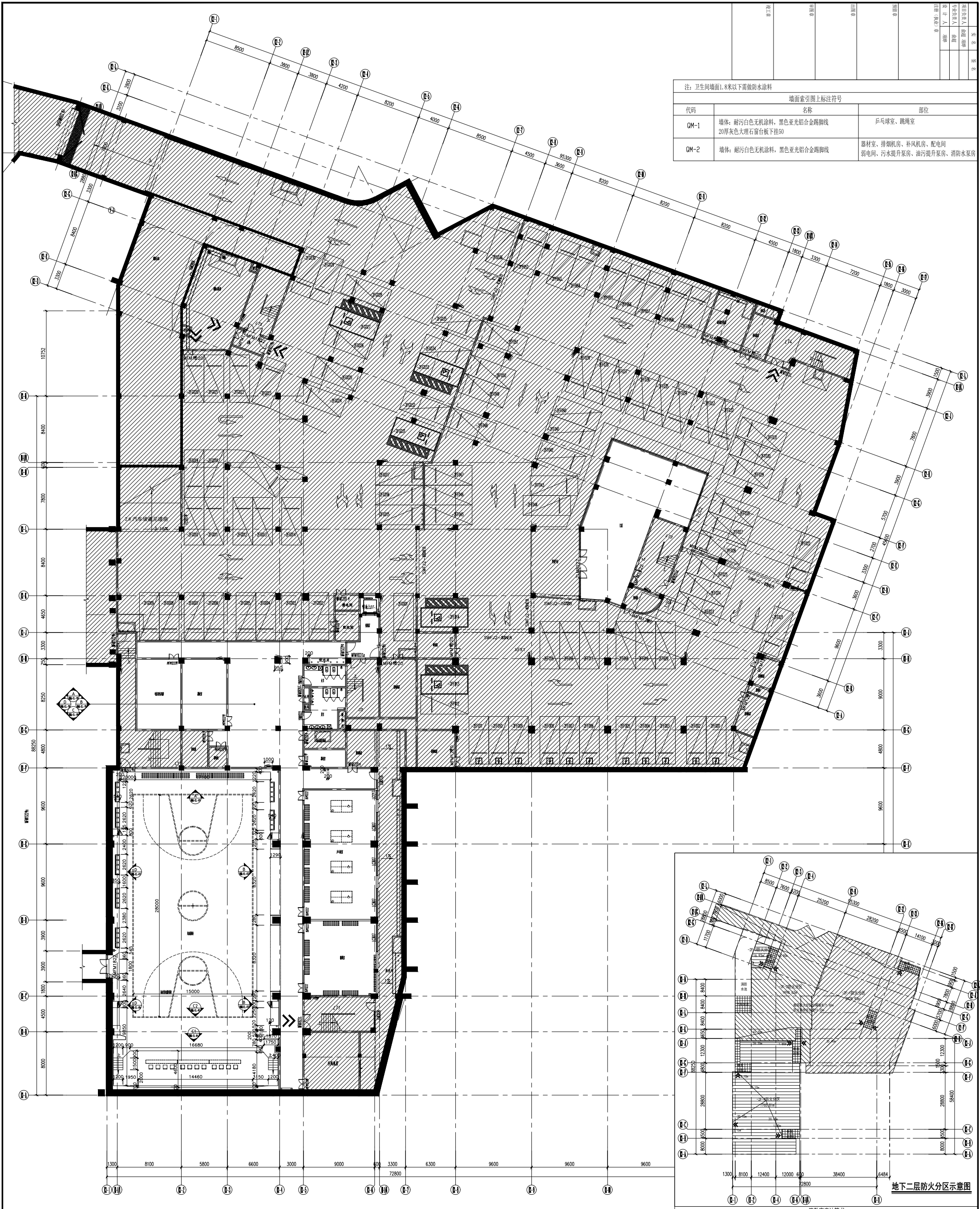
地下二层平面布置图 FIXTURE & FURNISHING PLAN SCALE 1:150
