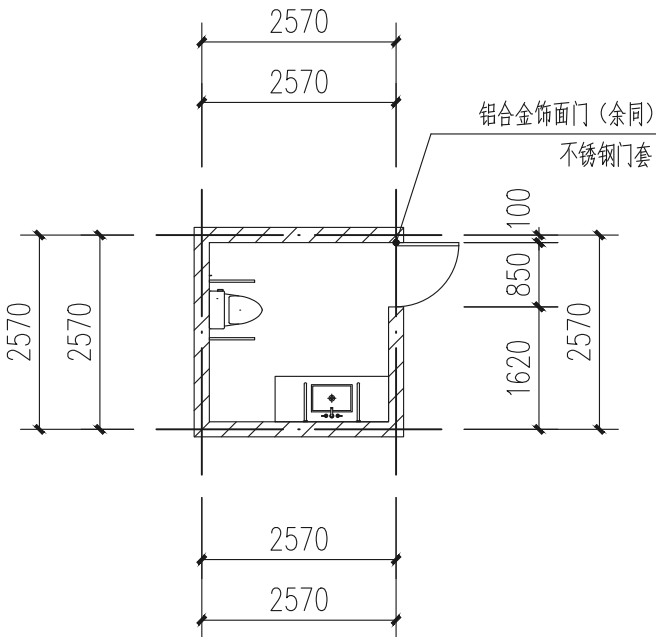
残疾人卫生间 1:100
