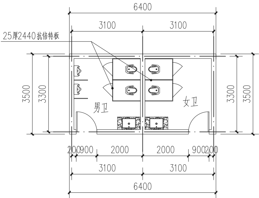
南门传达室平面图 1:100
