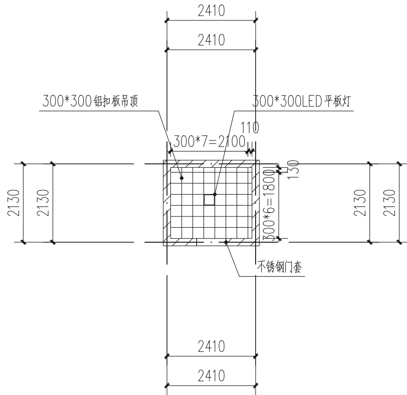
科技中心茶水间 1:100
