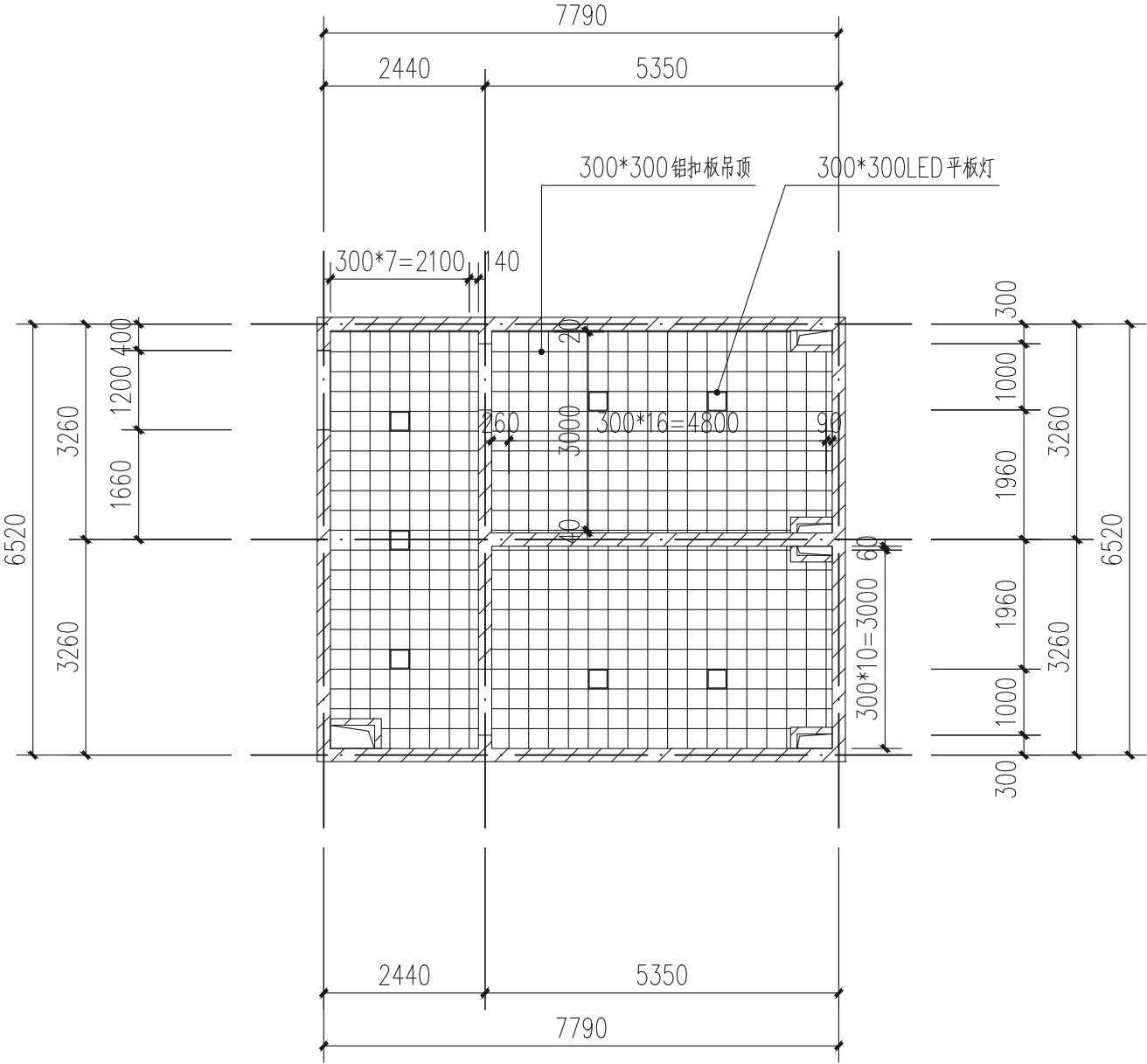
求是南楼、求是中楼、求是北楼卫生间天花平面图 1:100
