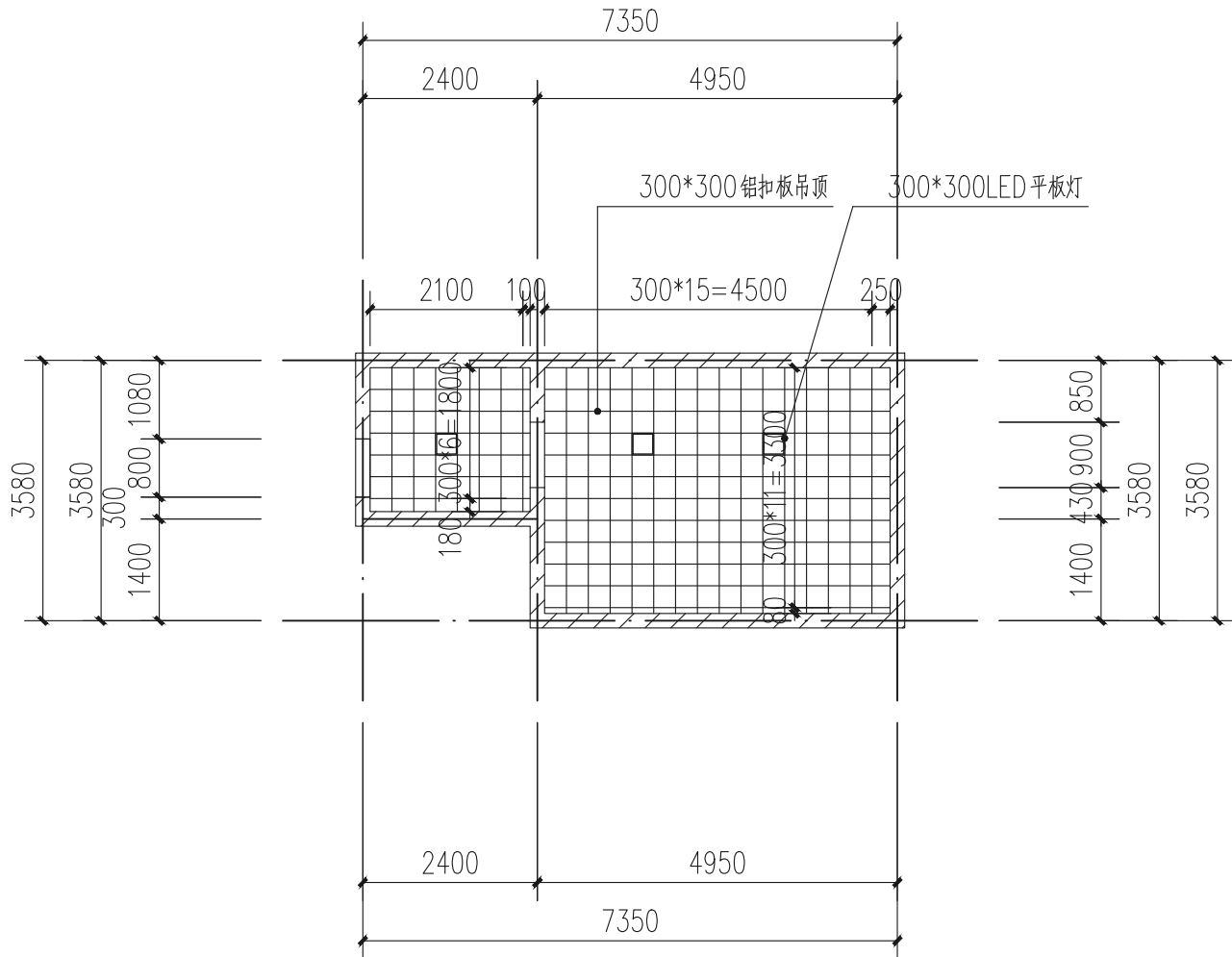
科技中心(男卫)卫生间天花平面图 1:100
