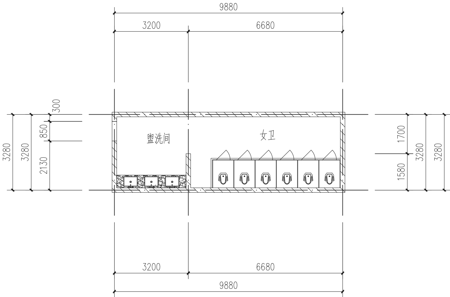
方正楼（女卫）卫生间 1:100 块料墙面破损处局部更换、地砖破损处局部更换
