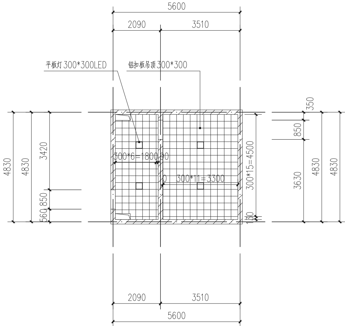
工训中心(女卫)卫生间天花平面图 1:100
