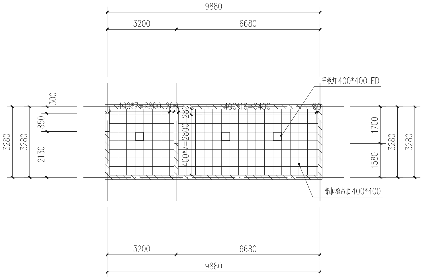
方正楼（女卫）卫生间天花平面图 1:100 注：1、原吊顶拆除，用400X400 铝扣板吊顶换新 2、原吸顶灯拆除，用400X400led平板灯换新
