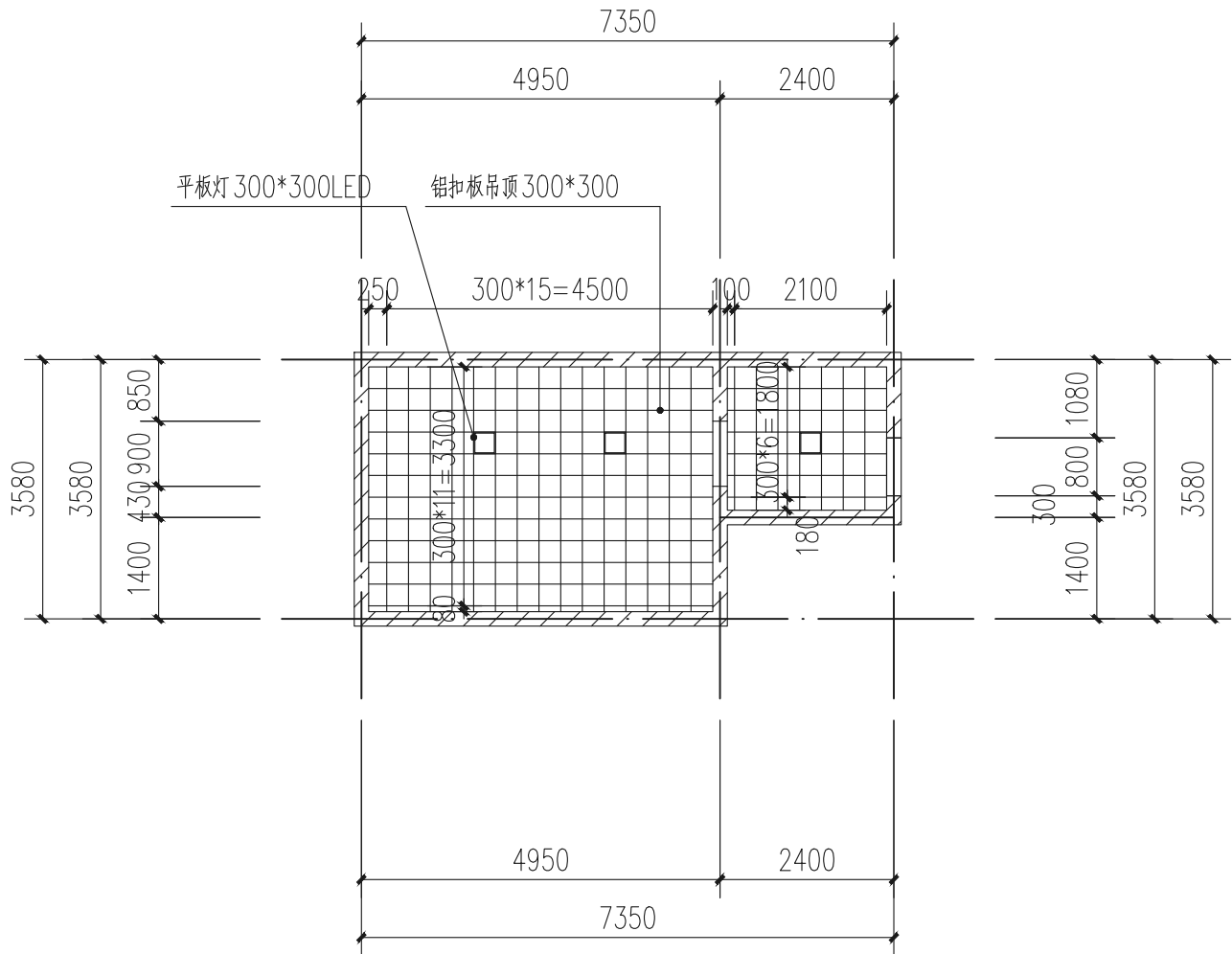
科技中心（女卫）卫生间天花平面图 1:100
