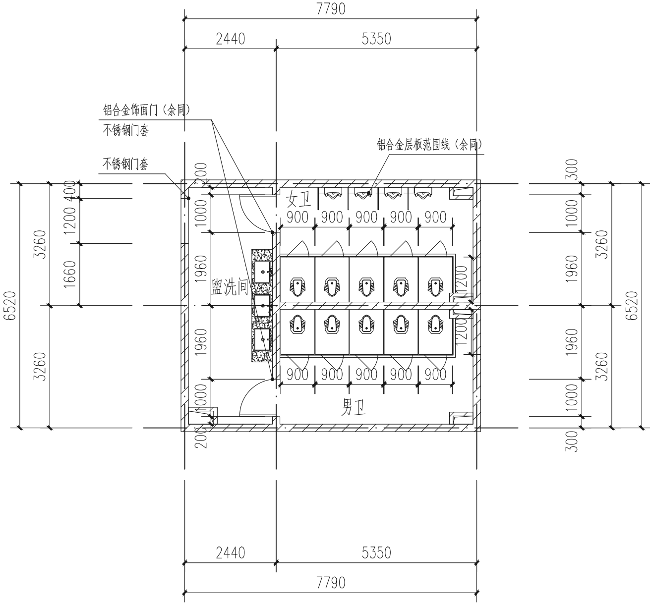
求是南楼、求是中楼、求是北楼卫生间 1:100
