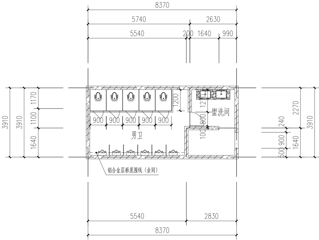
明德北楼（男卫）卫生间 1:100 注：明德南、北楼相同。
