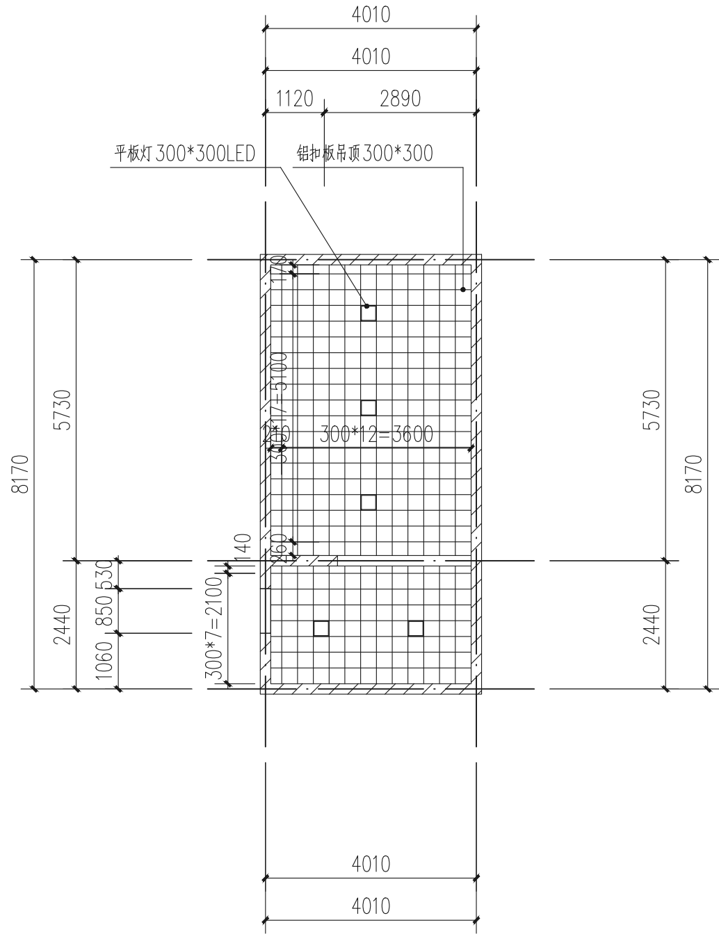
仰仪中楼、仰仪北楼（女卫）卫生间天花平面图 1:100
