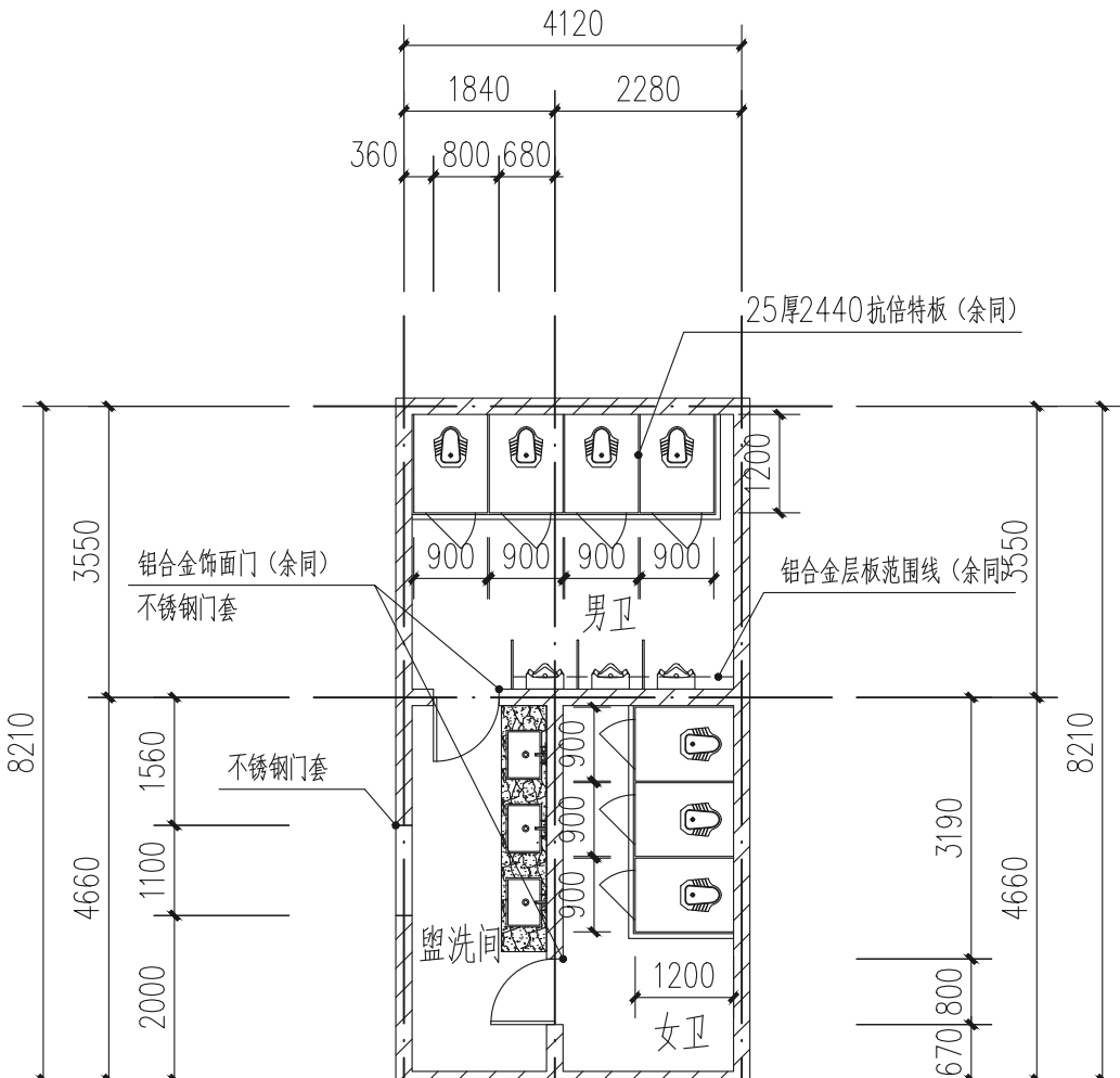
校医院卫生间 1:100
