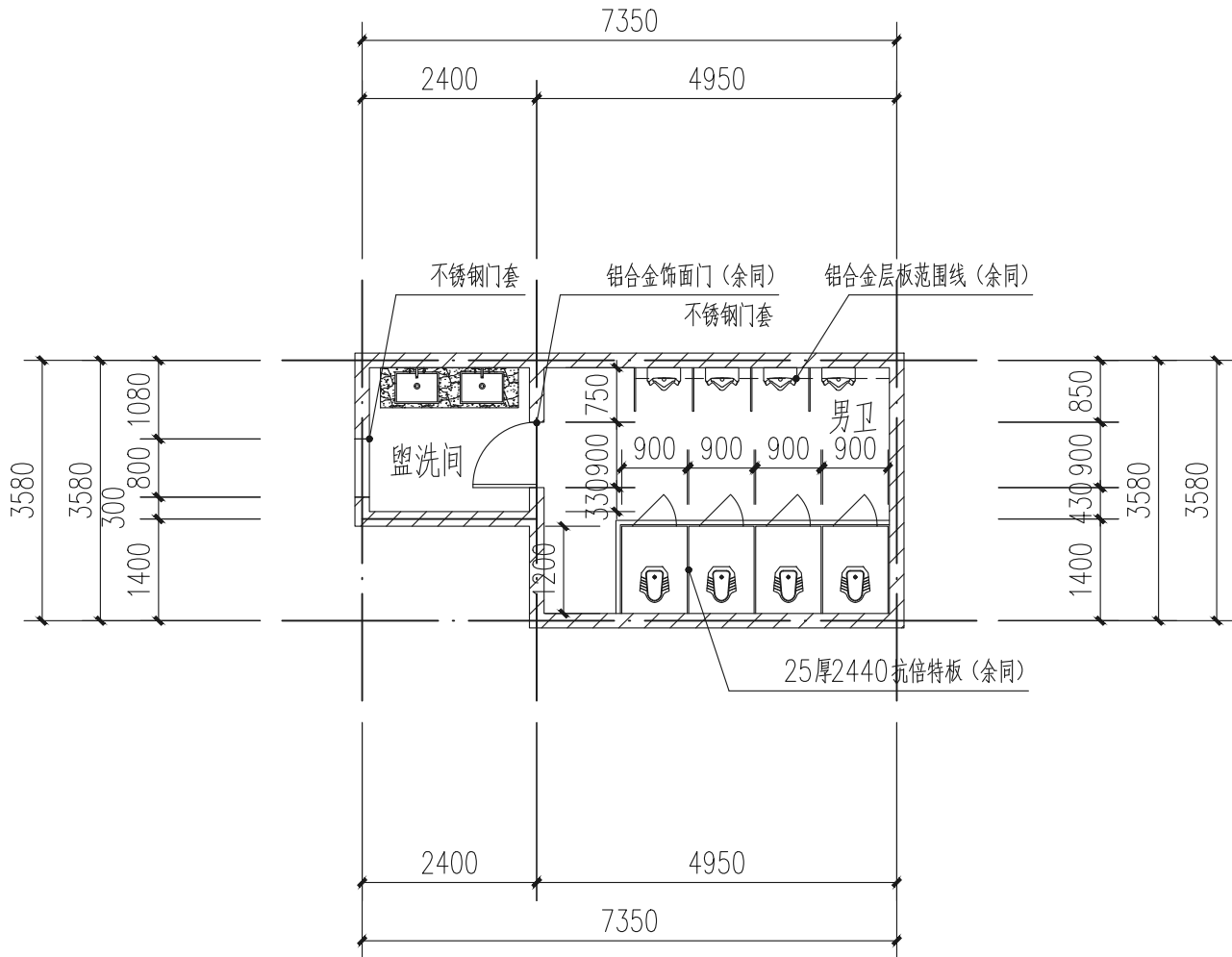
科技中心(男卫)卫生间 1:100
