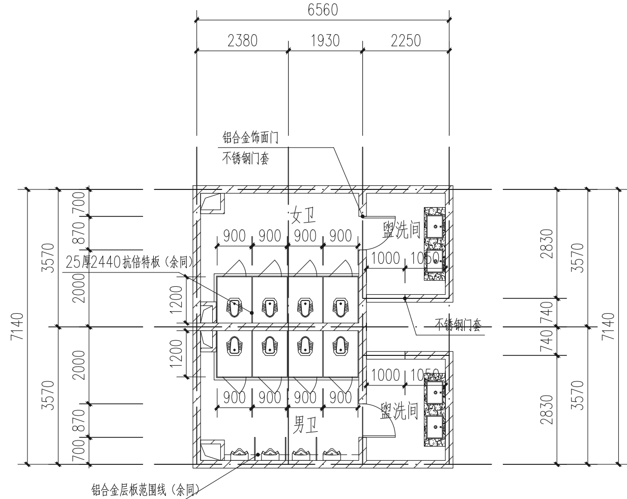
方圆南楼卫生间 1:100
