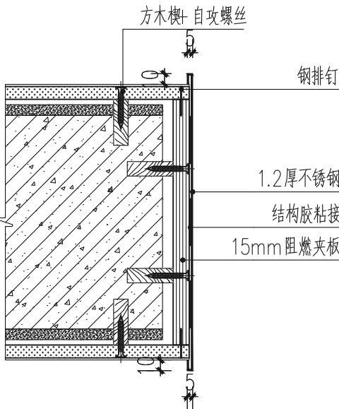
不锈钢门套节点图 1:50
