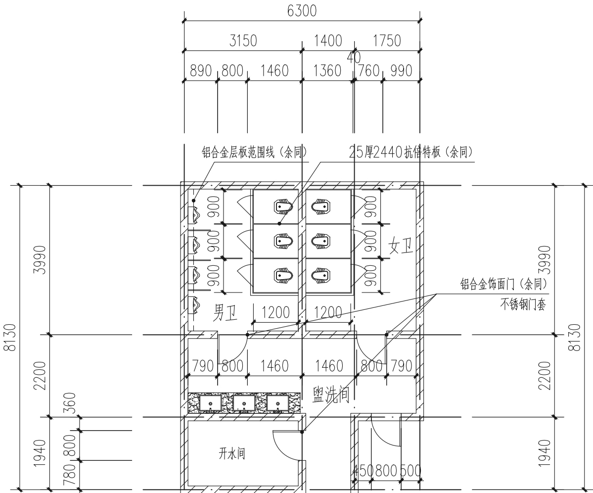
活动中心卫生间 1:100
