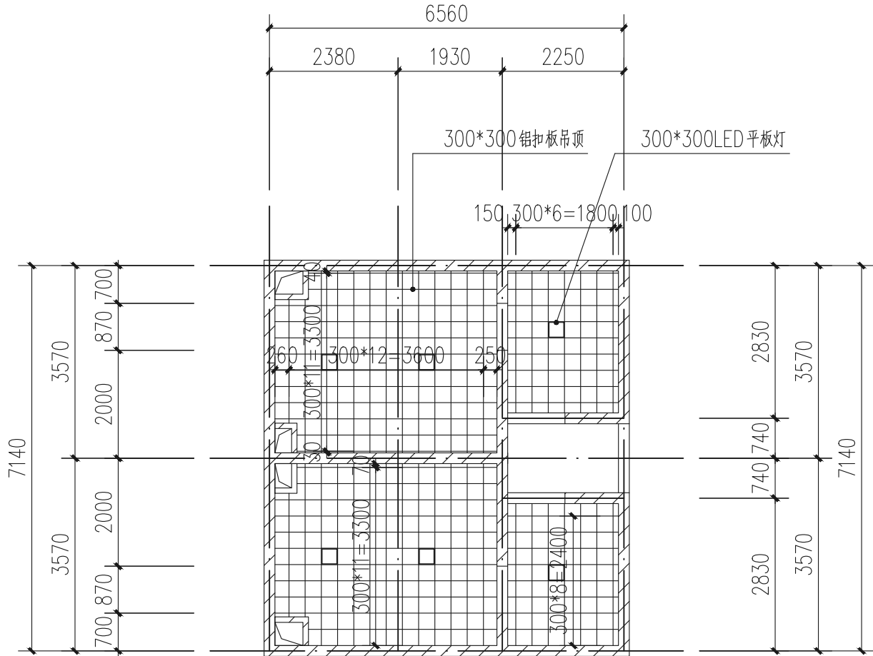
方圆南楼卫生间天花平面图 1:100
