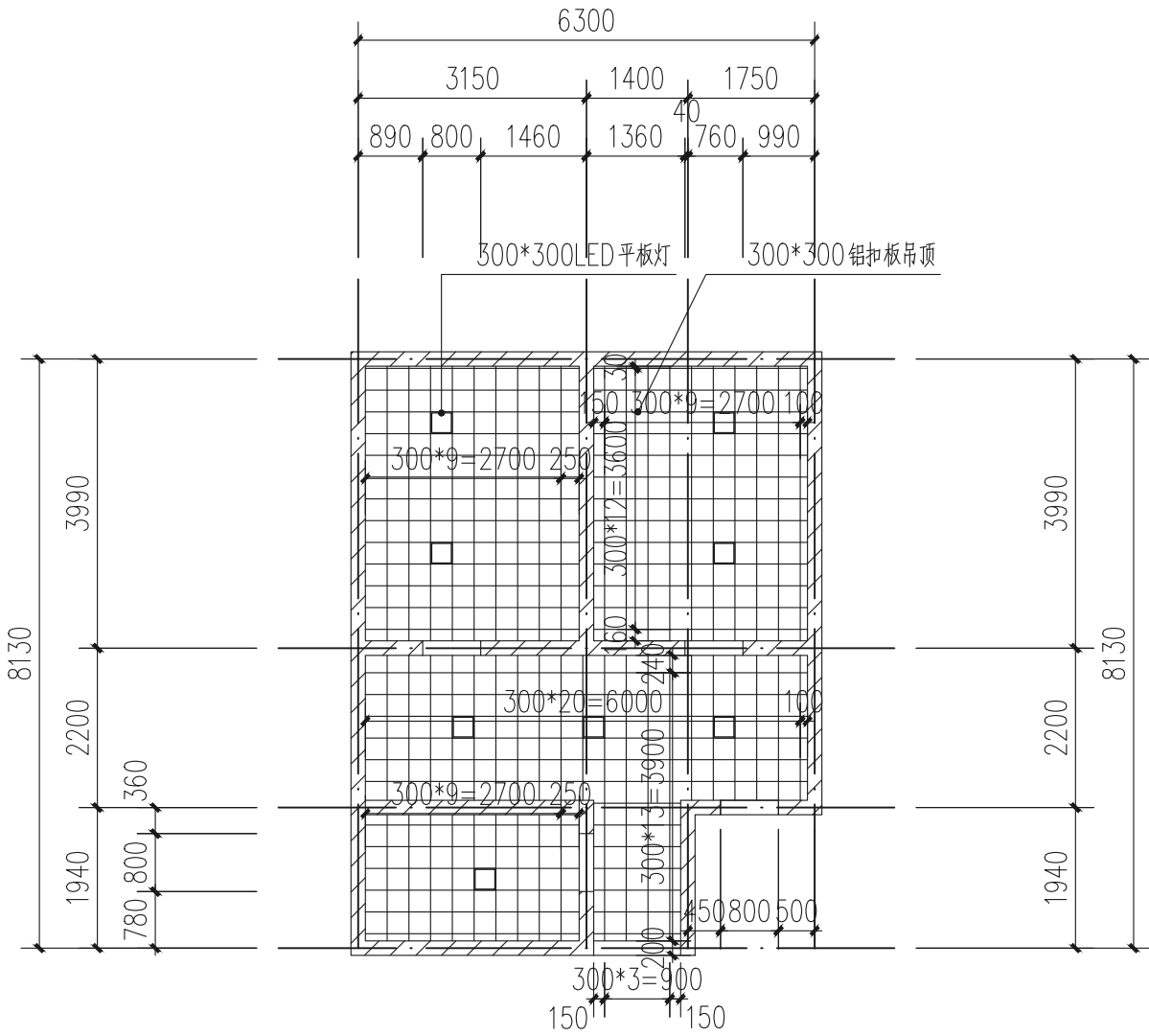
活动中心卫生间天花平面图 1:100
