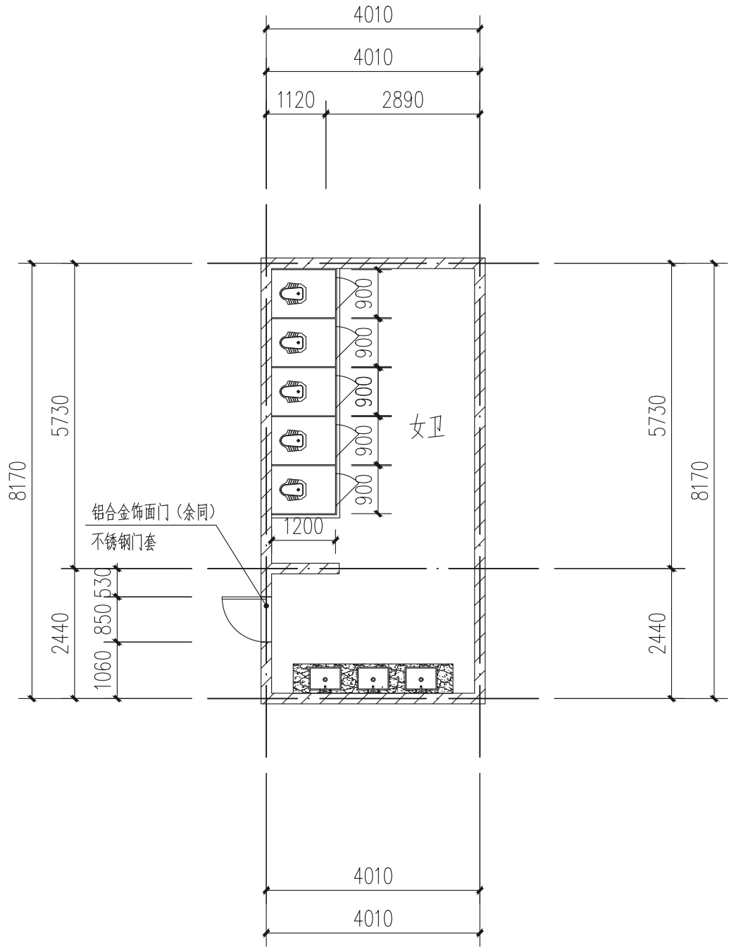
仰仪中楼、仰仪北楼（女卫）卫生间 1:100
