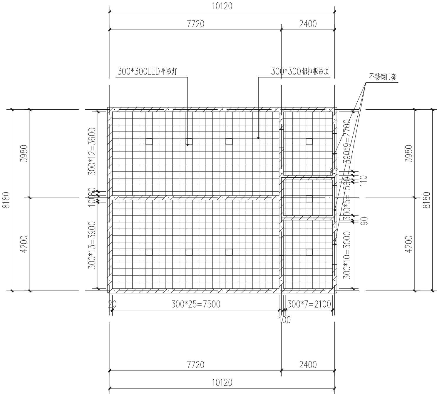
赛博北楼、赛博南楼标准层卫生间天花平面图 1:100
