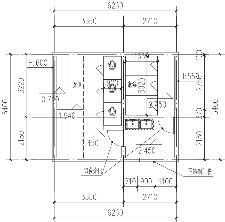
球场东女卫生间平面图 1:100
