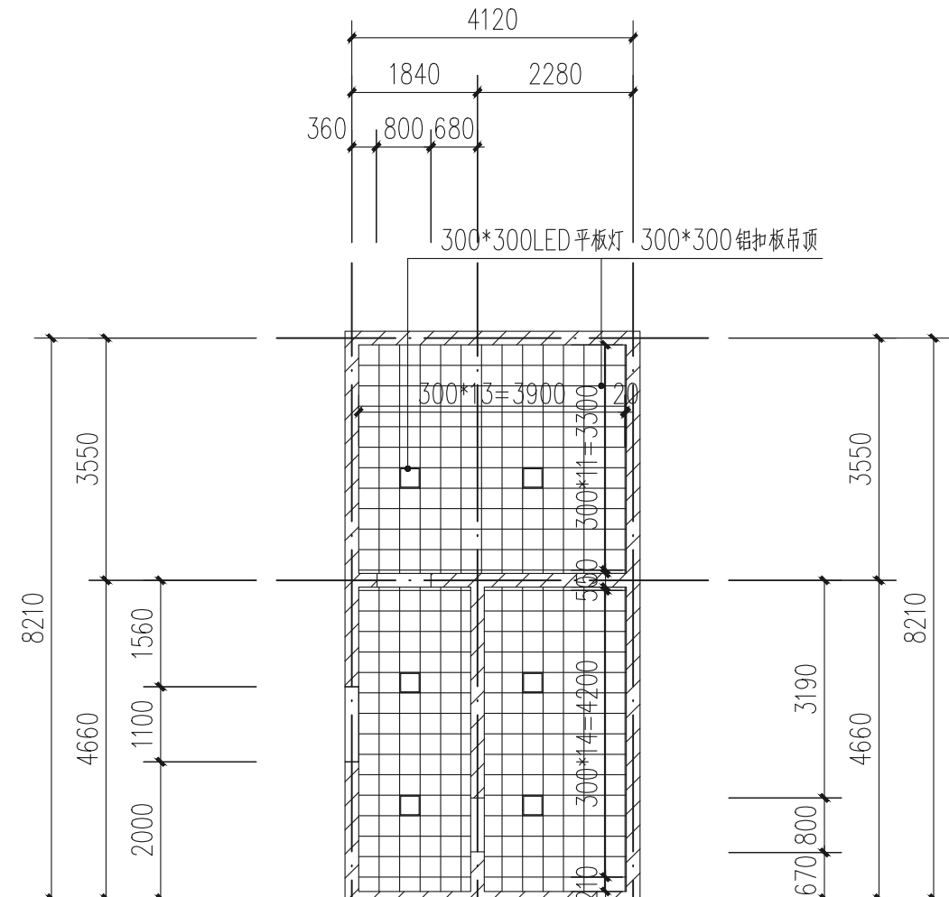
校医院卫生间天花平面图 1:100
