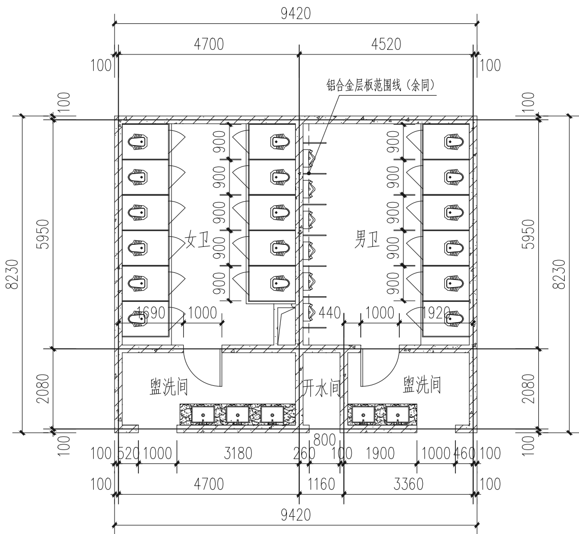
广宇楼C座平面图 1:100
