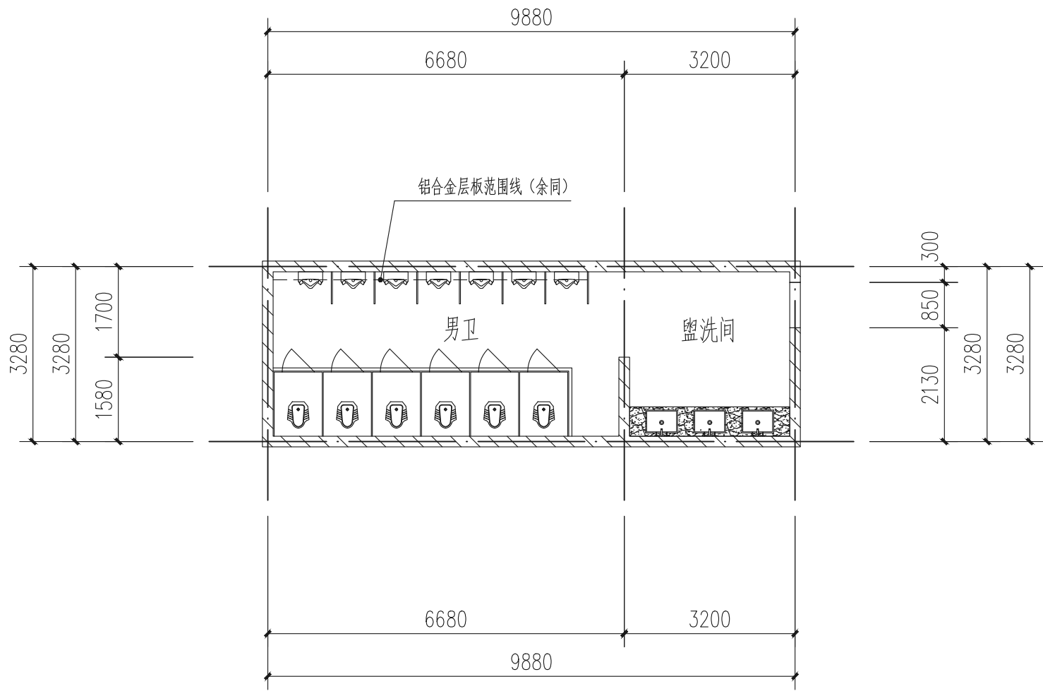
方正楼（男卫）卫生间 1:100
