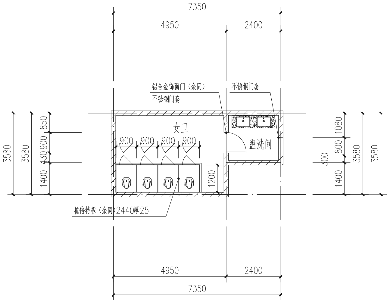
科技中心（女卫）卫生间 1:100
