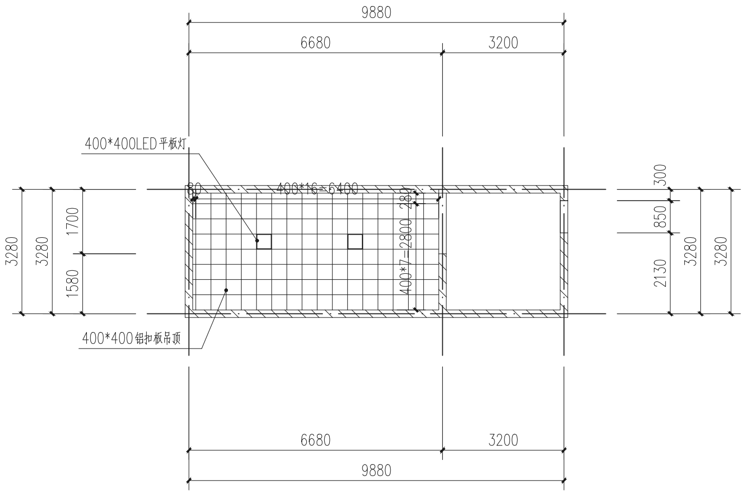
方正楼（男卫）卫生间天花平面图 1:100
