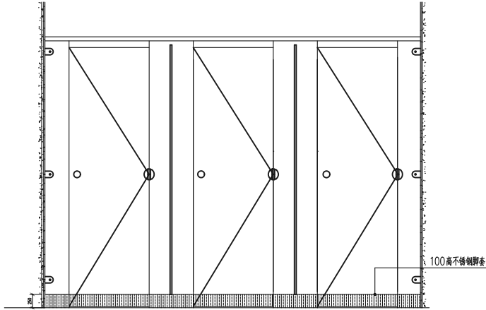
卫生间隔断示意图 1:50
