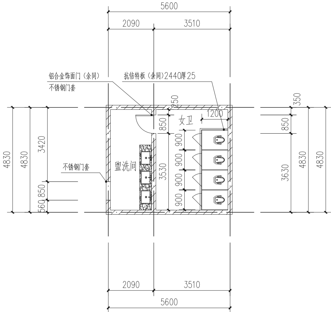
工训中心(女卫)卫生间 1:100
