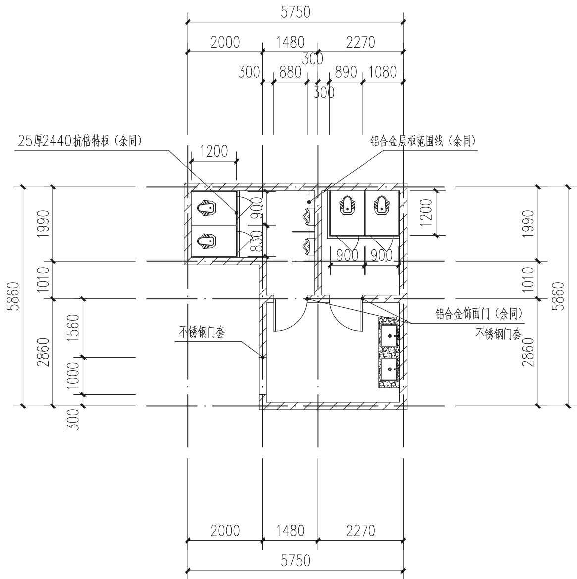
收发室卫生间 1:100
