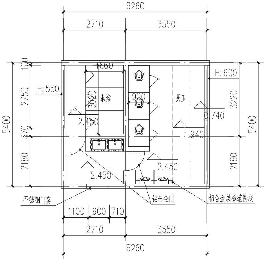
球场东男卫生间平面图 1:100
