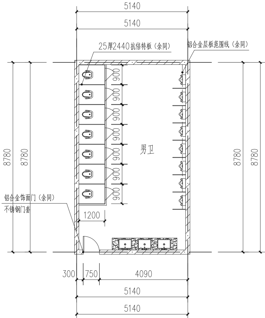
球场西男卫生间2 1:100
