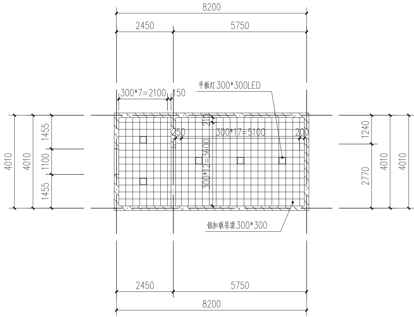
仰仪南楼（女卫）卫生间天花平面图 1:100
