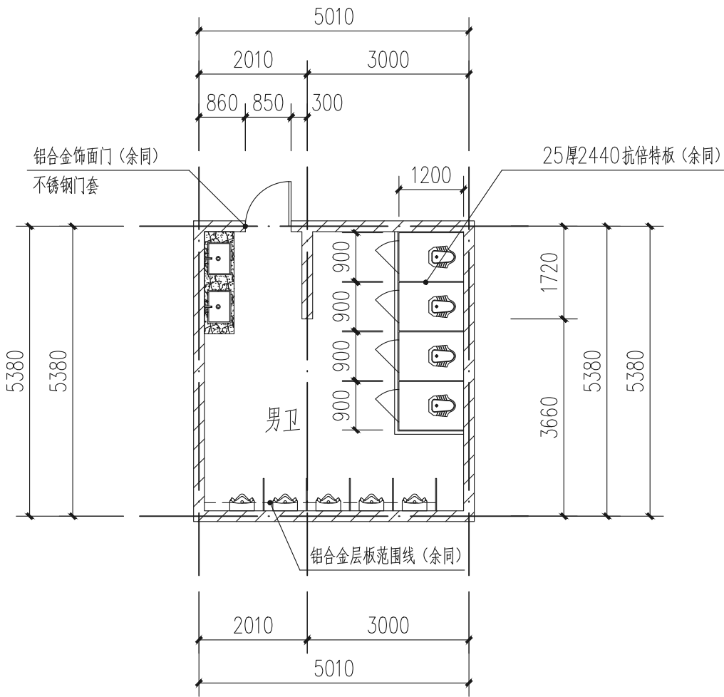
球场西男卫生间1 1:100
