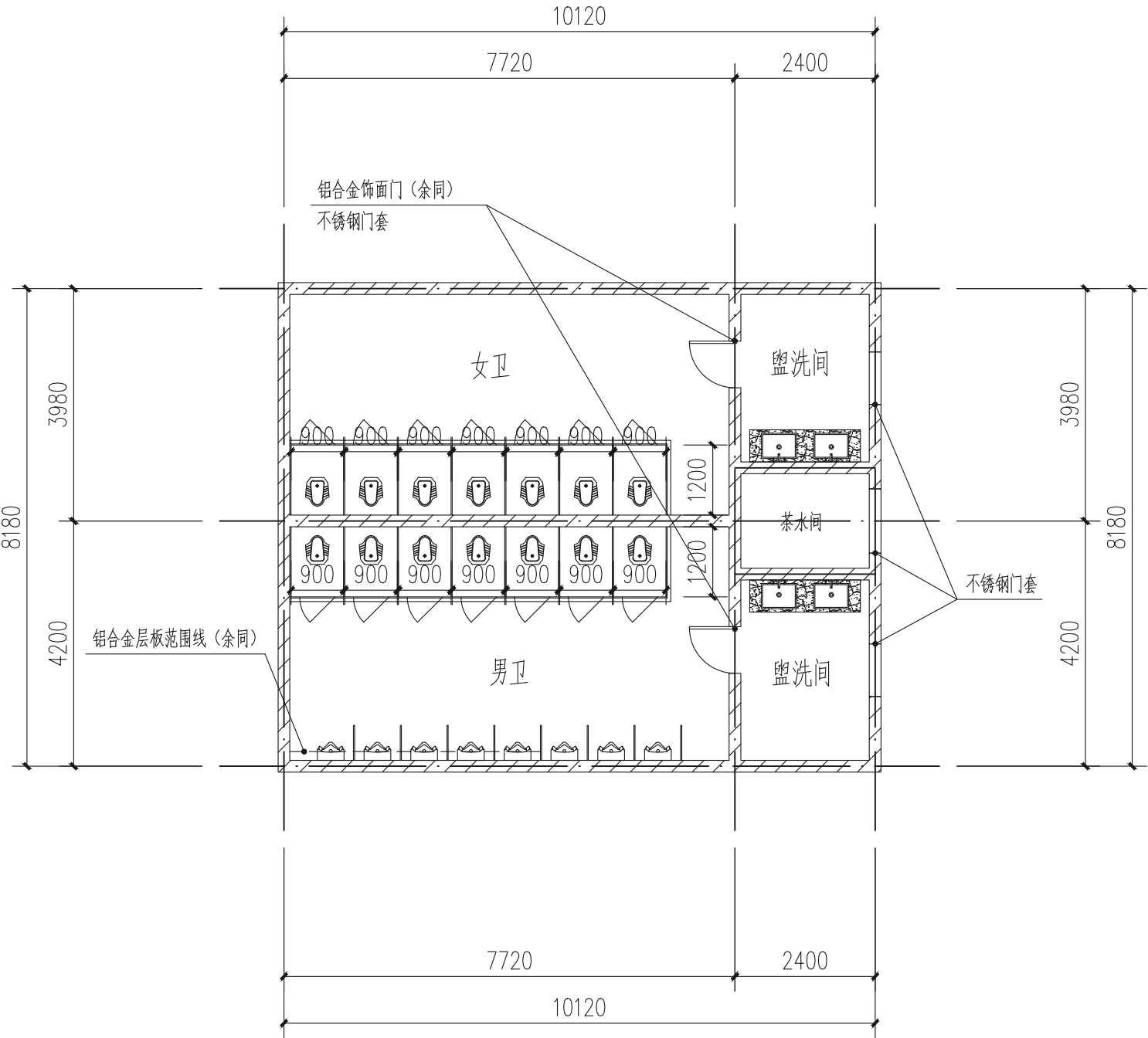
赛博北楼、赛博南楼标准层卫生间 1:100
