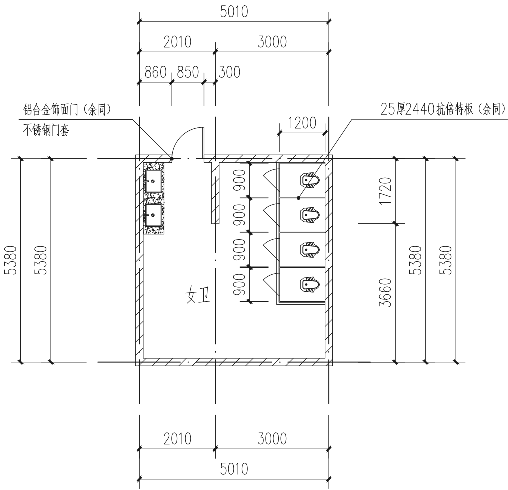
球场西女卫生间1 1:100
