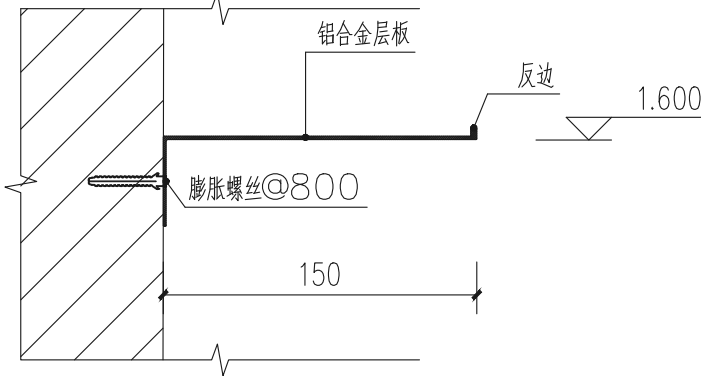
铝合金层板大样图 1:50
