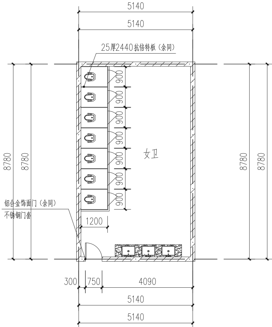
球场西女卫生间2 1:100
