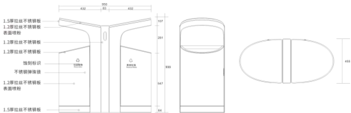
图 1 主干道次干道果屑箱尺寸
