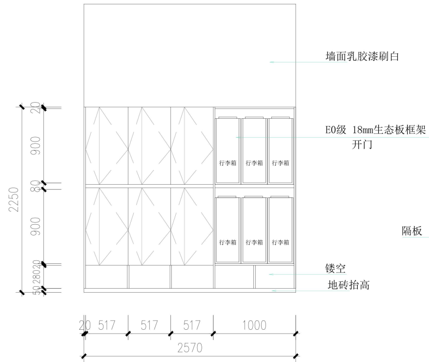
6人宿舍 衣柜立面图
