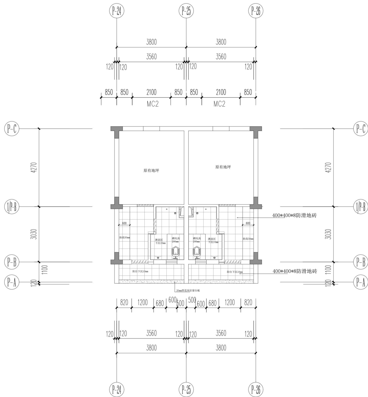
宿舍地面铺装平面图
