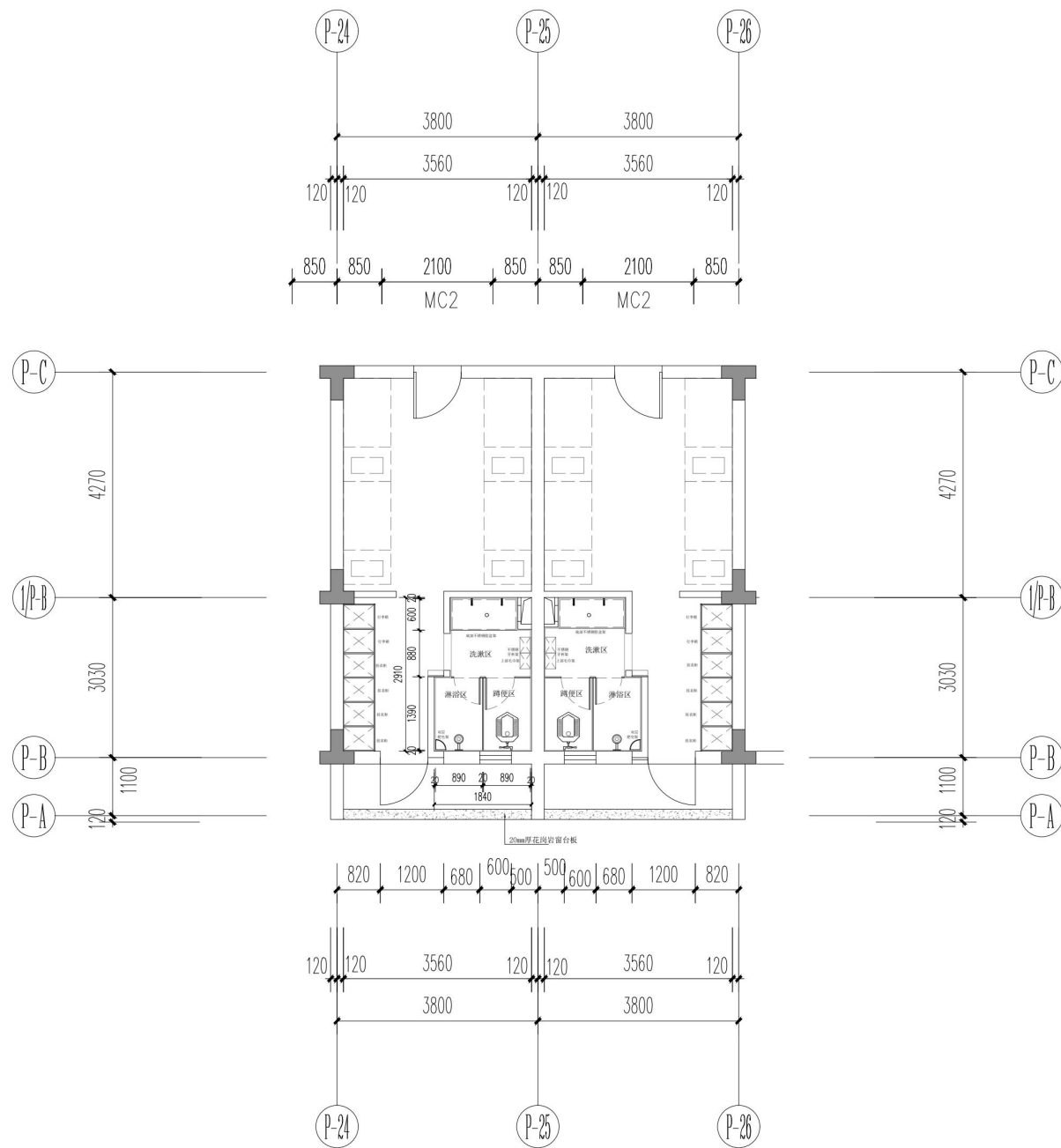
(4人间宿舍卫生间改造平面图)
