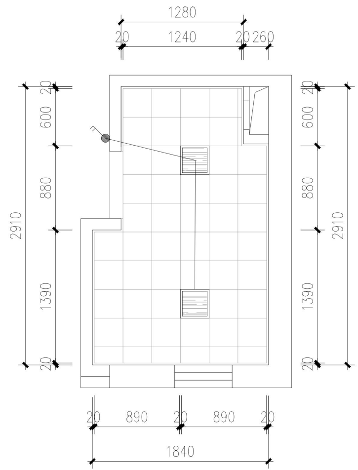
宿舍卫生间开关（2开控制）
