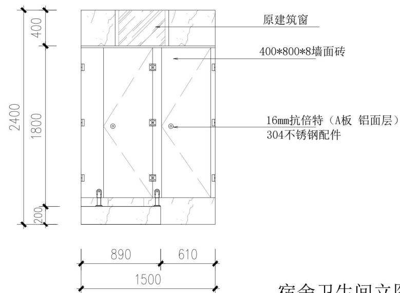
宿舍卫生间立图
