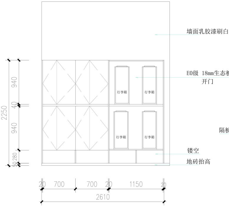
4人宿舍 衣柜立面图
