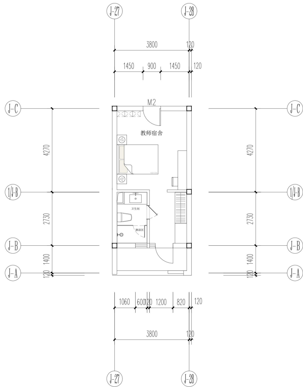
教师值班室房型 (2) 平面图
