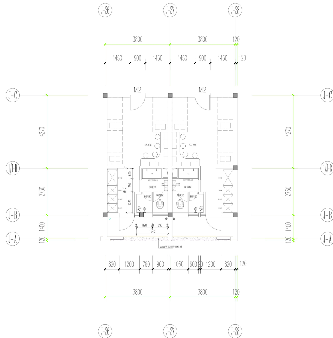
(6人间宿舍改造平面图)
