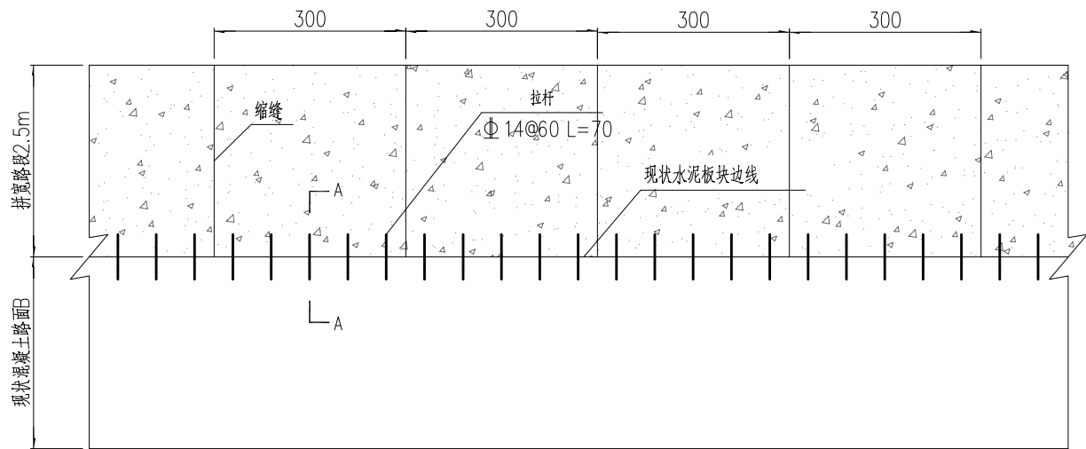
拼宽路面衔接平面图
