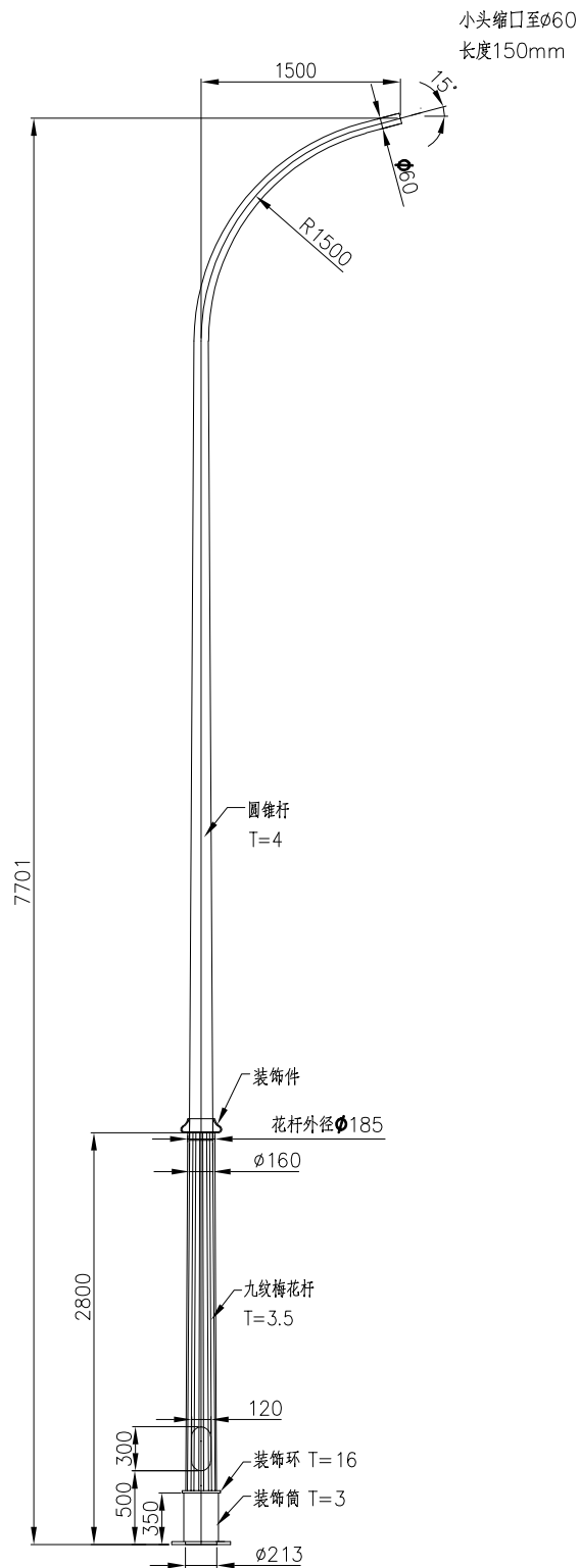
单挑路灯设计大样图
