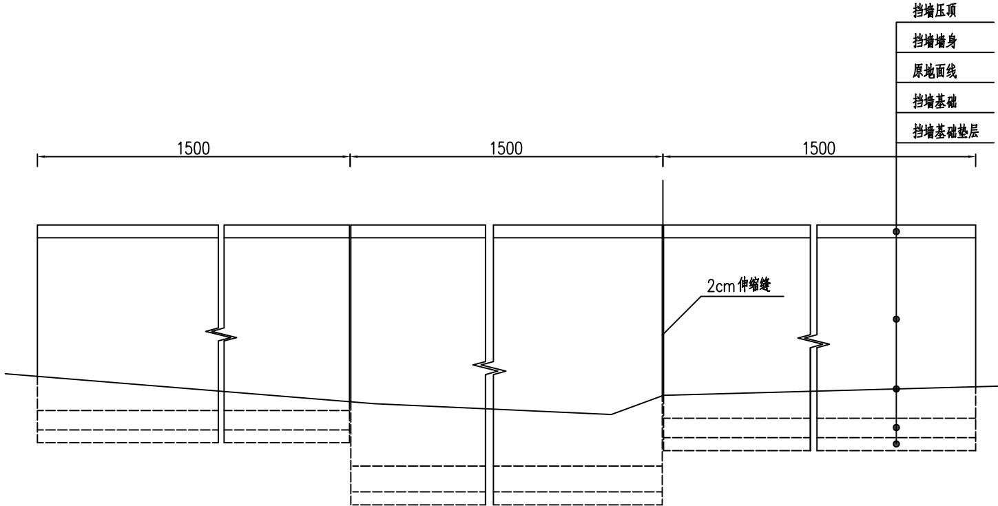
挡土墙立面示意图
