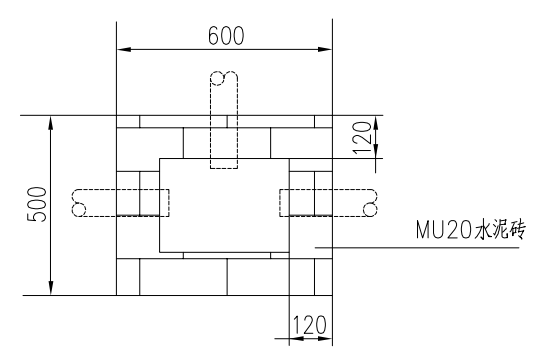
路灯检查井平面图
