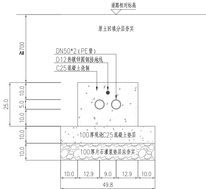
路灯电缆保护管敷设示意图 绿化带下
