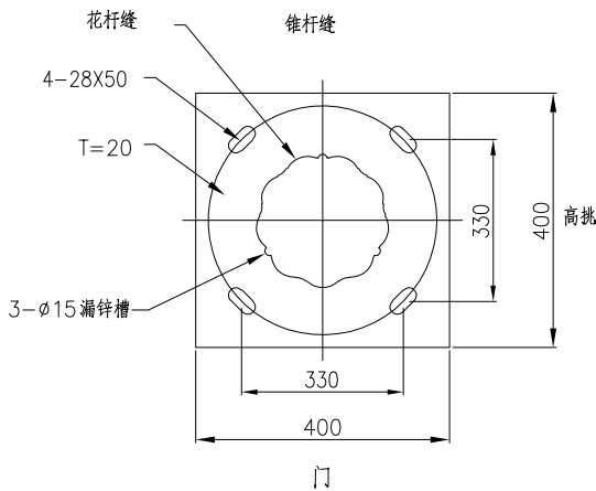
底法兰示意图
