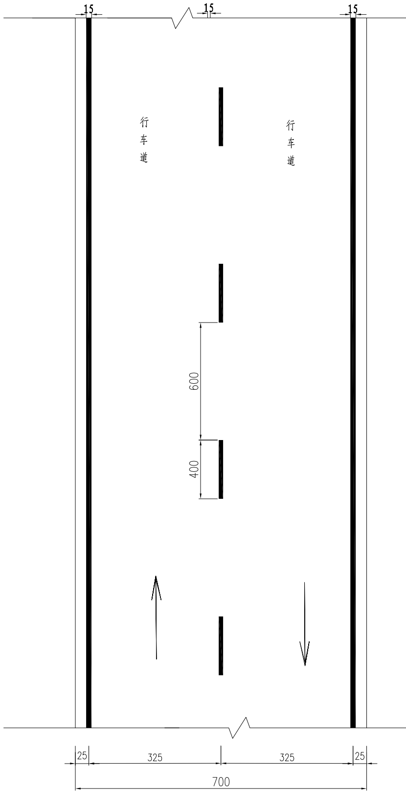
标准段标线布置图
