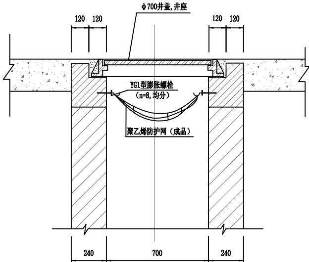
I-I 剖面图
