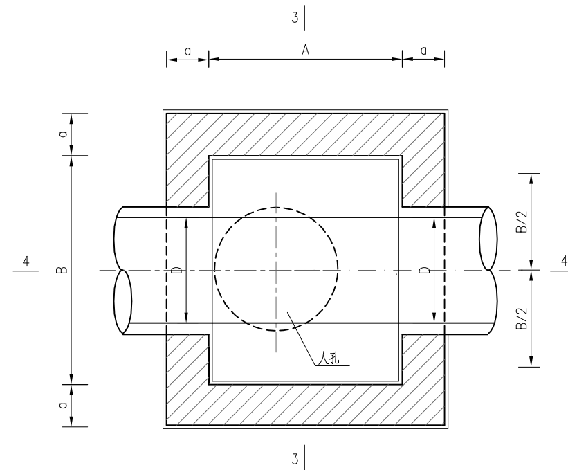
2--2 (井室平面)
