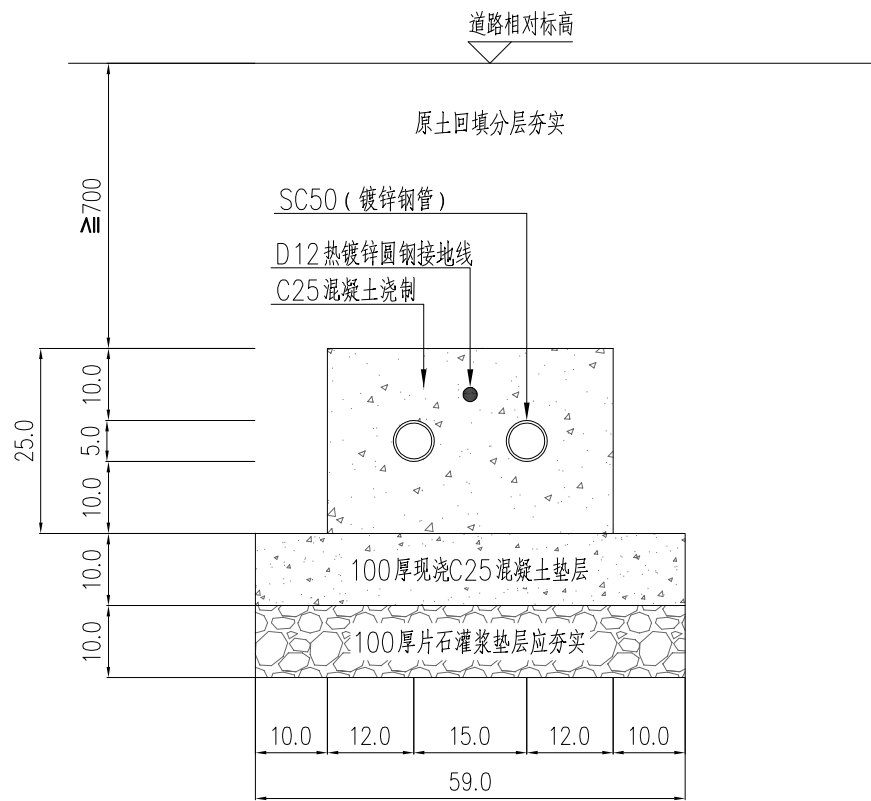
路灯电缆保护管敷设示意图 机动车道下
