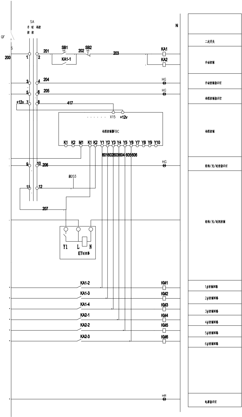
灯联网集中监控二次配电图
