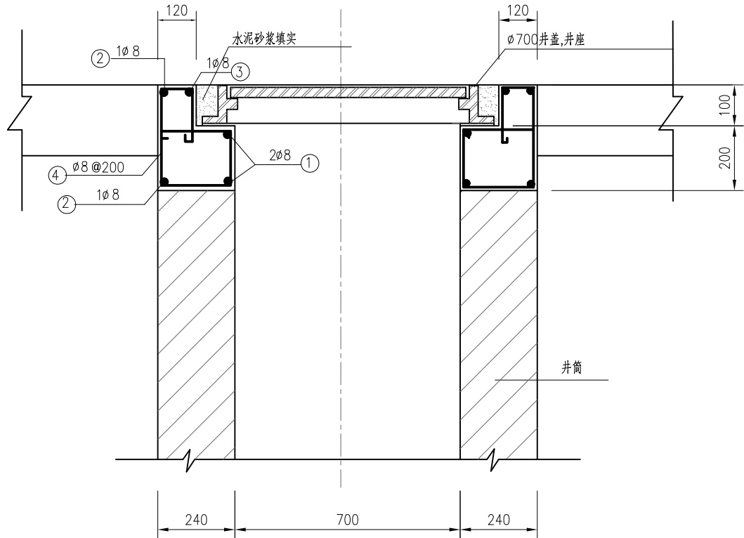
I—I 剖面图
