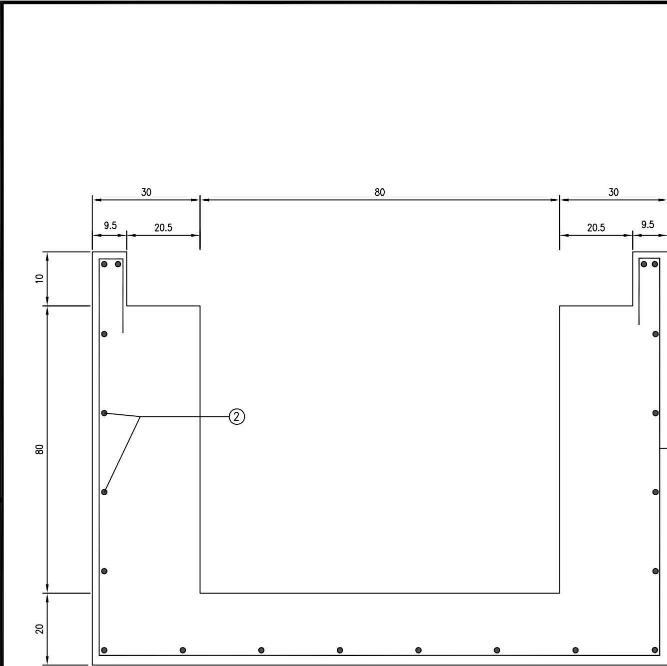
盖板沟配筋断面图
