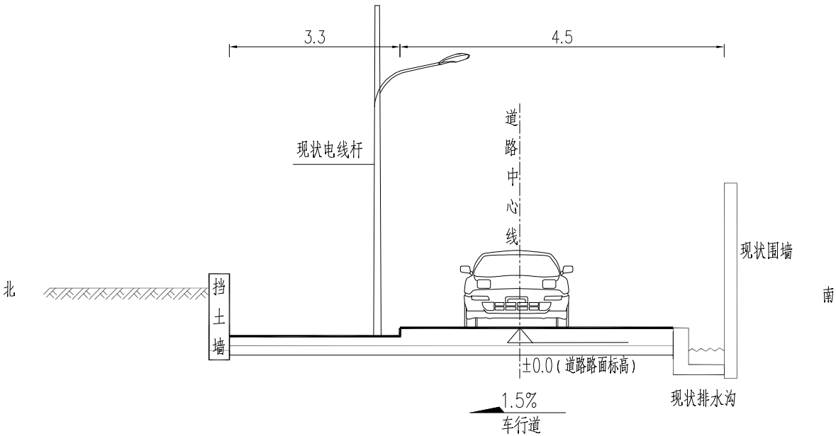
现状老路标准横断面设计图 K0+190-K0+290段
