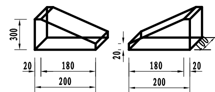
垫块大样图
