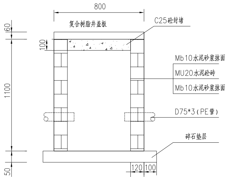
过街检修井剖面图
