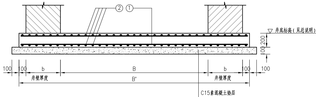
A-A剖面 1:30
