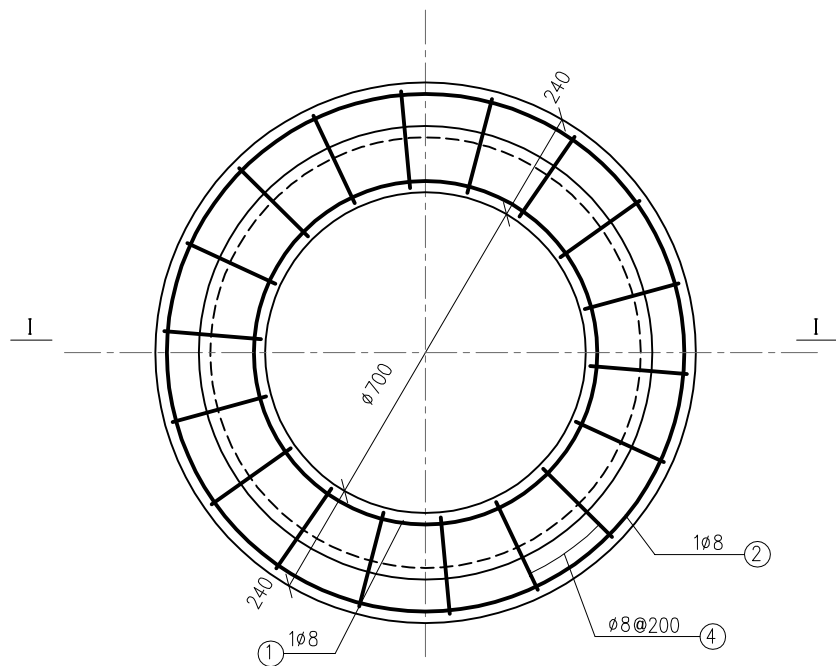
井座平面图
