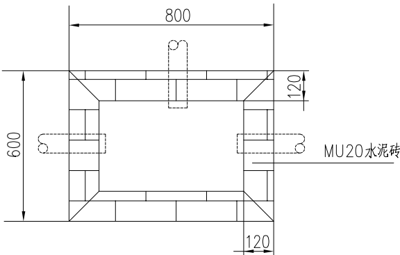
过街检修井平面图
