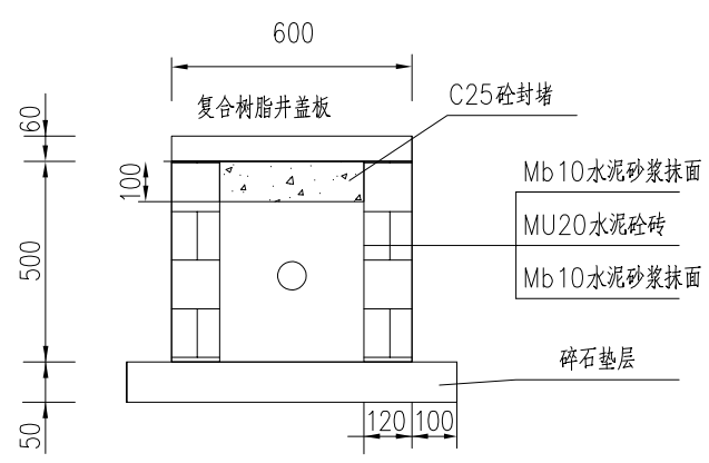
路灯检查井剖面图
