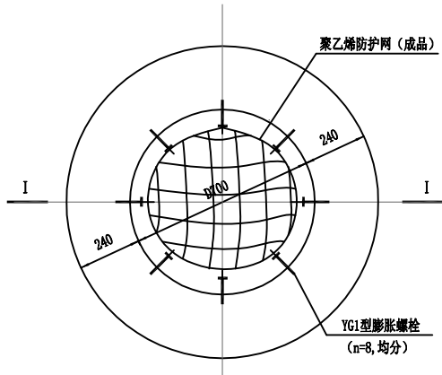
井座平面图
