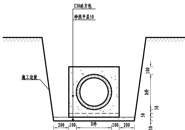
管道方包图
