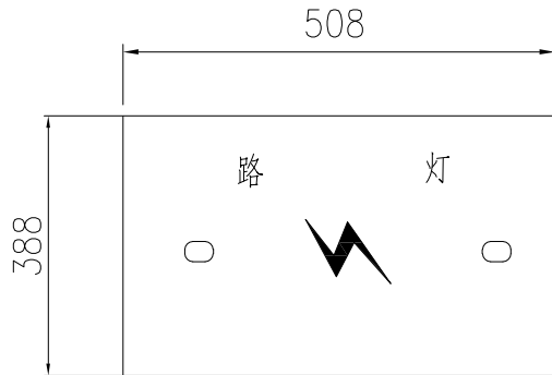
检修井盖板平面图
