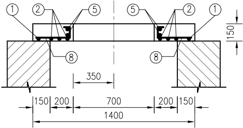
A—A剖面 1:30
