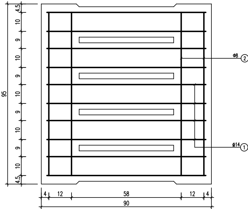
平面图
