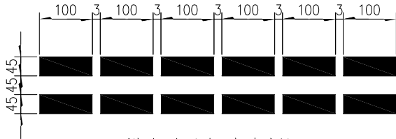
横向减速标线大样图
