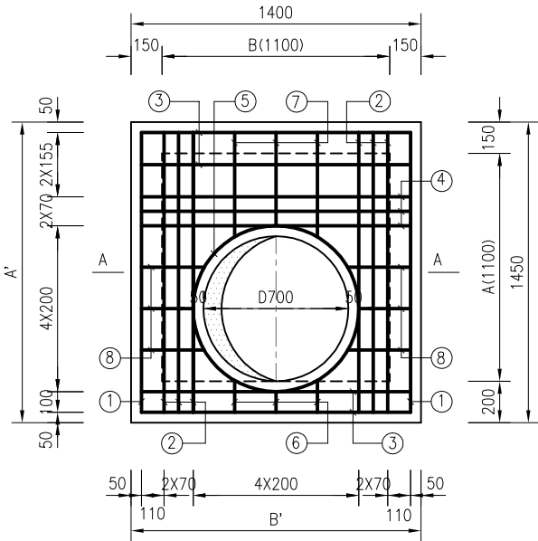
顶板配筋平面 1:30
