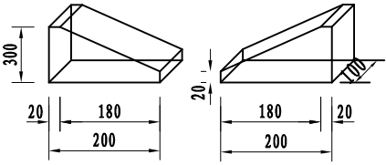
垫块大样图
