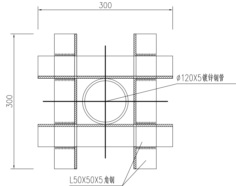
A-A 1:5
