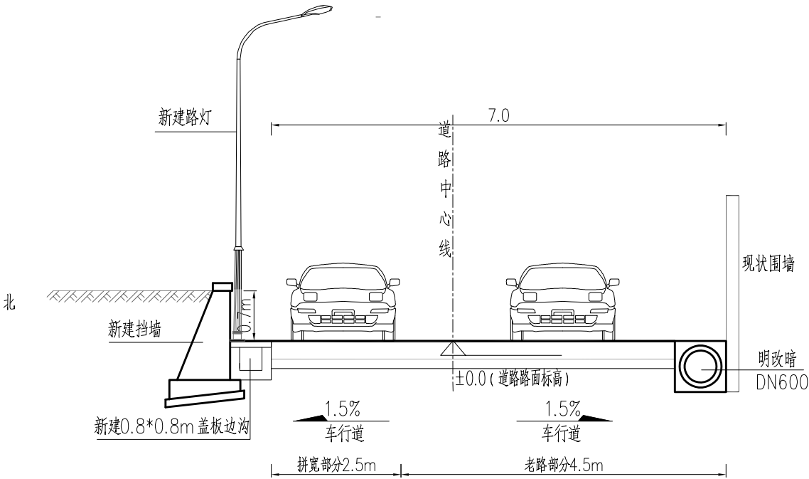
改造后标准横断面设计图 K0+190-K0+290段
