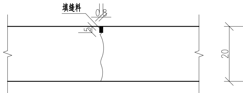
假缝型横向缩缝构造图
