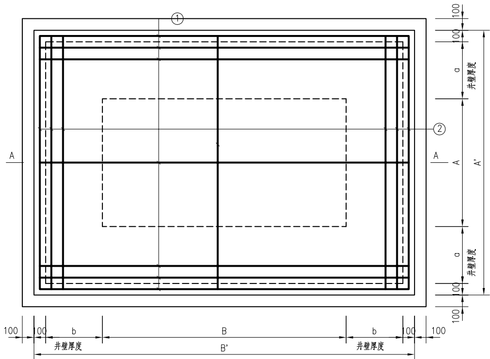
底板配筋平面 1:30
