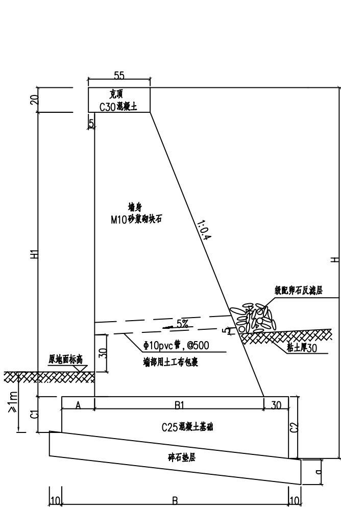
挡土墙结构图
