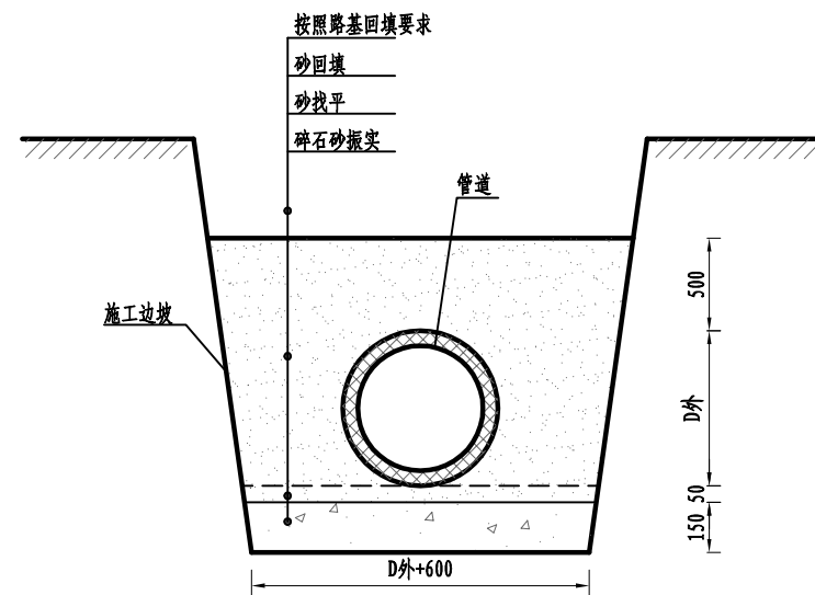
管道基础图
