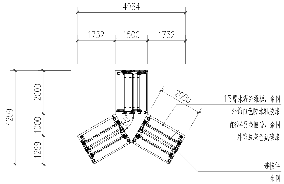
户外氛围装置(类型二)平面图
