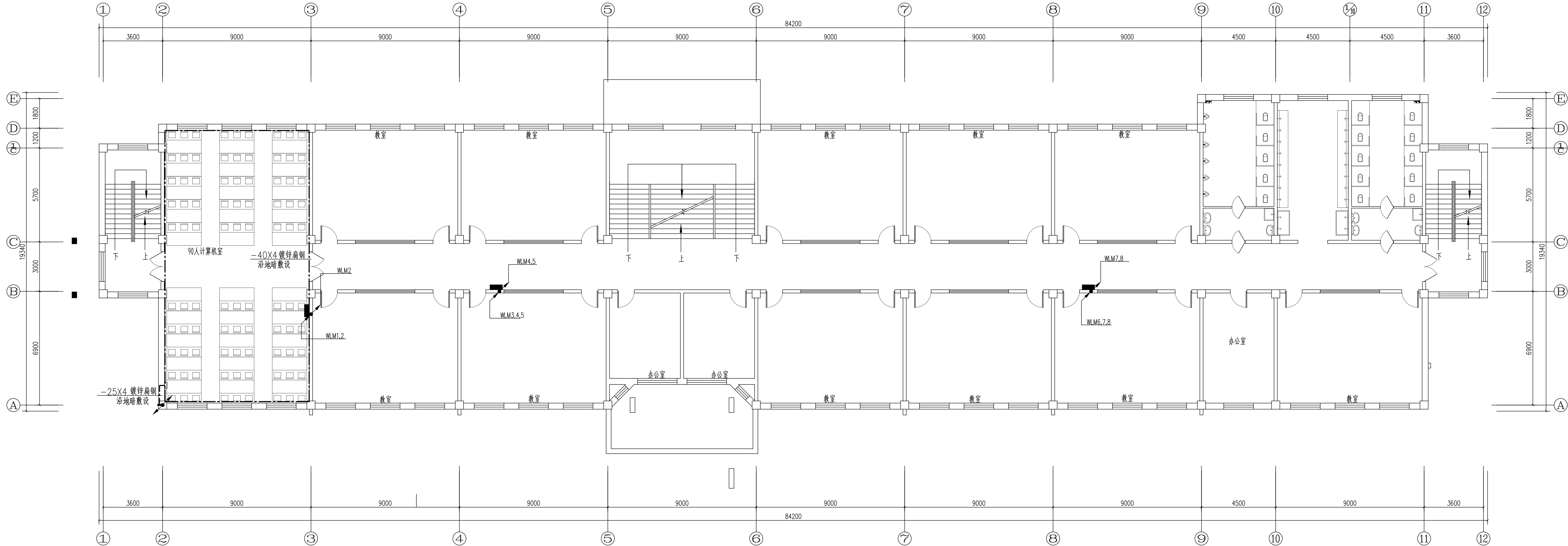
二层电气干线平面图 1:100
