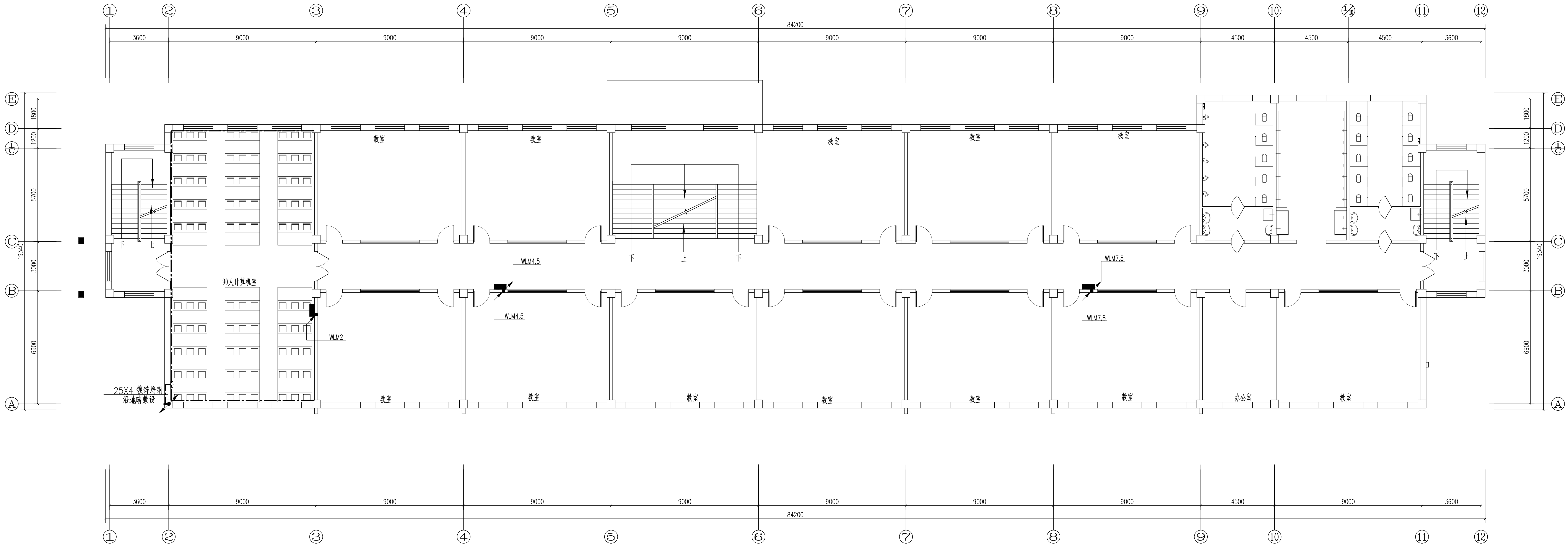
三层电气干线平面图 1:100
