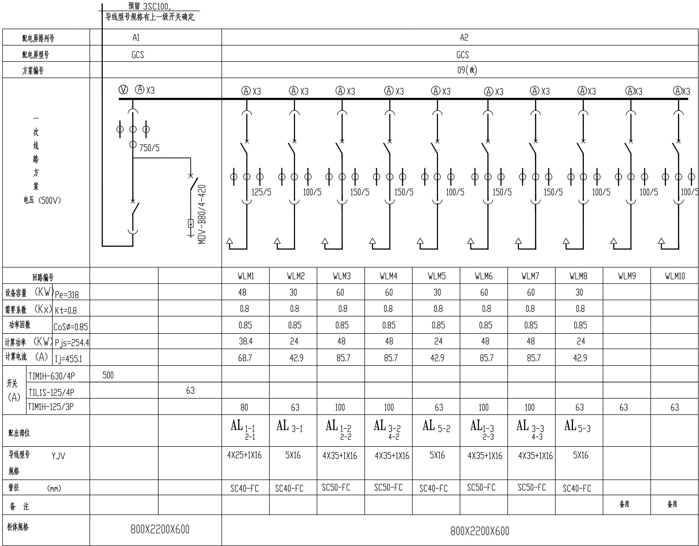
低压配电系统图
