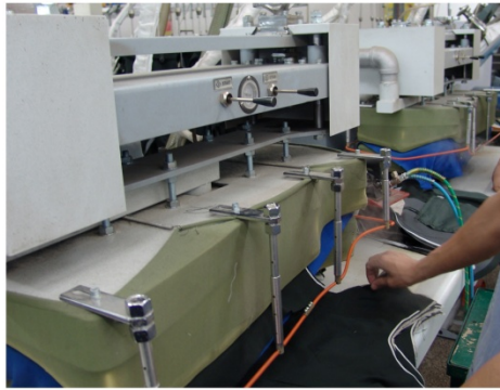
前门定型机
