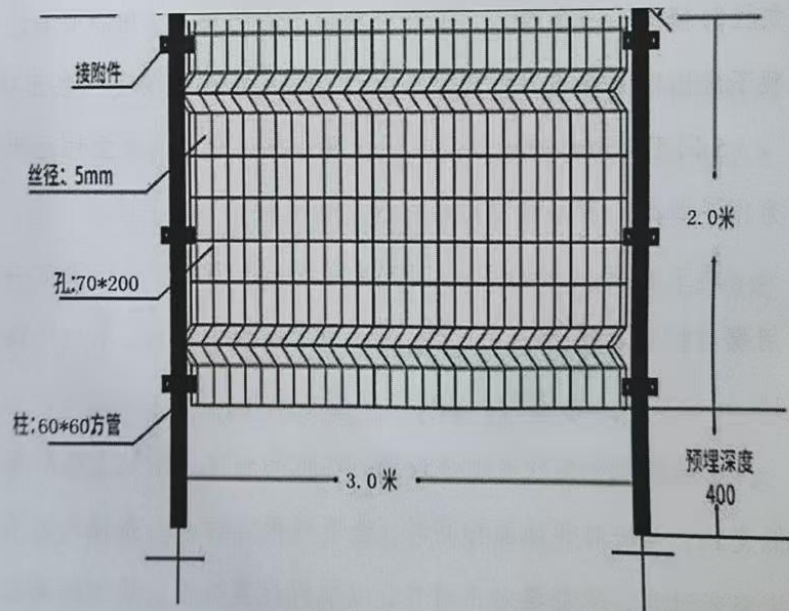
围栏安装示意图
