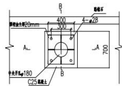
灯杆安装平面图
