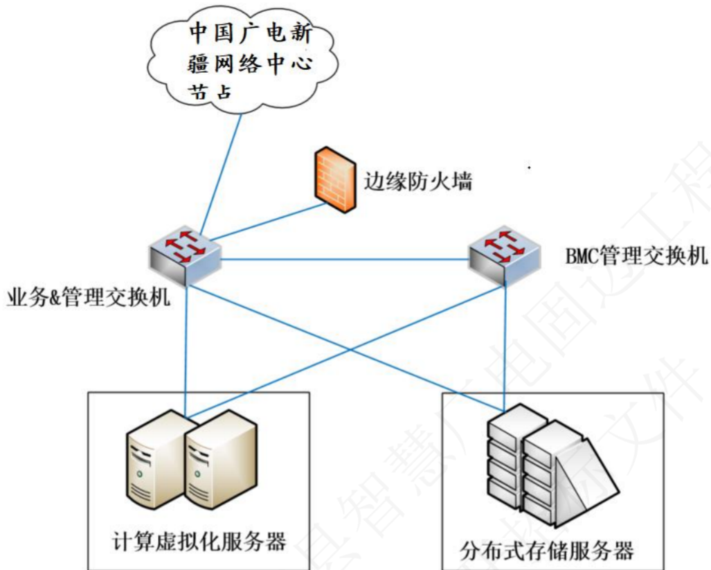
图 5-18 网络架构
