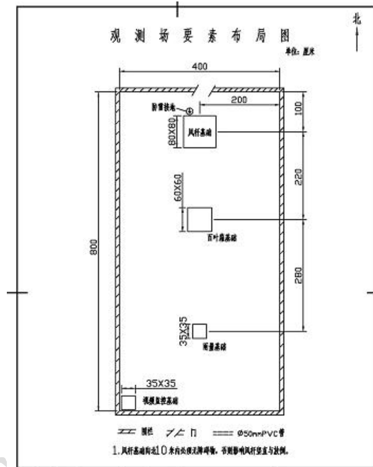
观测场布局图
